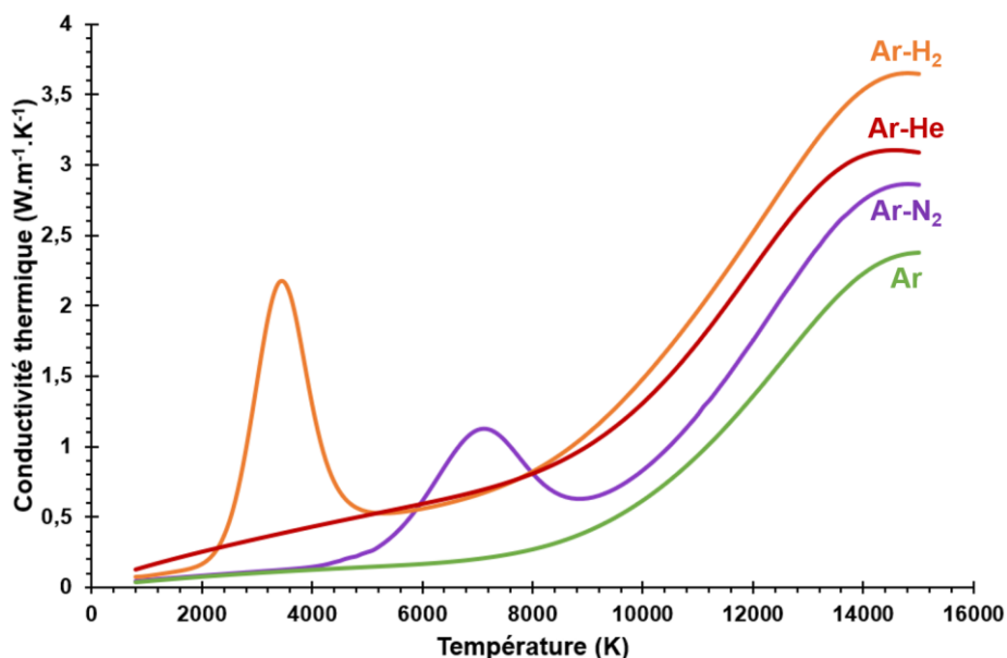
Figure III.11 : Évolution de la conductivité thermique avec la température pour les différentes compositions plasmagènes du Tableau III-1.
