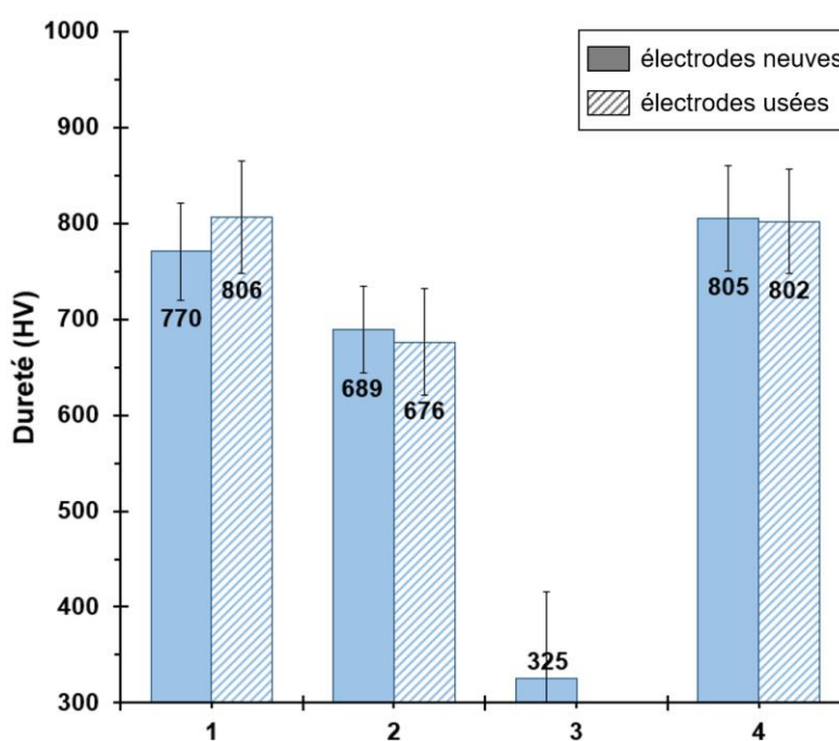
Figure V.13 : Microdureté des quatre conditions du Tableau V-10 pour des électrodes neuves et usées.
