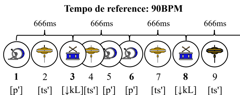
FIGURE 2.1 – Illustration de la structure métrique d'un Beat Pattern où le tempo de référence est 90BPM.
