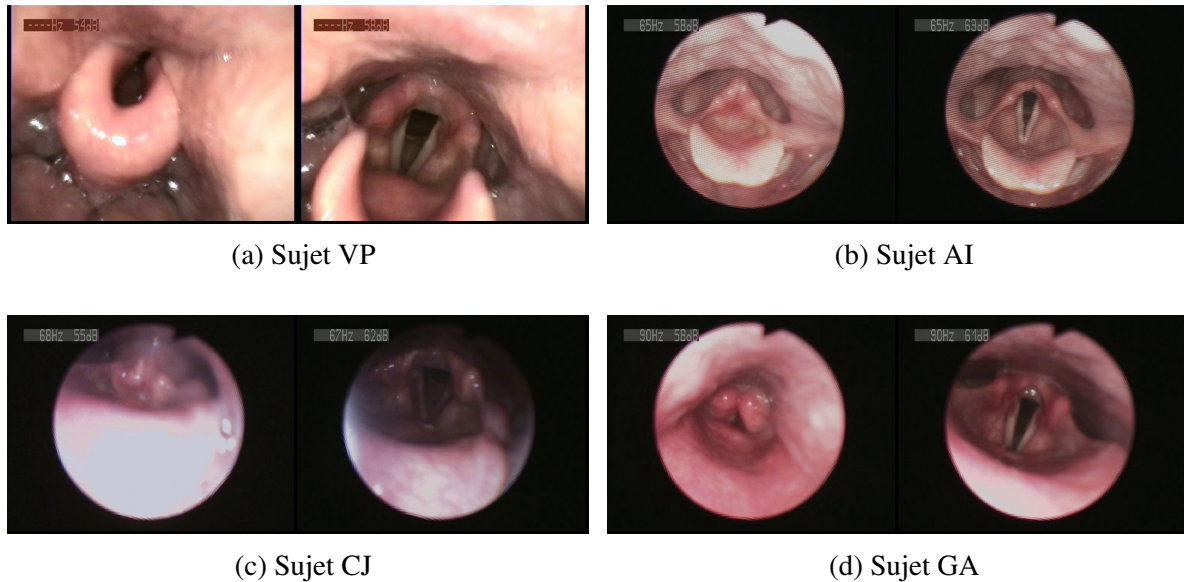
FIGURE 3.19 – Configuration laryngale pendant l'occlusion et le relâchement de [ʔ̥].
