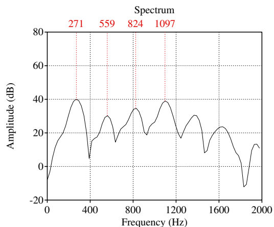
(c) Spectre FFT à 2kHz
