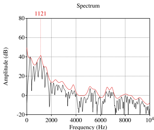
(b) Spectre FFT (noir) et LPC 12 coefficients (rouge) du bruit de friction
