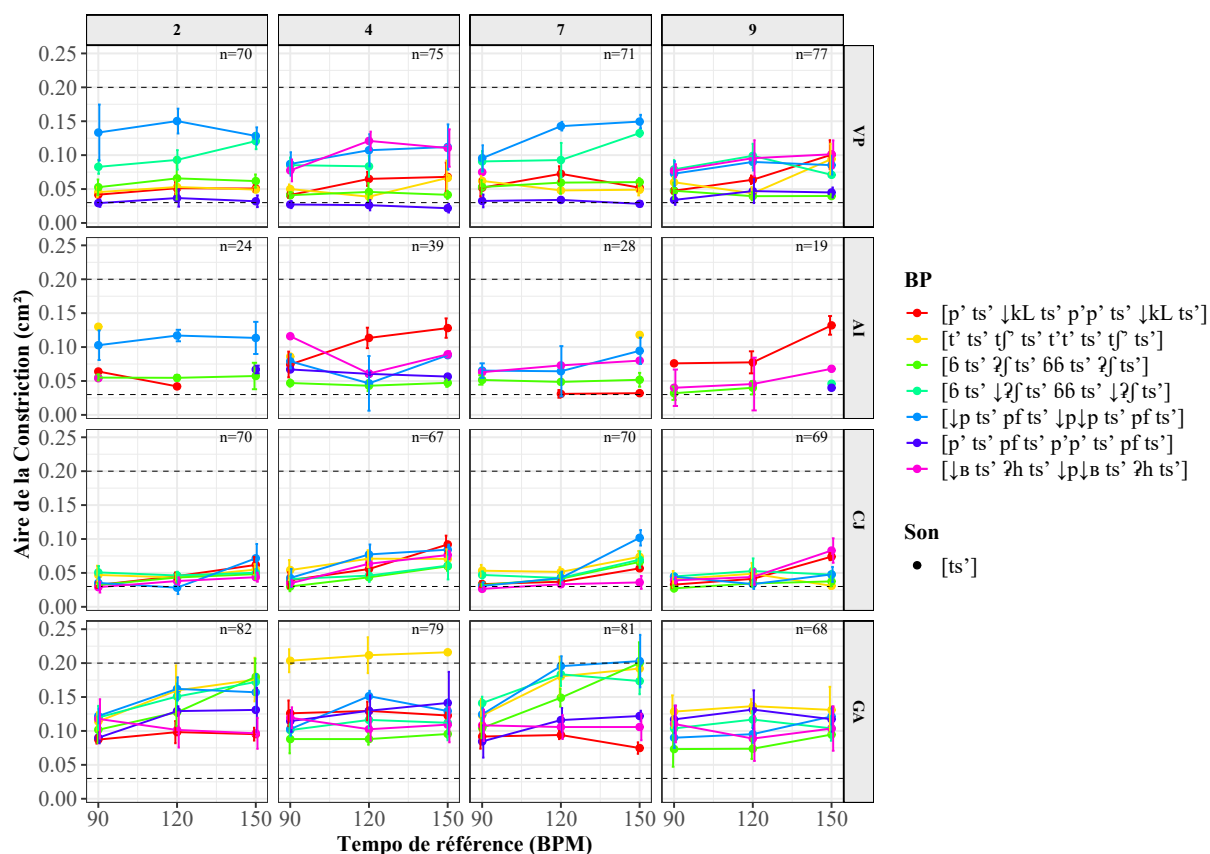
FIGURE 4.20 – Aire relative de constriction ( cm^2 ) en fonction du tempo de référence (BPM) pour le son [\widehat{ts}] dans différents BP et différentes positions. Les pointillés à 0.03cm^2 indiquent le seuil en-dessous duquel l'intensité de la turbulence est réduite. Les pointillés à 0.2cm^2 indiquent le seuil au dessus duquel l'intensité de la turbulence est réduite.
