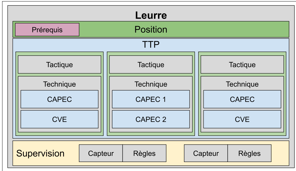
Figure 3.3: Différents composants possibles de notre modèle de leurre détaillés. Le leurre est défini par une position, un ensemble de couples (Tactique, technique) groupés sous appellation TTP ainsi que plusieurs éléments de supervision couvrant la Supervision Générale et la Supervision Ciblée.
