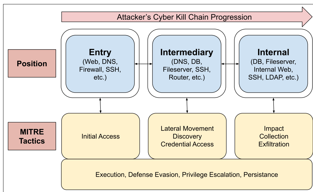
Figure 3.2: Schéma des parallèles entre la progression spatiale des attaquants et leur avancée dans la CKC. Les leurres peuvent appartenir à trois positions en fonction de leur accessibilité depuis l'extérieur du réseau de leurres. Ces positions reflètent l'organisation réelle des réseaux et la progression des attaquants sur la CKC. Cet exemple de progression est implémenté dans notre première expérience.
