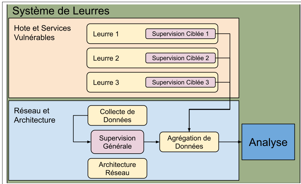
Figure 4.1: Niveaux d’architecture de notre implémentation de leurres. La Supervision Générale est intégrée au niveau “Network and Architecture”, avec ses composantes et ses contraintes, notamment concernant l’agrégation des données pour l’analyse. A l’opposé, la configuration des leurres liée à leur Supervision Ciblée appartient au niveau “Hosts and Vulnerable Services”.
