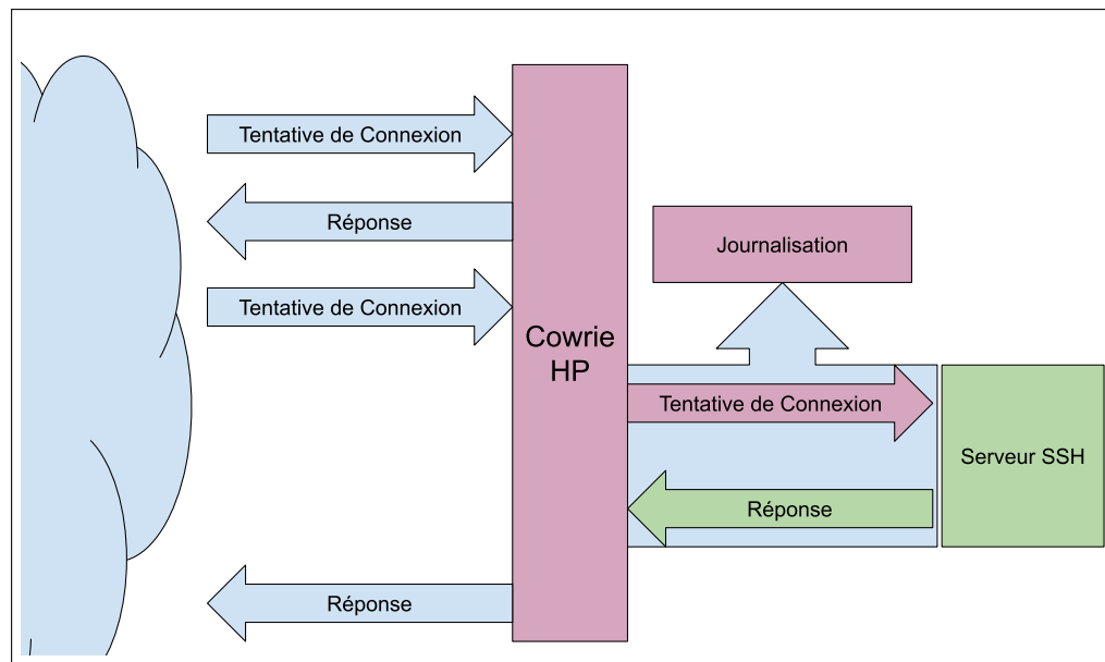
Figure 4.5: Description schématique du fonctionnement de Cowrie. Le proxy gère la phase d’authentification en journalisant les données entrées par le client. Une fois l’utilisateur authentifié, le proxy journalise puis transmet les commandes au serveur intégrant le démon ssh et renvoie à l’attaquant les réponses.
