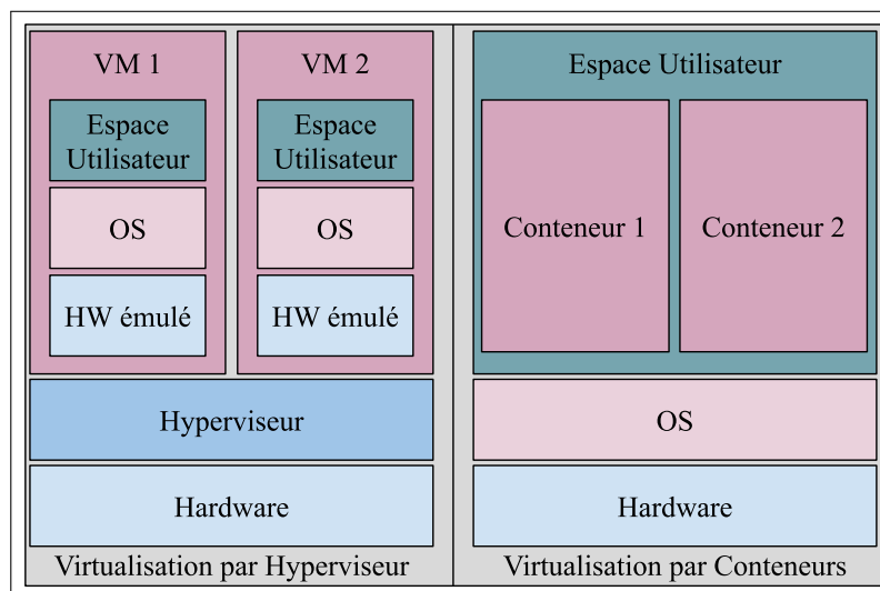
Figure 2.4: Schéma des architectures de virtualisation basées sur les hyperviseurs et sur les conteneurs, inspiré de Eder [24]. On remarque que les conteneurs n'émulent pas de hardware et n'intègrent pas leur propre système d'exploitation, allégeant conséquemment la virtualisation.
