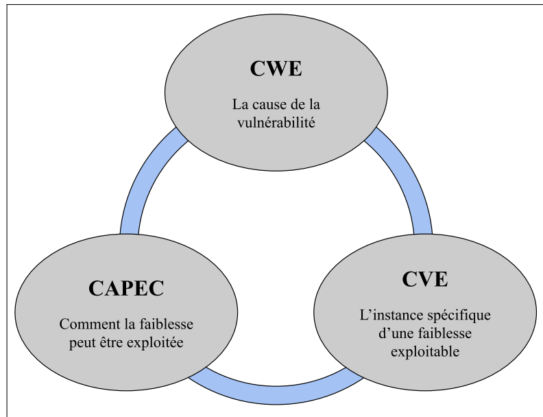
Figure 2.6: Lien entre les CAPEC, les CVE et les CWE, d'après le site web décrivant les CAPEC[52]
