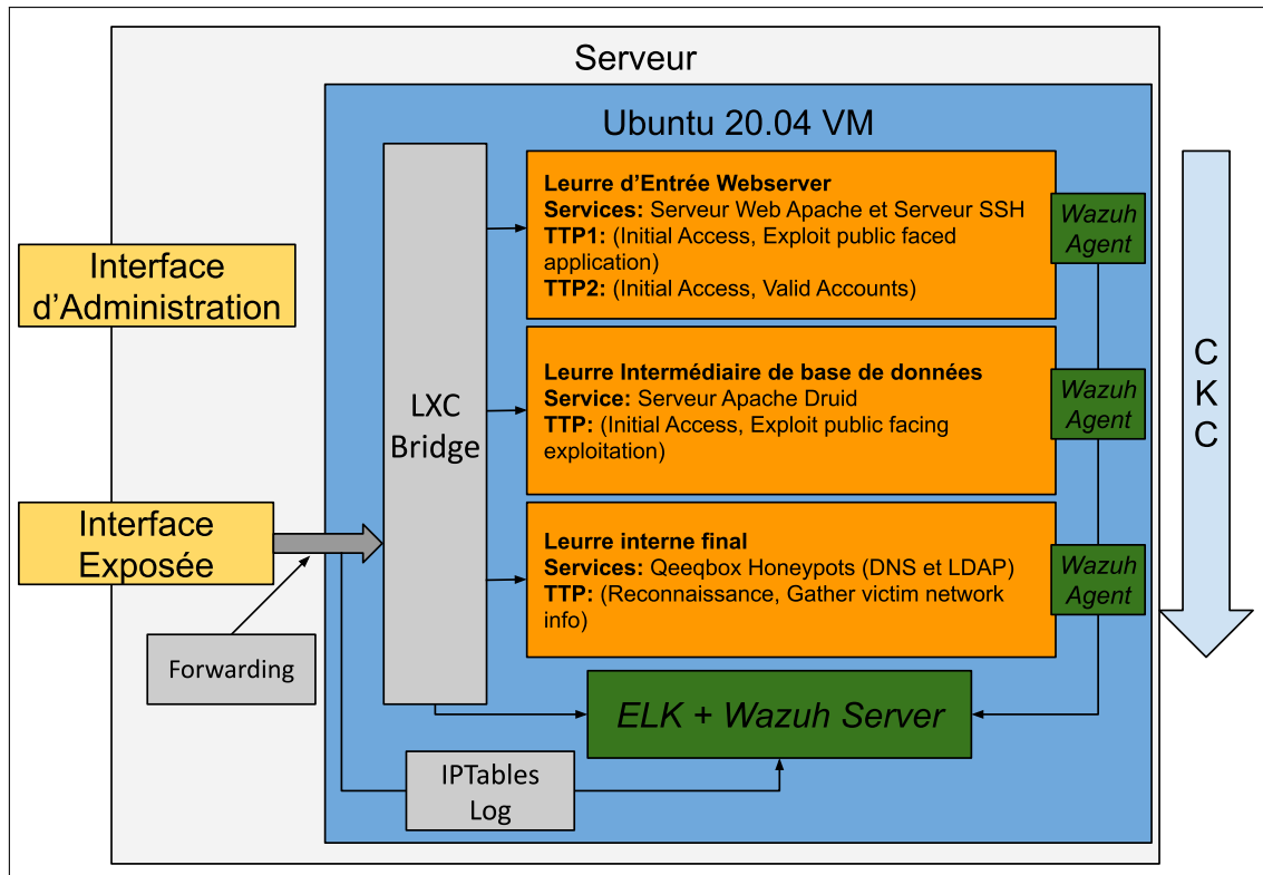
Figure 4.2: Schéma de notre implémentation. En jaune, les deux interfaces permettent de connecter le réseau de leurres à l'extérieur. En Orange, on représente les trois leurres sous la forme de conteneurs LXC. En gris, on retrouve les éléments de réseau qui permettent le fonctionnement de notre implémentation. En vert, on représente les éléments des supervisions générales et spécifiques. On représente aussi sur le schéma le sens de progression des attaquants.
