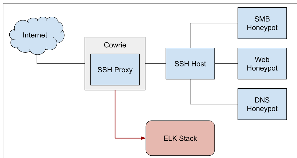
Figure 4.3: Architecture générale de la seconde implémentation du système de leures. Nous avons conservé de la première implémentation le service web, le serveur DNS simulé ainsi que la pile ELK pour l'agrégation des données. Nous avons ajouté un nouveau leurre SSH ainsi qu'un leurre SMB simulé.
