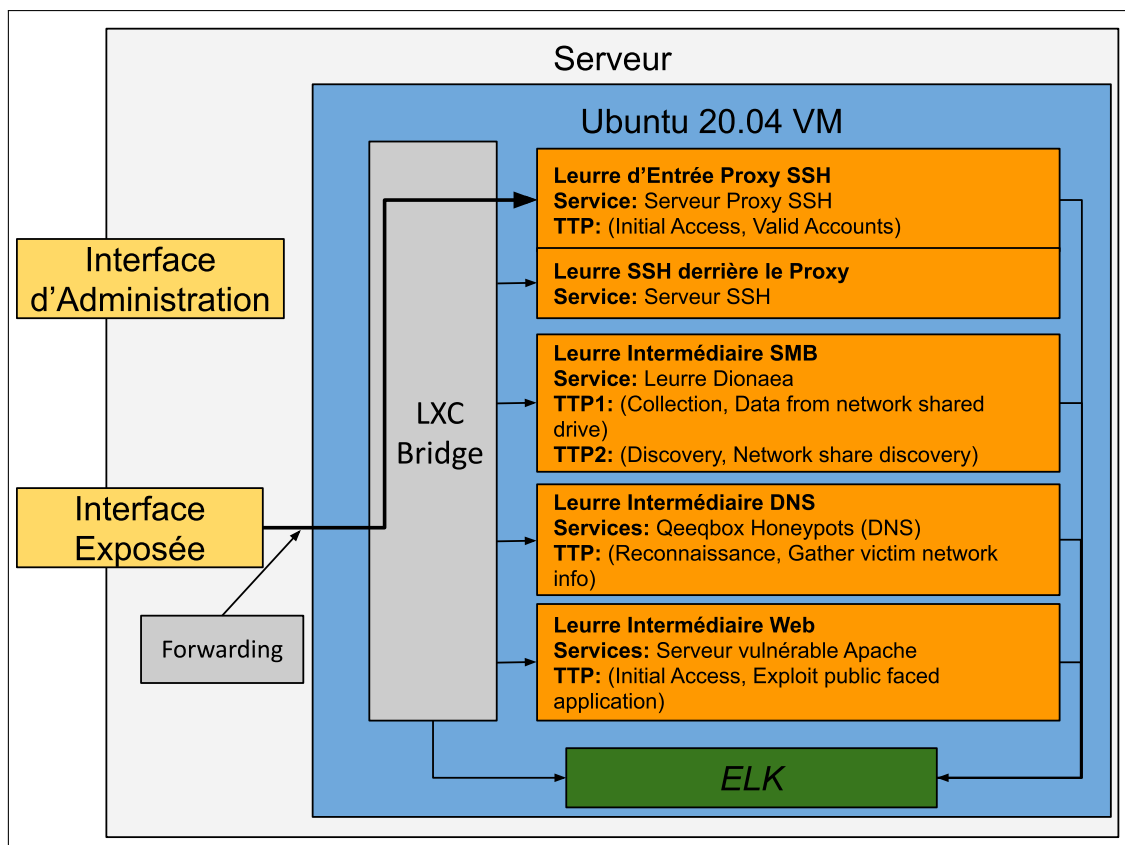
Figure 4.4: Schéma de notre implémentation. En jaune, les deux interface permettent de connecter le réseau de leures à l'extérieur. En Orange, on représente les leures sous la forme de conteneurs LXC. En gris, on retrouve les éléments de réseau qui permettent le fonctionnement de notre implémentation. En vert, on représente les éléments de supervision, en particulier la pile ELK qui permet la centralisation des données.
