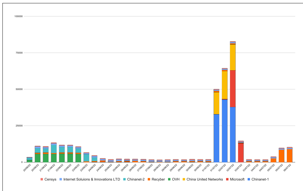
Figure 5.2: Distribution du nombre d'événements par demi-journée liés aux 8 acteurs les plus actifs uniquement. On remarque que certains sont actifs tout au long ou presque de la durée de l'expérience, tandis que d'autres focalisent leurs attaques sur un ou deux jours, avec un très haut volume journalier.
