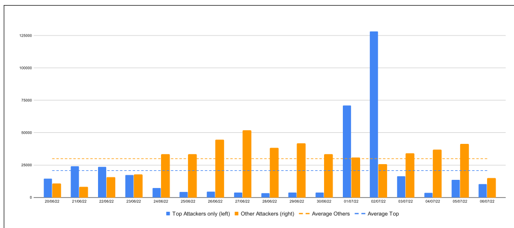
Figure 5.1: Distribution comparée du nombre d'événements par jour liés aux 8 acteurs les plus actifs (Top) et aux autres sources (Other). On remarque que les pics les plus élevés d'activité sont du fait des acteurs les plus actifs, et qu'ils représentent souvent une partie importante du trafic journalier.
