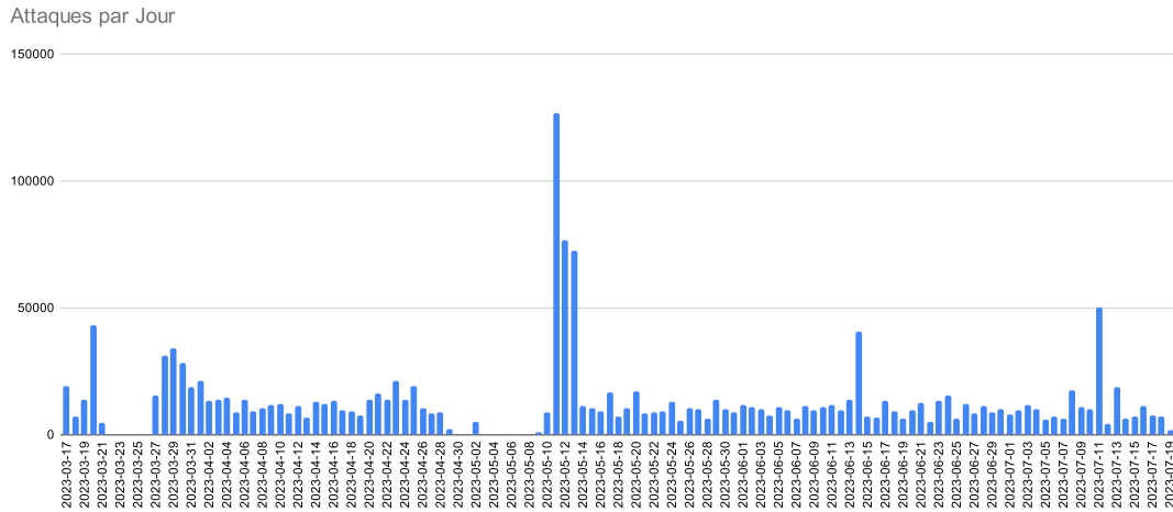
Figure 5.6: Analyse temporelle du nombre d'attaques par jour. On remarque pour la seconde partie de notre expérience, entre mai et juillet, une distribution très lisse des attaques, avec deux pics d'une journée.
