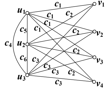
(6) G^6_{3,1}
