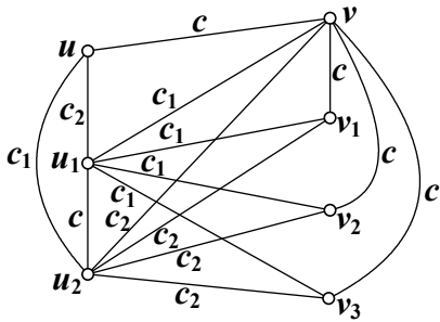
(3) G^3_{2,1}
