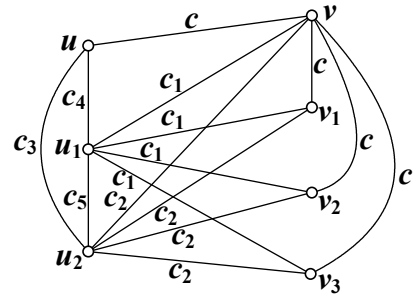
(4) G^4_{2,1}
