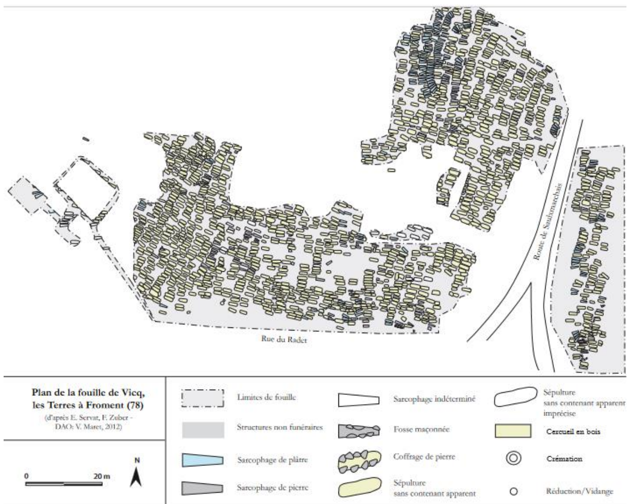
Figure 15 -Espace densément occupé de la nécropole de Vicq "le radet, les terres à froment" (DAO Maret, 2012 in Le Forestier, 2016)
