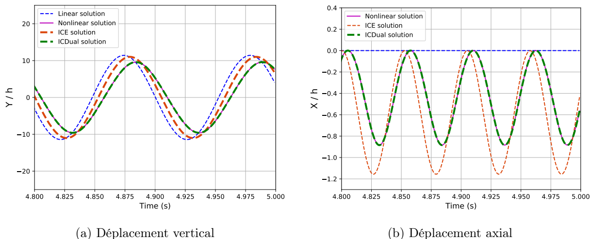
Figure 6.6: Déplacement non-linéaire dynamique à l'extrémité de la poutre de Bernoulli/von Kármán encastree-libre en rotation à 500 tr/min soumise à un chargement suiveur sinusoïdal en bout de poutre d'amplitude 7,350 N et de fréquence correspondant à celle du premier mode en rotation. Comparaison des résultats des différents modèles.
