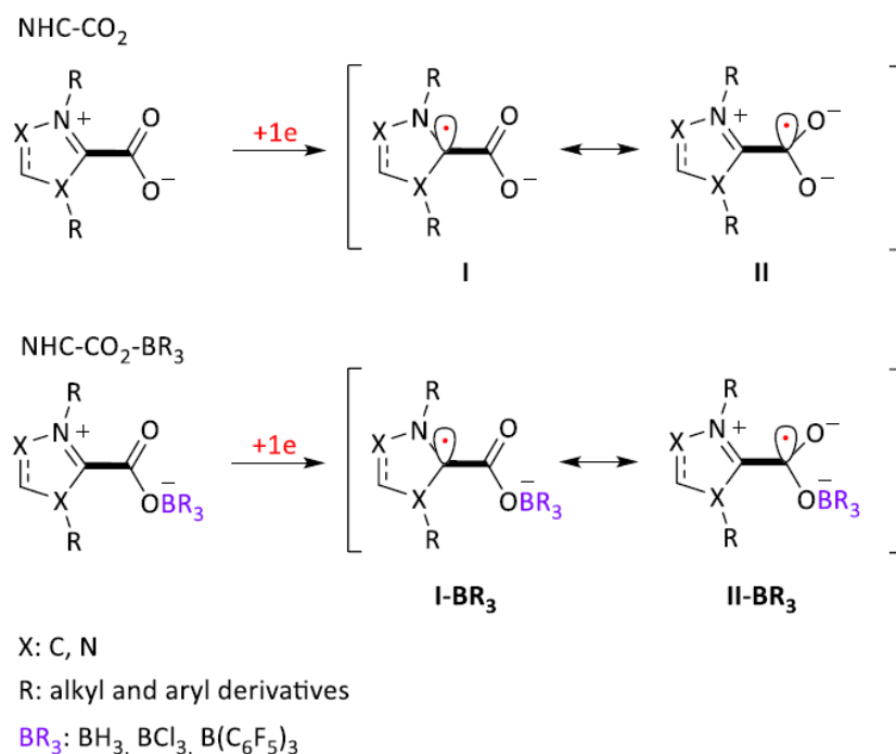
Schéma 10. Structures résonantes dans la forme réduite d'adduits NHC-CO 2 et NHC-CO 2 -BR 3 .
