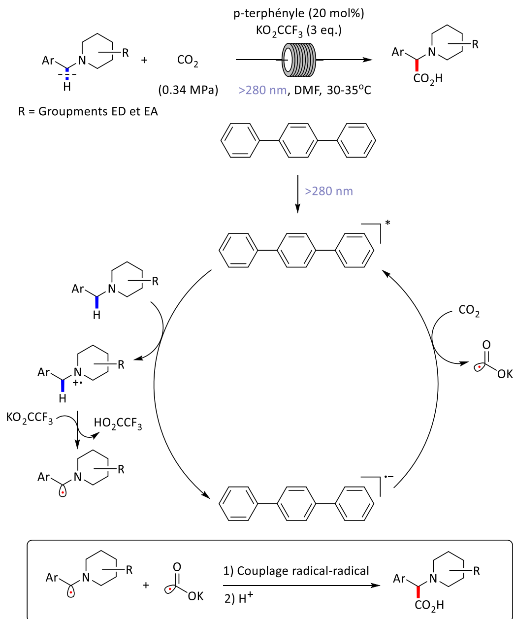
Schéma 2. Activation photorédox du dioxyde de carbone pour la synthèse d'acides aminés en flux continu par le groupe de Jamison.
