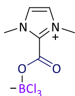
(1-BCl 3 )
