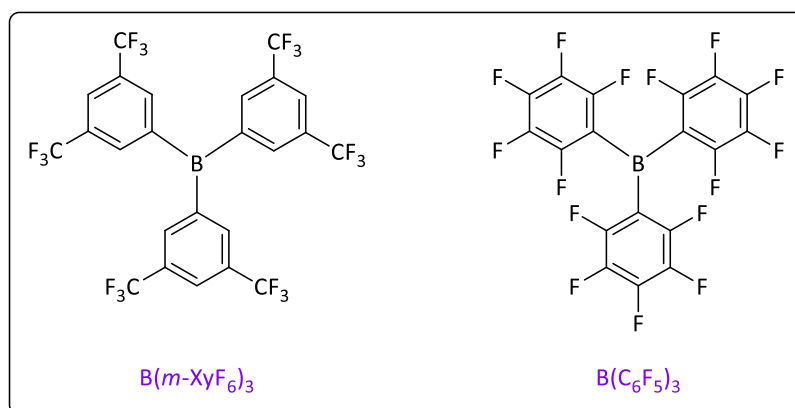
Schéma 5. Synthèse des adduits NHC-CO 2 -BR 3 .
