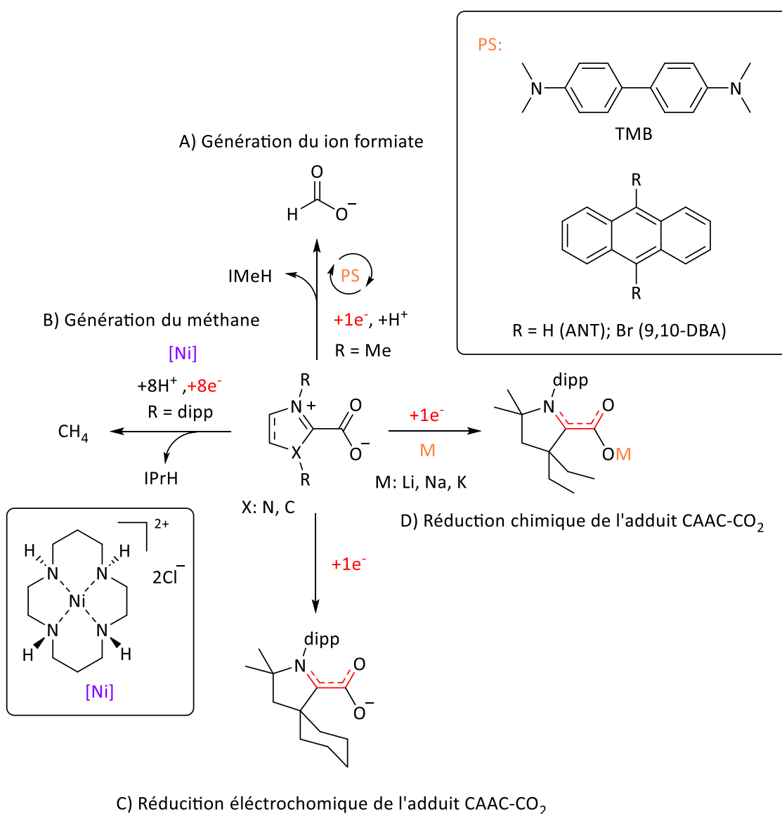
Schéma 4. Réduction des adduits NHC-CO 2 . A) Génération de l'ion formiate. B) Génération du méthane. C) Réduction électrochimique de l'adduit CAAC-CO 2 . D) Réduction chimique de l'adduit CAAC-CO 2 .
