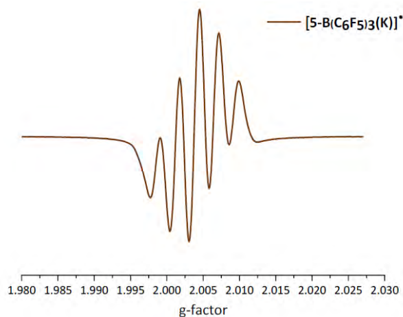
Figure 3. Spectre de RPE en bande X à régime continu de [5-B(C_6F_5)_3(K)]^* pris dans une solution de THF à température ambiante.
