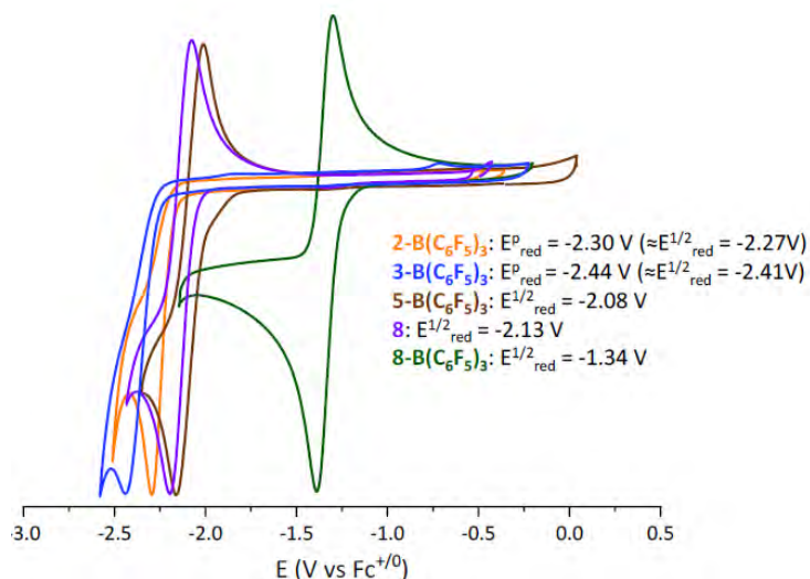
Figure 1. Détermination par voltampérométrie des potentiels de réduction des adduits 2-, 3-, 5-, 8-B(C 6 F 5 ) 3 dans le CH 2 Cl 2 par rapport à Fc +/0 .
