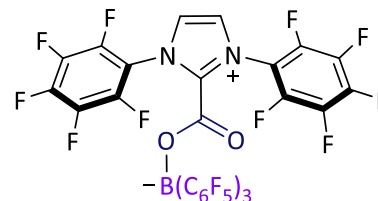
(6-B(C 6 F 5 ) 3 )
