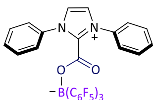
(4-B(C 6 F 5 ) 3 )
