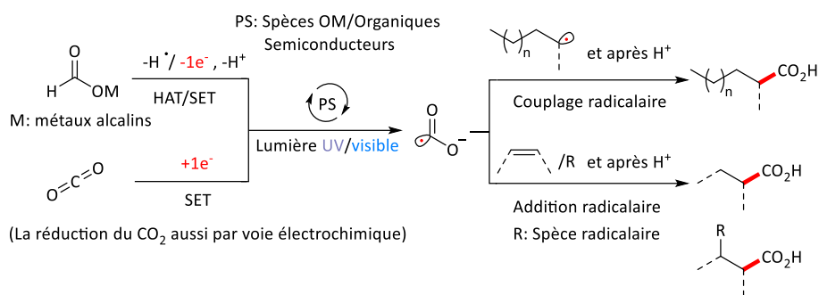
Schéma 1. Génération de l'anion radical [CO 2 ] •- et son utilisation dans la formation de liaisons C-C.
