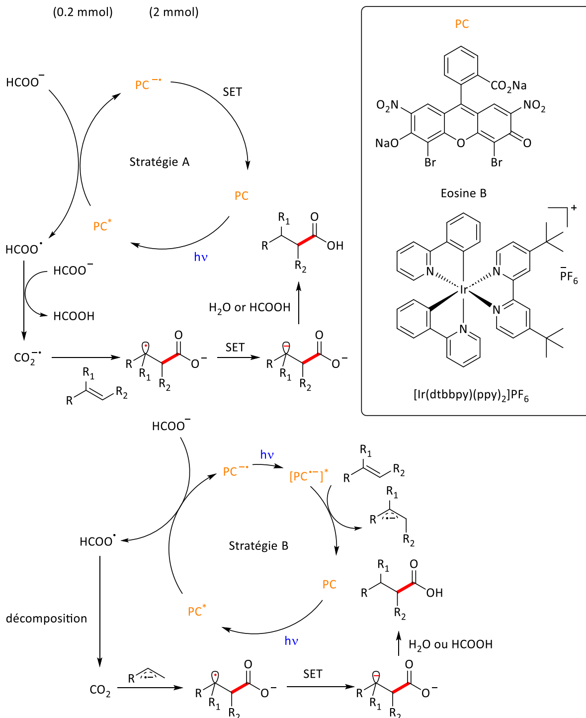
Schéma 3. Hydrocarboxylation des dérivés d'alcènes avec des sels de formiate catalysée par un photocatalyseur organique ou organometallique à base d'iridium.
