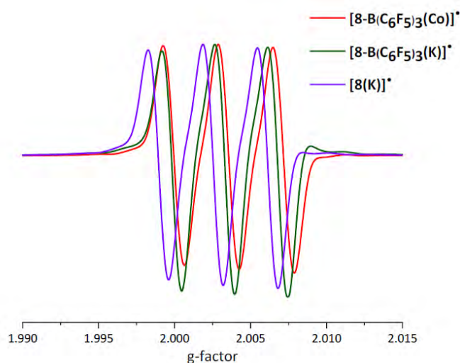
Figure 2. Spectres de RPE en bande X à régime continu de [8(K)]^* et [8-B(C_6F_5)_3(K)]^* pris dans une solution de THF, ainsi que [8-B(C_6F_5)_3(Co)]^* dans une solution à 3,7 mM de CH_2Cl_2 à température ambiante.
