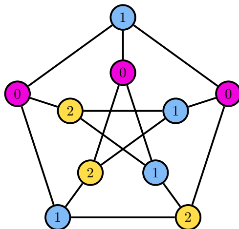
Figure 6: Une 3-coloration du graphe de Petersen
