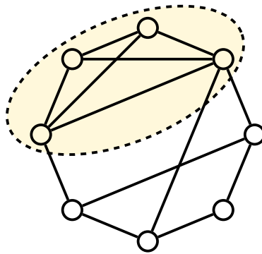
Figure 7: Un graphe contenant une clique de taille 4
