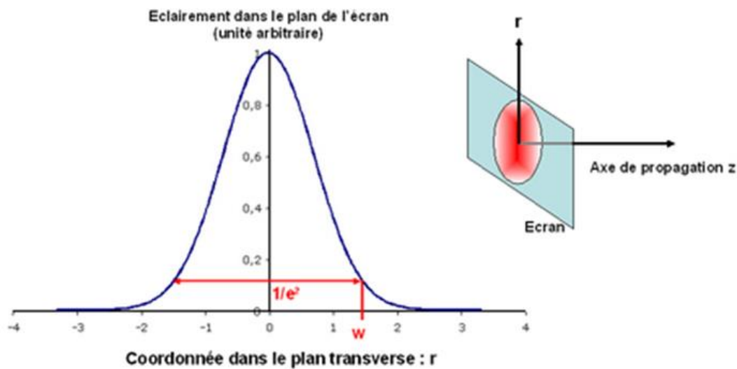
Figure 0.8. Allure d'une onde gaussienne : répartition de l'éclairement d'un faisceau laser dans un plan perpendiculaire à la direction de propagation ( http://www.optique-ingenieur.org/fr/cours ).
