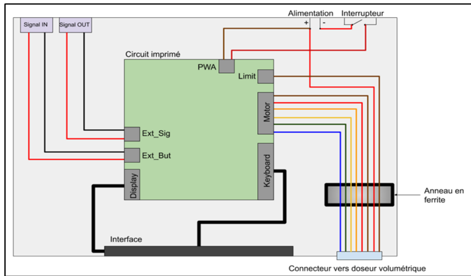
Figure 1.26. Schématisation du fonctionnement et du câblage du boîtier de contrôle du doseur volumétrique Precifluid®.
