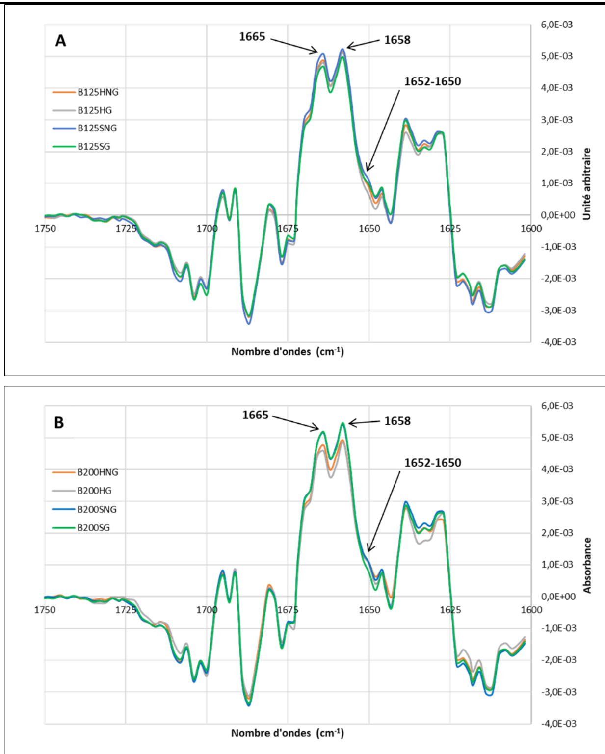
Figure 2.32. Représentation des courbes moyennes obtenues à partir de 3 répétitions pour la bande spectrale attribuée à l'Amide I, après dérivée seconde des spectres. (–) condition Humide/Non-Glyquée (HNG) ; (–) condition Humide/Glyquée (HG) ; (–) condition Sèche/Non-Glyquée (SNG) ; (–) condition Sèche/Glyquée (SG). A – Gélatine d'indice Bloom 125 ; B – Gélatine d'indice Bloom 200. Les nombres d'onde indiqués sont associés à des vibrations de la bande Amide I (étirement de la liaison C=O) (Movasaghi et al., 2008).
