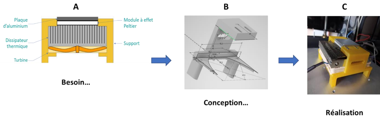
Figure 1.19. Détails du système de plateau d'impression refroidi, spécialement conçu pour le second prototype d'imprimante 3D alimentaire développée au laboratoire. A – Vue en coupe du module de plateau d'impression refroidi ; B – Vue du plan de conception et, C – Vue du dispositif fixé sur le plateau de l'imprimante.
