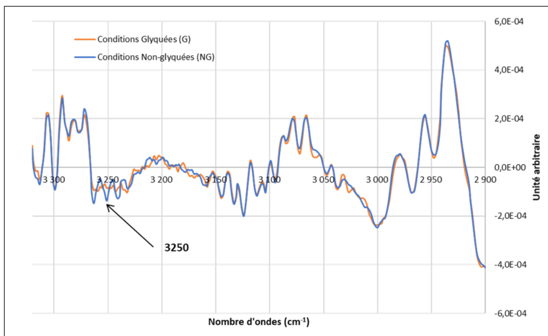
Figure 2.28. Représentation des courbes moyennes obtenues à partir des 12 conditions Glyquées (G) et des 12 conditions Non-Glyquées (NG) au niveau de la bande spectrale intermédiaire, située entre les bandes Amide A et B. Le nombre d'onde 3250 cm -1 est attribué à la vibration d'élongation de la liaison peptidique (traitement : dérivée seconde des spectres).
