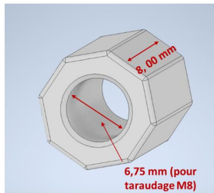
Figure 3.13. Raccord modélisé pour l'assemblage de la buse et de la seringue.
