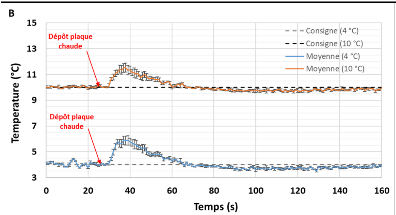
Figure 1.33. Evaluation de la réponse de la régulation thermique du module à effet Peltier suite au dépôt de matière chaude : A – Dépôt d’un cylindre de gélatine préalablement chauffé à 30 °C ; B – Dépôt d’une plaque d’aluminium de 2 mm d’épaisseur, de surface égale à celle de la plaque d’impression (16 cm 2 ) et préalablement chauffée à 30 °C. Les courbes moyennes sont obtenues à partir de 3 répétitions (barres d’erreur = SEM).
