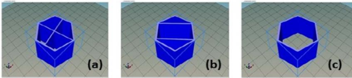
Figure 3.2. Différents types de structure de remplissage de formes hexagonales imprimées en chocolat par (Mantihal et al., 2017) pour l'étude des propriétés mécaniques : A – avec supports croisés ; B – avec supports parallèles ; C – sans support.
