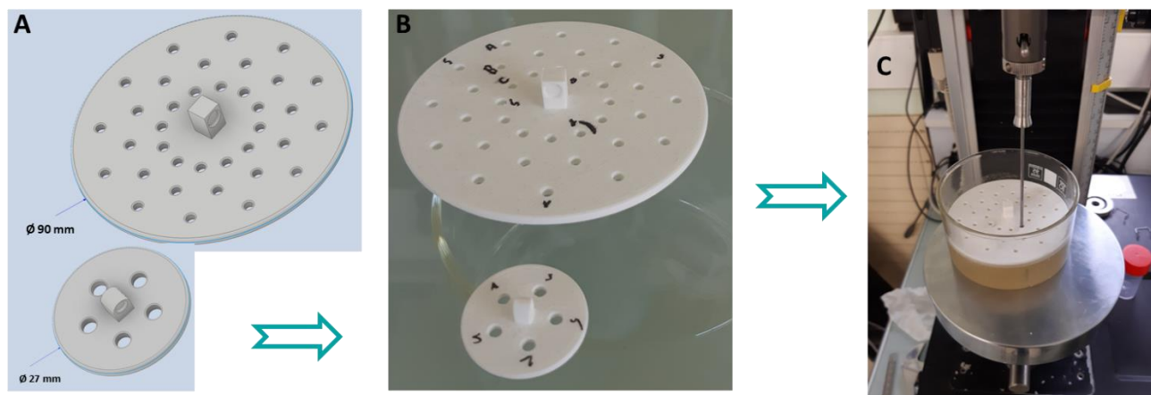
Figure 2.12. Dispositifs permettant de tester la répétabilité des mesures du pénétromètre pour des gels de diamètre 27 et 90 mm. A - Conception des dispositifs (CAO), B – Dispositifs imprimés en 3D (acide polylactique), et C – Mesures sur le texturomètre Instron dans le cas d'un gel de 90 mm de diamètre.
