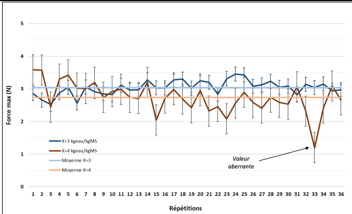
Figure 2.14. Mesures de répétabilité ( n=36 ) de la force maximale avec une sonde de pénétration de 2 mm de diamètre sur des gels de gélatine de 90 mm de diamètre et de teneurs en eau égales à 3 \text{kg}_{\text{eau}}/\text{kg}_{\text{MS}} (bleu foncé) et à 4 \text{kg}_{\text{eau}}/\text{kg}_{\text{MS}} (bleu foncé). Les barres d'erreur correspondent à l'écart-type. Une valeur aberrante a été mise en évidence par le test de Grubbs ( P\text{-value} = 0,01 ) pour la mesure 33 (gel à 4 \text{kg}_{\text{eau}}/\text{kg}_{\text{MS}} ).
