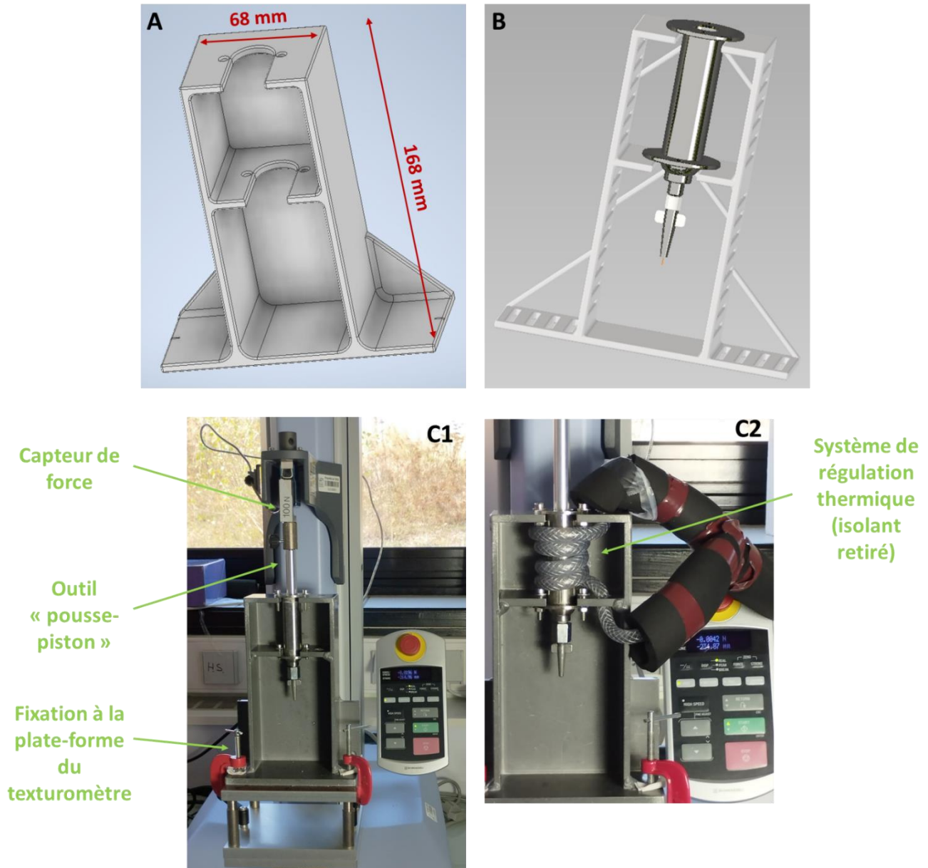
Figure 3.16. Représentations schématiques et photographies du bâti qu'il a été nécessaire de concevoir afin de permettre le positionnement de la seringue et de la buse d'extrusion sur le texturomètre. A – Modélisation CAO du bâti ; B – Assemblage CAO (le raccord (Figure 3.13) n'est pas positionné pour plus de lisibilité) ; C1 et C2 – Photographies après installation sur le texturomètre.
