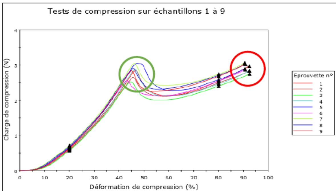
Figure 2.11. Effet d'une sonde de pénétration de 10 mm de diamètre sur un gel de gélatine. Malgré une répétabilité acceptable ( n=9 répétitions), la charge de compression est faible, proche de la limite de détection du capteur de force et, la déformation liée à la compression se traduit par 2 pics (entourés en vert et en rouge). Le second pic (entouré en rouge) se produit après la fracture du gel.
