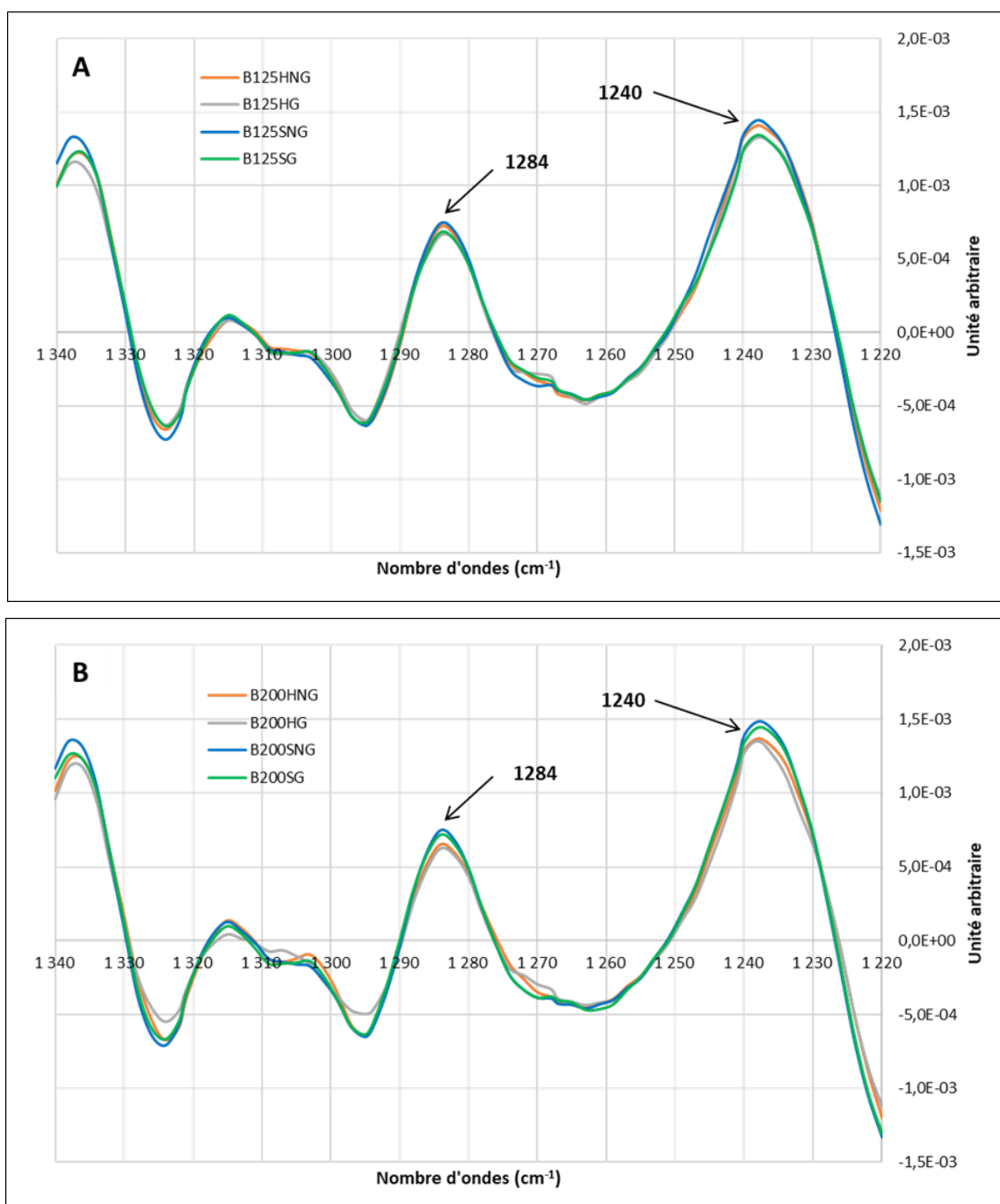
Figure 2.35. Représentation des courbes moyennes obtenues à partir de 3 répétitions pour la bande spectrale attribuée à l'Amide III, après dérivée seconde des spectres. (–) condition humide/non-glyquée (HNG) ; (–) condition humide/glyquée (HG) ; (–) condition sèche/non-glyquée (SNG) ; (–) condition sèche/glyquée (SG). A – Gélatine d'indice Bloom 125 ; B – Gélatine d'indice Bloom 200.
