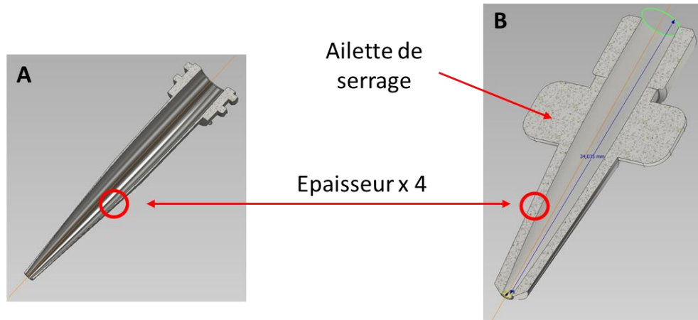
Figure 3.12. Vue en coupe d'une : A – buse d'extrusion, dont la paroi a une épaisseur de 0,25 mm ; et B – buse d'extrusion dont la paroi a été renforcée à 1 mm d'épaisseur, de façon à éviter toute déformation lors de l'impression 3D métal.
