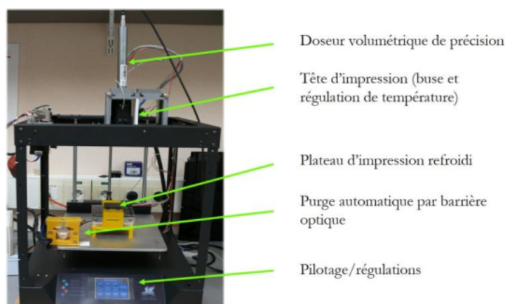
Figure 2 : Prototype d'imprimante 3D dédiée à la conception d'aliments fonctionnels carnés ou multi-sourcés.
