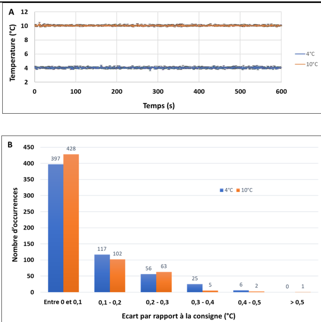
Figure 1.32. Evaluation de la régulation de la température du module à effet Peltier placé sous le plateau d'impression du second prototype d'imprimante développé au laboratoire : A – Stabilité de la régulation du module à effet Peltier pour une consigne fixée à 4 °C et à 10 °C (les barres d'erreur correspondent à la SEM) ; B – Classement par occurrence de la valeur absolue de la différence entre la température mesurée et la température de consigne.
