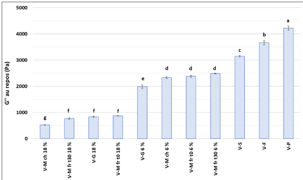
Figure 3.36. Classement des formulations selon la limitation de l'écoulement avant impression (valeur du module de perte – G'' au repos au cours d'un balayage en déformation). Des lettres identiques signifient une absence de différence significative entre les formulations (analyse de variance, test Post-hoc de Tukey, P > 0,05 ). Les barres d'erreur correspondent aux SEM, calculées à partir de 3 répétitions.
