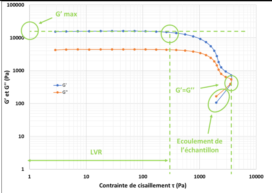
Figure 3.7. Représentation graphique des paramètres rhéologiques, déterminés en régime oscillatoire, sur de la viande de bœuf broyée et tamisée (à 30 °C).
