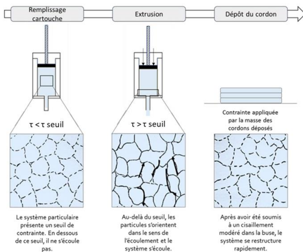
Figure 3.9. Représentation schématique de l'impression 3D de systèmes particulaires concentrés en particules molles. Les flèches noires représentent le glissement des particules les unes sur les autres et sur la paroi de la buse (D'après (Masbernat, 2021)).
