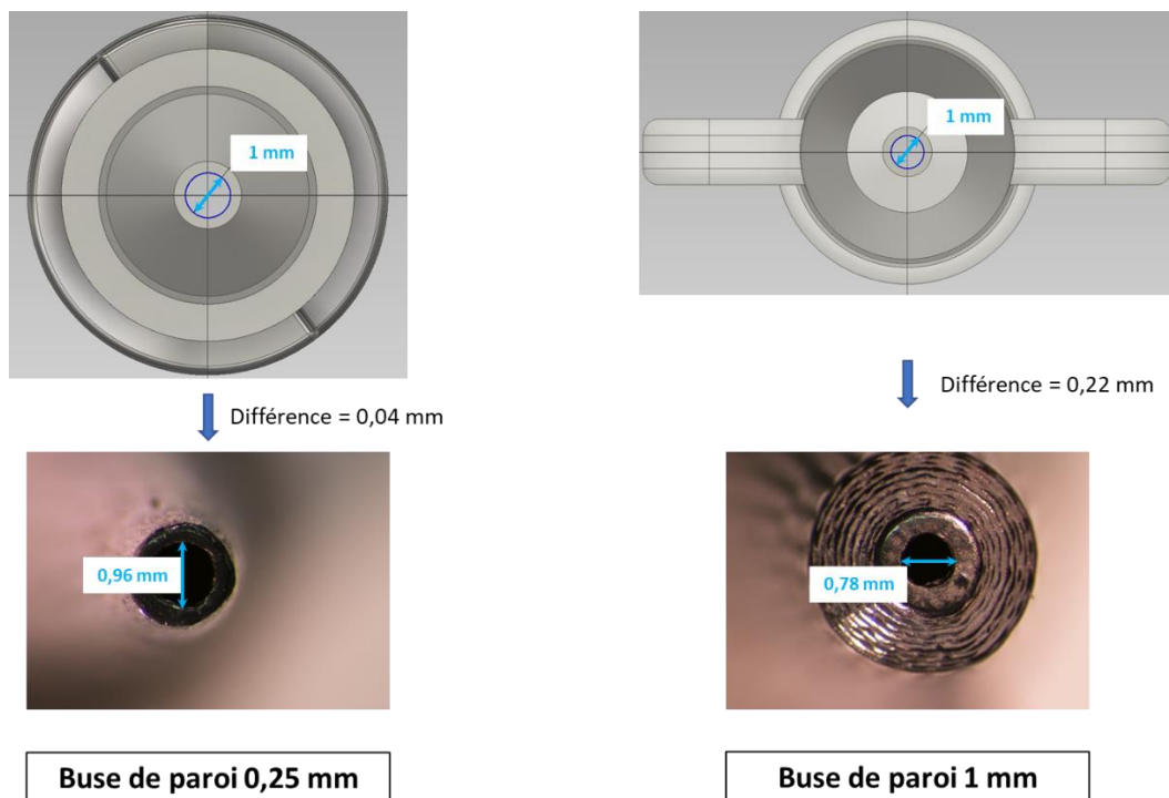
Figure 1.18. Mesure, au moyen d’un stéréomicroscope, du diamètre de buses d’extrusion imprimées en inox 316L. Les écarts mesurés entre les cotes du modèle CAO et les mesures expérimentales sont indiqués. A – buse avec une paroi de 0,25 mm d’épaisseur ; B – buse avec une paroi renforcée de 1 mm d’épaisseur.
