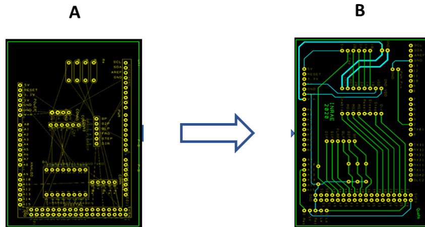
Figure 1.24. Typon du circuit imprimé. A – Connexion automatique des éléments à partir du schéma de câblage. B – Placement manuel des connexions des éléments.
