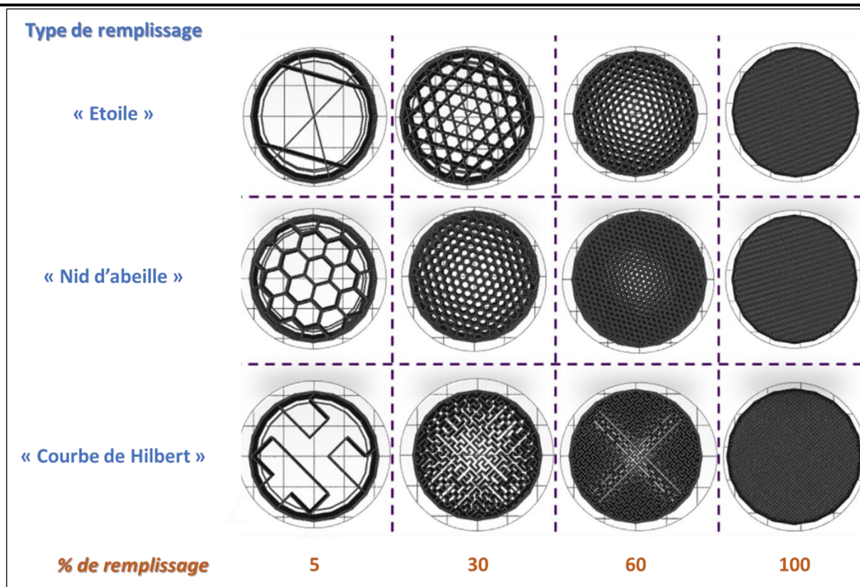
Figure 3.3. Modélisation numérique de différents motifs, à différents pourcentages de remplissage interne, utilisés pour imprimer des structures en chocolat (d'après Mantihal et al., 2019).
