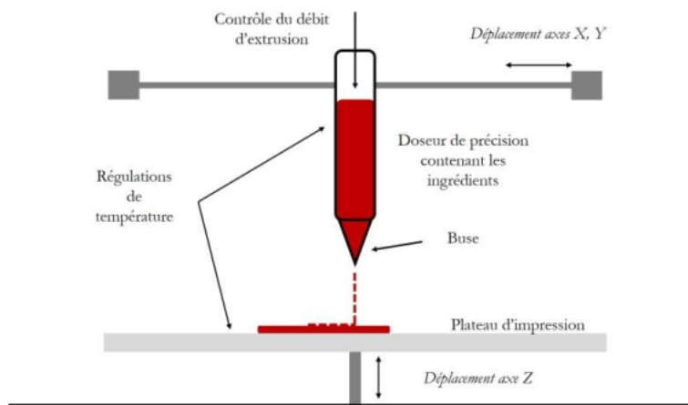
Figure 1 : Représentation schématique d'une imprimante 3D alimentaire.
