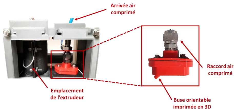
Figure 1.38. Intégration du dispositif de refroidissement additionnel par air comprimé à la tête d'impression du second prototype d'imprimante 3D alimentaire développé au laboratoire.
