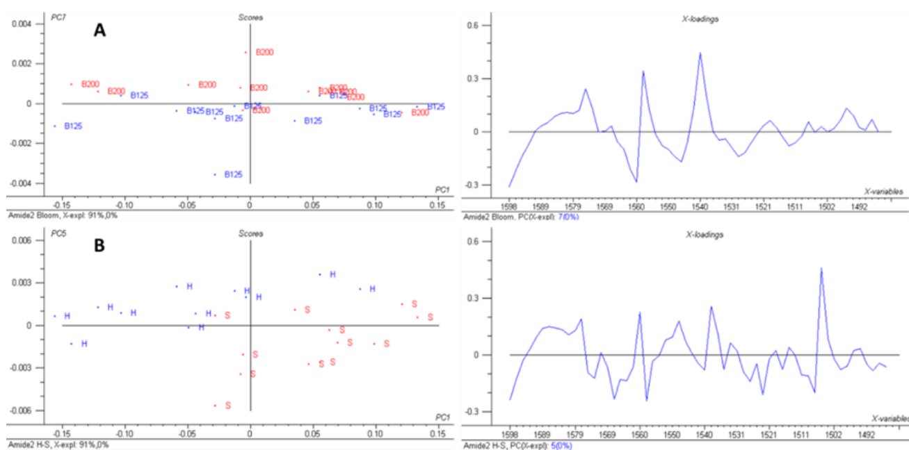
Figure 2.34. Analyses en composante principale. Absorbances mesurées (dérivée seconde) sur la bande spectrale attribuée à la fonction Amide II (1599-1500 \text{cm}^{-1} ). A – Effet de l'indice Bloom (B125 en bleu vs. B200 en rouge) ; B – Effet de la teneur en eau initiale (H vs. S).
