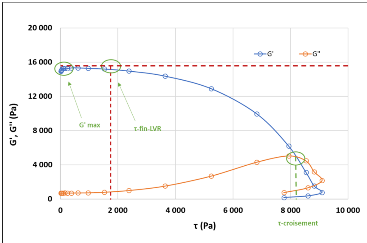
Figure 2.38. Représentation graphique des courbes des modules de stockage ( G' ) et de module de perte ( G'' ), en fonction de la contrainte de cisaillement, obtenues pour un gel de gélatine préparé à base de gélatine d'indice Bloom 125 en condition Sèche/Glyquée (SG). Les paramètres calculés ( \tau -croisement, G' max et \tau -fin-LVR) sont indiqués en vert.
