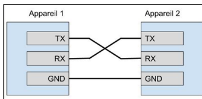
Figure 1.22. Représentation schématique d'une de liaison de type UART ( Universal Asynchronous Receiver-Transmitter ) entre deux appareils.
