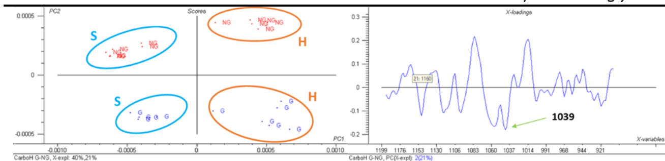
Figure 2.29. Analyse en composante principale. Effet de l'ajout de D -ribose (G vs. NG) et de la teneur en eau initiale (H vs. S), dans des gels de gélatine, sur les absorbances (après dérivée seconde) mesurées au niveau de la bande spectrale attribuée aux glucides (ACP réalisée avec « The Unscrambler »).
