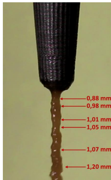
Figure 3.38. Illustration du phénomène d'amincissement par cisaillement. Capture vidéo de l'écoulement d'une matrice constituée de viande pure à la suite d'une extrusion au travers d'une buse de 0,97 mm de diamètre, à une vitesse de 2,08 \text{mm.min}^{-1} . La vidéo a été réalisée avec une caméra Canon EOS 70D (objectif 18/300 réglé à 300 mm), à une fréquence de 25 images par seconde (full HD). L'image présentée a été extraite du film avec le lecteur multimédia VLC 3.0.18 Vetinari.
