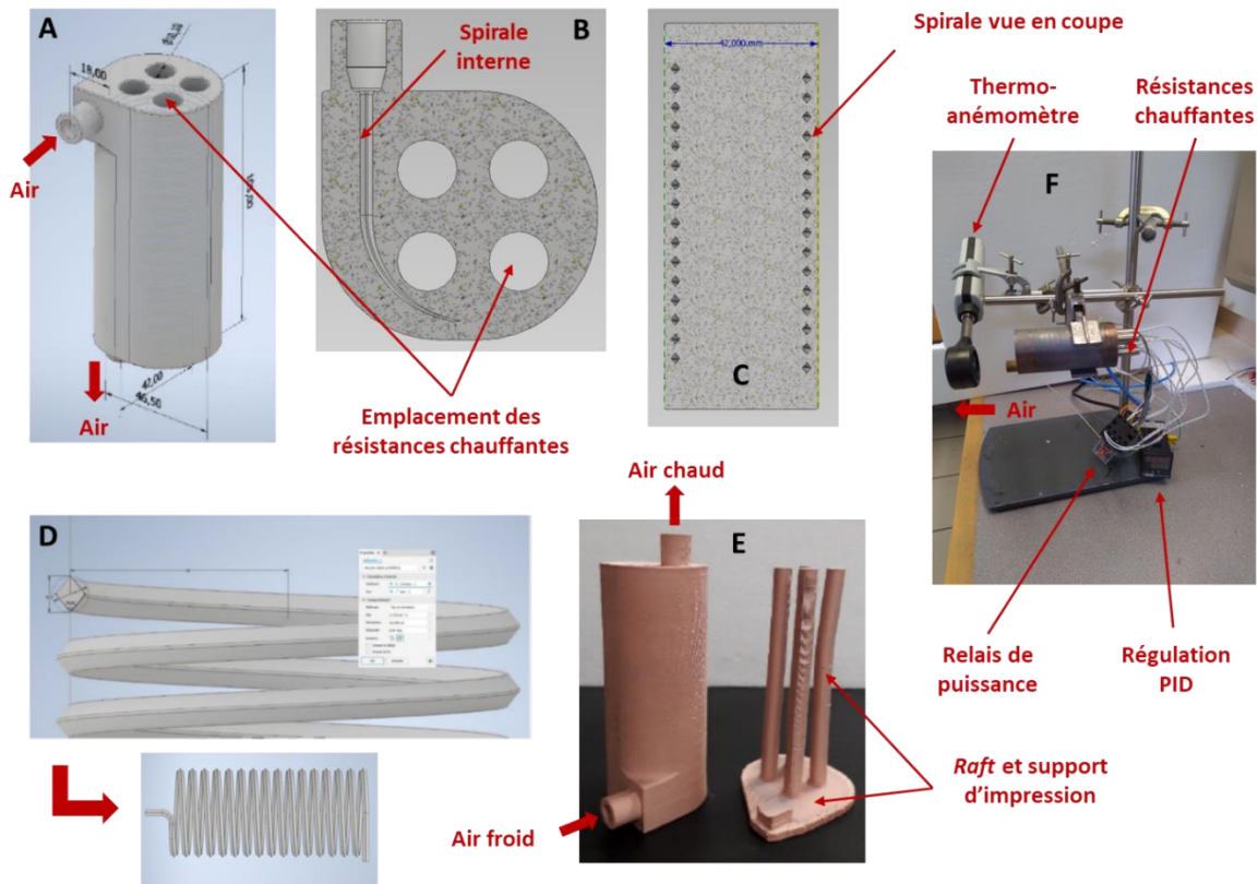
Figure 1.40. Vues détaillées de l'échangeur thermique conçu pour chauffer l'air en vue de procéder à une cuisson de l'aliment en cours d'impression : A – Vue générale de la modélisation CAO ; B – Vue selon une coupe transversale de l'échangeur ; C – Vue selon une coupe longitudinale de l'échangeur ; D – Vue modélisée de la spirale interne dans laquelle l'air circule ; E – Vue extérieure du système en cuivre après impression ; F – Installation du dispositif pour la mesure des températures et des vitesses d'air (isolant retiré pour la prise de la photographie).
