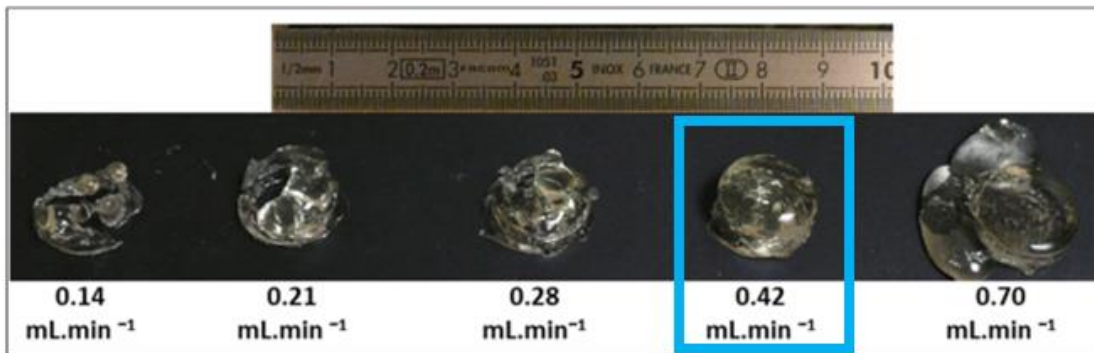
Figure 1.31. Effet du débit d'extrusion sur la géométrie de gels de gélatine imprimés, sachant que l'objectif était d'obtenir un cylindre de 20 mm de diamètre et 10 mm de hauteur.
