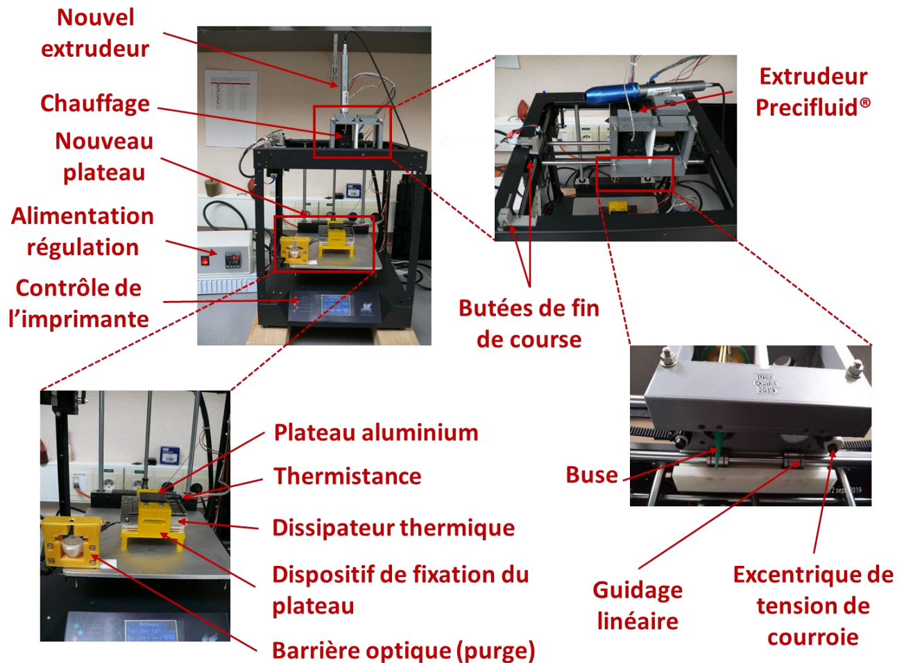
Figure 1.12. Vues des principales modifications apportées (tête et plateau d'impression) à l'imprimante 3D Ghost achetée dans le commerce (à comparer avec la Figure 1.3a) pour le développement du second prototype d'imprimante 3D alimentaire.
