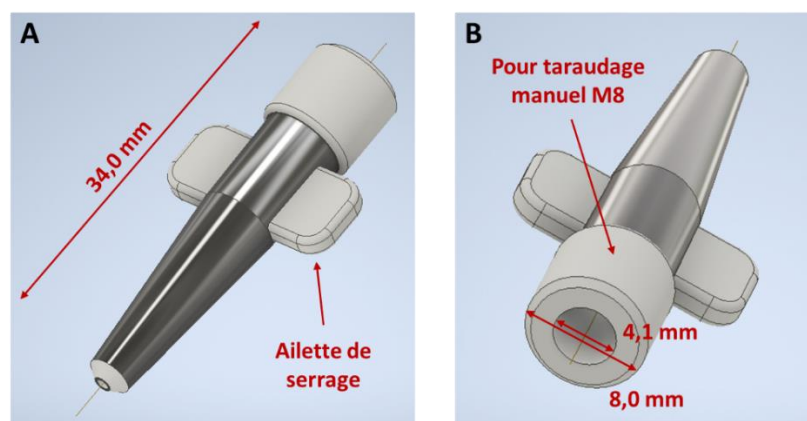
Figure 3.14. Vue entière de la nouvelle buse d'extrusion. A – Vue avant (orifice d'extrusion) ; B – Vue arrière (connexion à la seringue).
