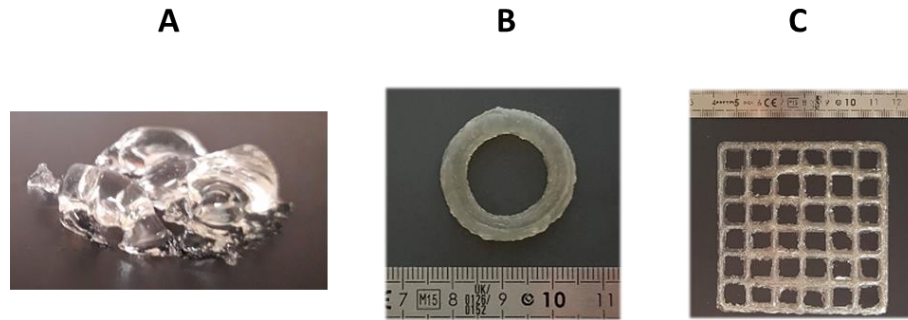
Figure 1.11. Exemples de gels imprimés avec le premier prototype d'imprimante 3D alimentaire, conçu au laboratoire, sur la base d'une imprimante 3D du commerce (modèle Prusa i3). A – gel ne contenant pas d'alginate, B et C – gels contenant des alginate.
