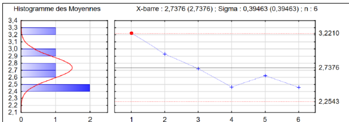
Figure 2.15. Evaluation de la répétabilité des mesures de pénétration avec la sonde de 2 mm de diamètre dans des gels de gélatine de 90 mm de diamètre. Représentation sous la forme d'une carte de contrôle.
