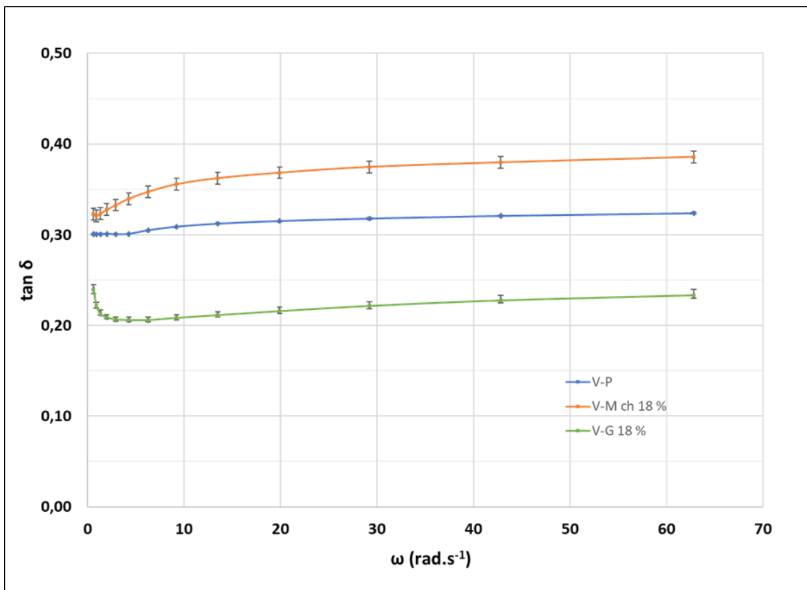
Figure 3.34. Représentation graphique du facteur d'amortissement ( \tan \delta ) moyen calculé à partir d'un balayage en fréquence ( 0,628 - 62,8 \text{ rad.s}^{-1} ) dans la Région Viscoélastique Linéaire (LVR). Les barres d'erreur correspondent aux SEM, calculées à partir de 3 répétitions.
