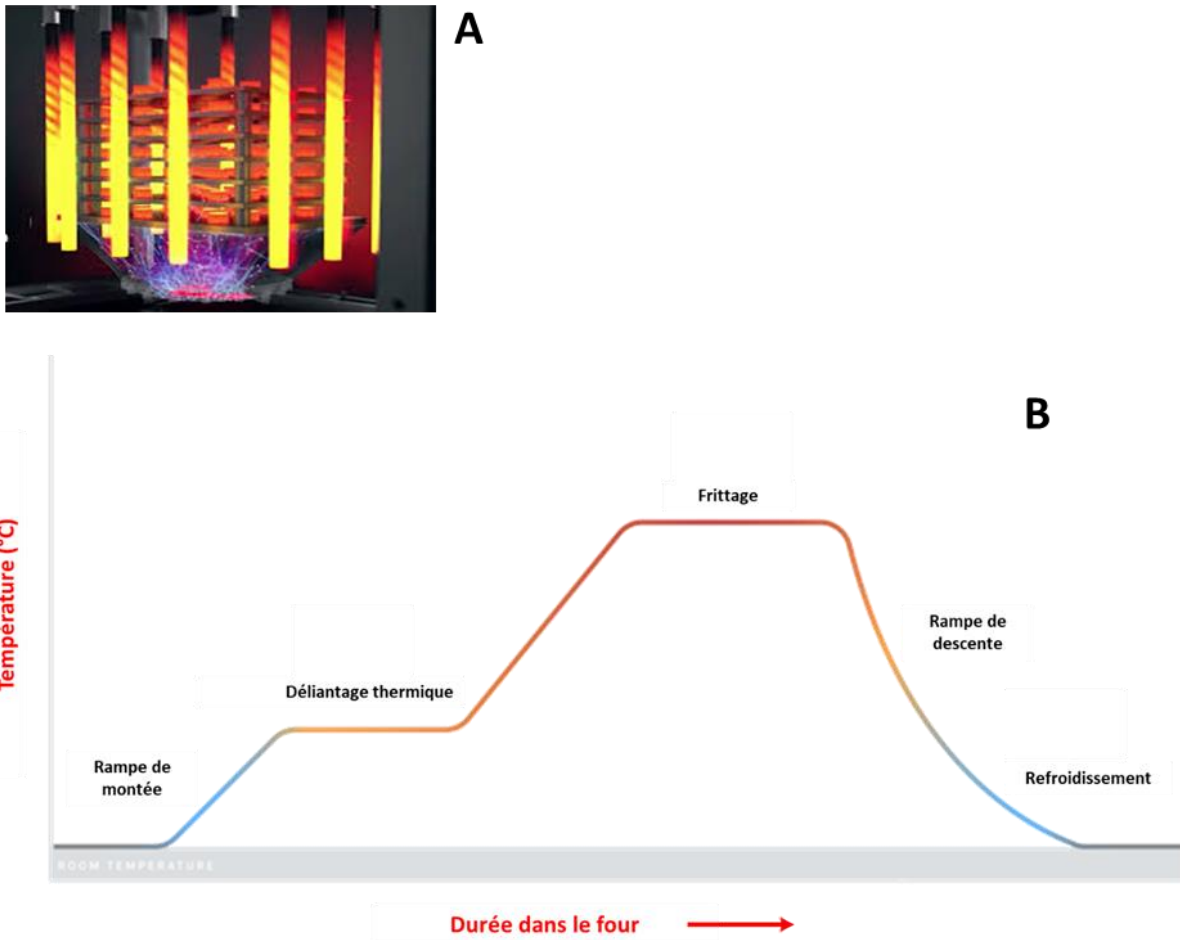
Figure 1.5. Système d'impression 3D métal basé sur la technologie Bound Metal Deposition : A – Illustration du système de chauffage du four de frittage ; les pièces à traiter sont placées au sein d'un boîtier en graphite entouré de résistance chauffantes ; B – Cycle de température au cours de l'étape de frittage.
