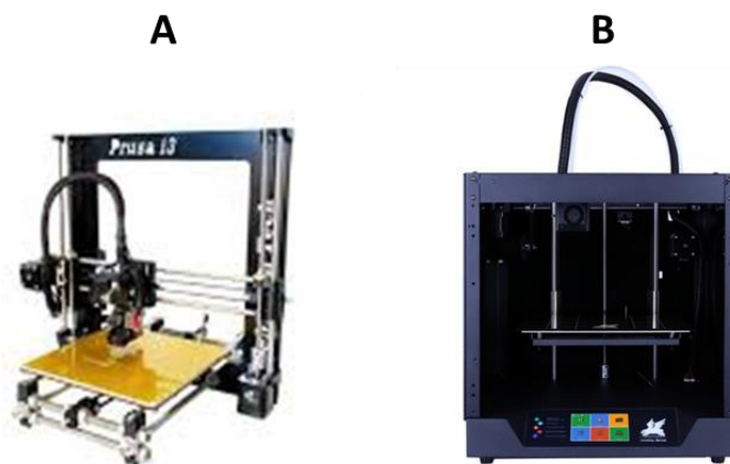
Figure 1.3. Images des deux imprimantes 3D achetées en kit dans le commerce et qui ont été utilisées pour concevoir au laboratoire deux prototypes d'imprimantes 3D alimentaires : A – Imprimante Prusa i3 ; B – Imprimante Ghost, dans leur configuration d'origine.
