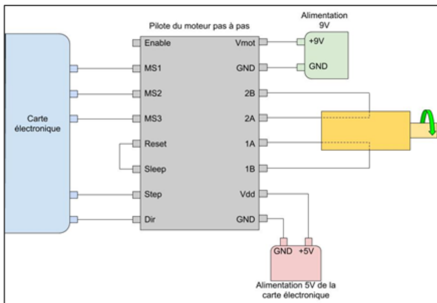
Figure 1.28. Schéma de câblage du circuit pilote du moteur pas-à-pas mis en place pour contrôler l'action du doseur volumétrique Precifluid®.
