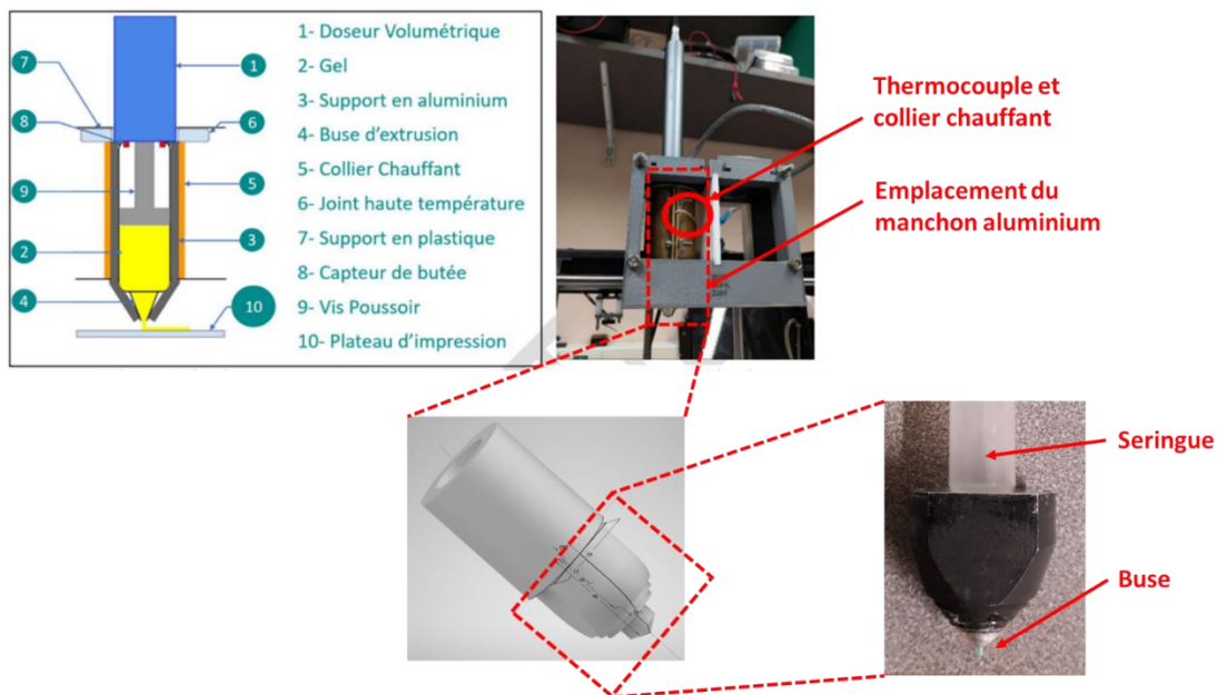
Figure 1.14. Vues détaillées du manchon conducteur en aluminium et du collier chauffant qui ont été installés sur le second prototype d'imprimante 3D alimentaire développé au laboratoire.
