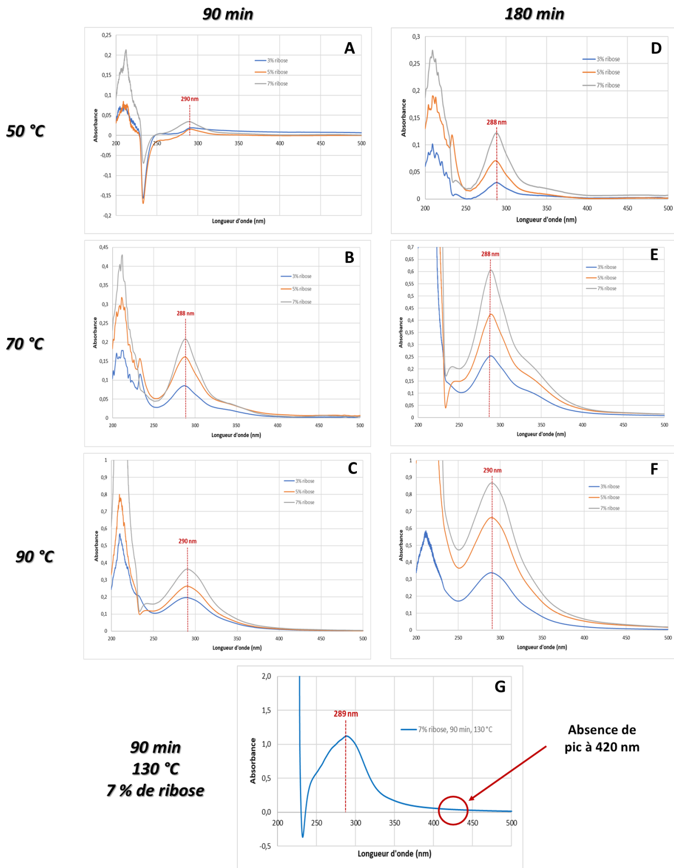
Figure 2.17. Spectres d'absorption de gels de gélatine glyqués en fonction de la durée et des températures réactionnelles. A-C – Spectres obtenus à 50, 70 et 90 °C au bout de 90 min de réaction ; D-E - Spectres obtenus à 50, 70 et 90 °C au bout de 180 min de réaction ; G – condition la plus poussée : 130 °C ; 90 min et 7% de D-ribose.
