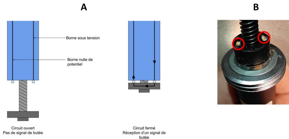
Figure 1.27. A – Schéma de fonctionnement de la butée et, B – Butées physique du doseur volumétrique Precifluid® (entourée en rouge).
