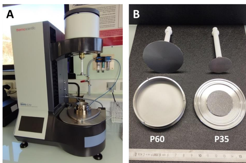
Figure 3.18. Photographies : A – Rhéomètre HAAKE MARS iQ Air ; B – Géométries de type plan-plan de 60 et 35 mm de diamètre, utilisées pour caractériser le comportement rhéologique des différentes formulations d'aliments.
