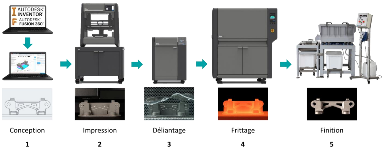
Figure 1.4. Processus de conception, de fabrication et post-traitement d'une pièce métallique (acier inoxydable 316L) par impression 3D, selon la méthode BMD – Exemple de l'équipement Studio System+ (DeskTop Metal™) acheté au laboratoire.
