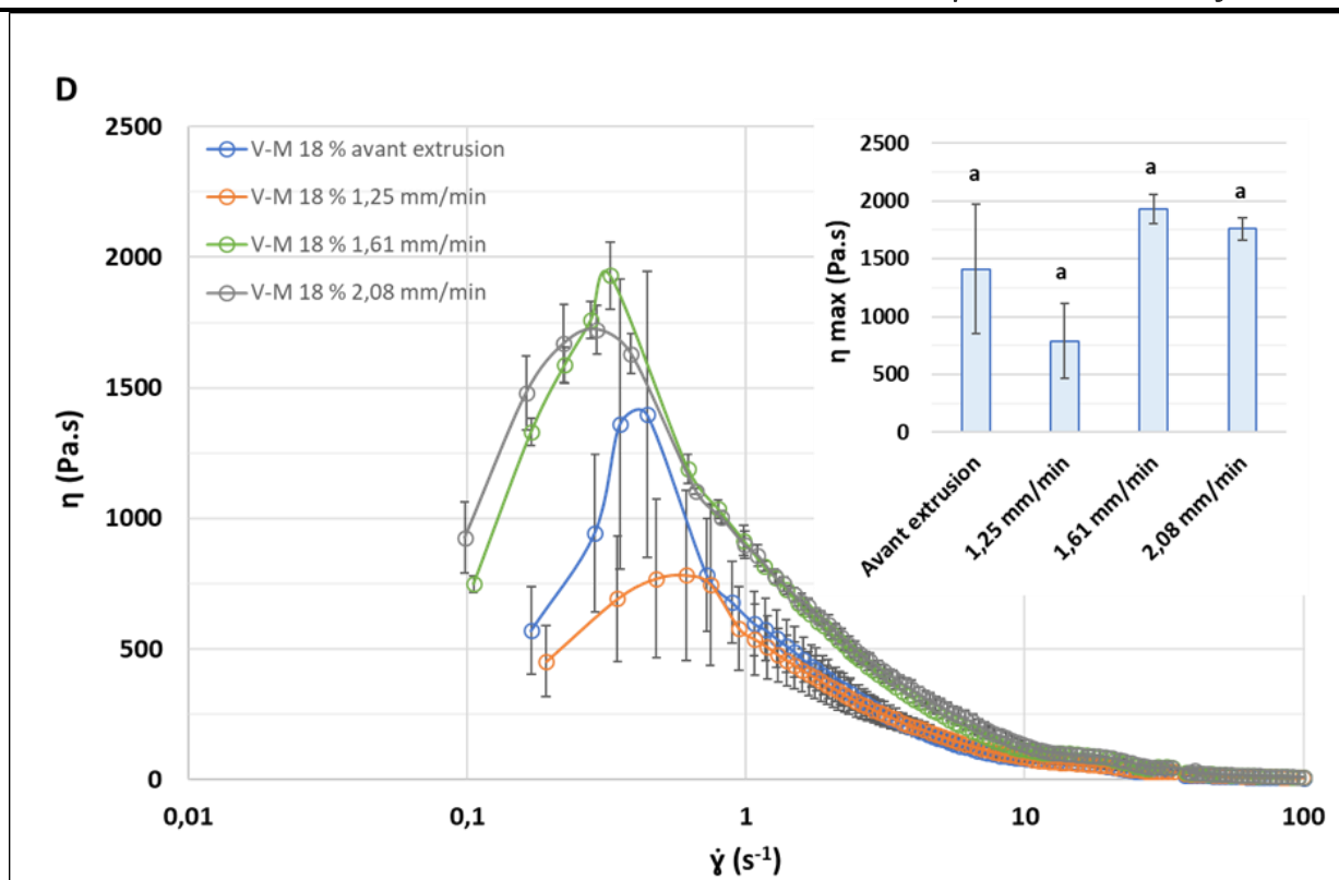
Figure 3.40. Effet de l'extrusion au travers d'une buse d'impression 3D à des vitesses de 1,25 ; 1,61 et 2,08 mm.min -1 sur la viscosité apparente, en fonction du taux de cisaillement, de formulations à base de viande : A – viande pure (V-P) ; B – Viande salée (V-S) ; C – viande + 6 % de mucilage extrait à chaud ; D – viande + 18 % de mucilage extrait à chaud. Les graphiques en histogrammes représentent, pour chaque formulation, les analyses statistiques réalisées sur les viscosités apparentes maximales. Des lettres identiques signifient une absence de différence significative entre les formulations (analyse de variance, test Post-hoc de Tukey, P > 0,05 ). Les barres d'erreur correspondent aux SEM, calculées à partir de 3 répétitions.
