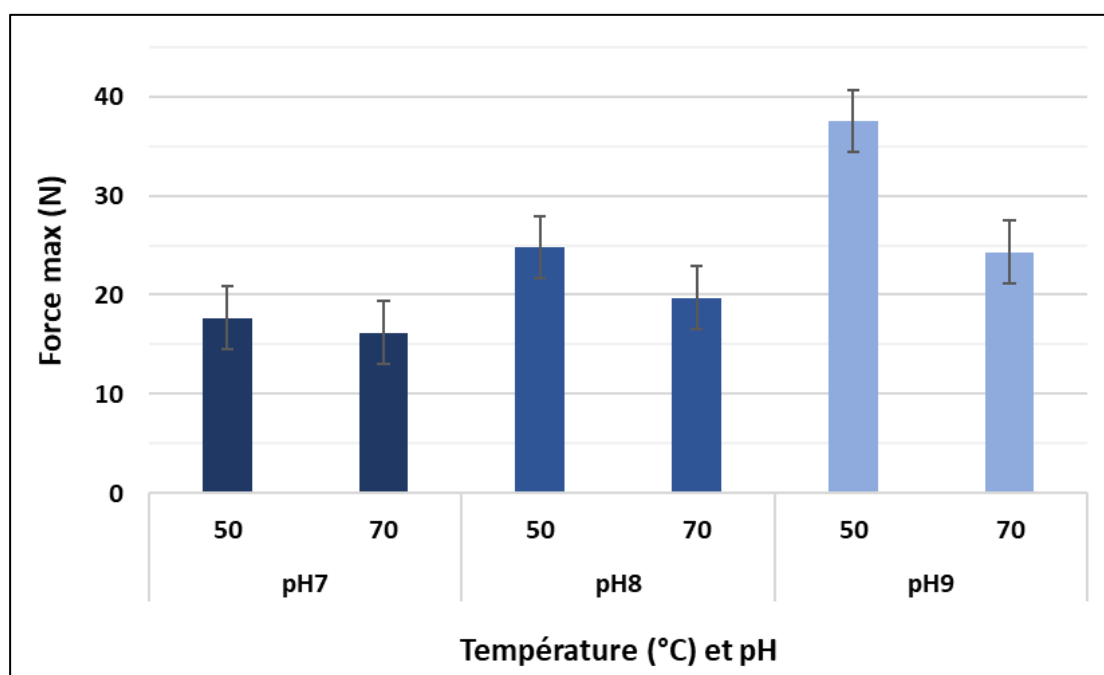
Figure 2.21. Force maximale du gel mesuré au texturomètre en fonction du pH et de la température réactionnelle, avec 5 % de D-ribose. Préparation avec du tampon Tris 1 M. Les barres d'erreur correspondent à l'erreur standard à la moyenne (SEM).
