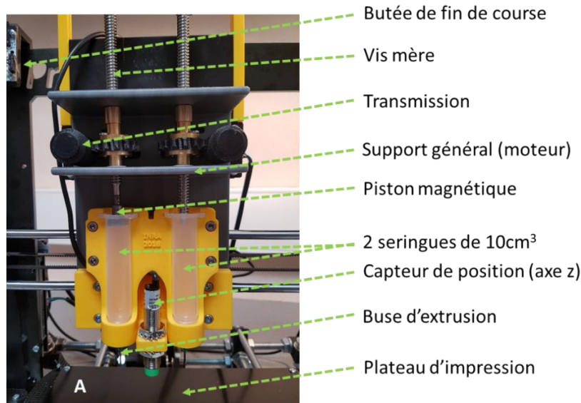
Figure 1.9. Vue de la tête d'impression conçue pour l'extrusion de gels protéiques et installée sur le premier prototype d'imprimante alimentaire, développé à partir d'une imprimante 3D du commerce (modèle Prusa i3).
