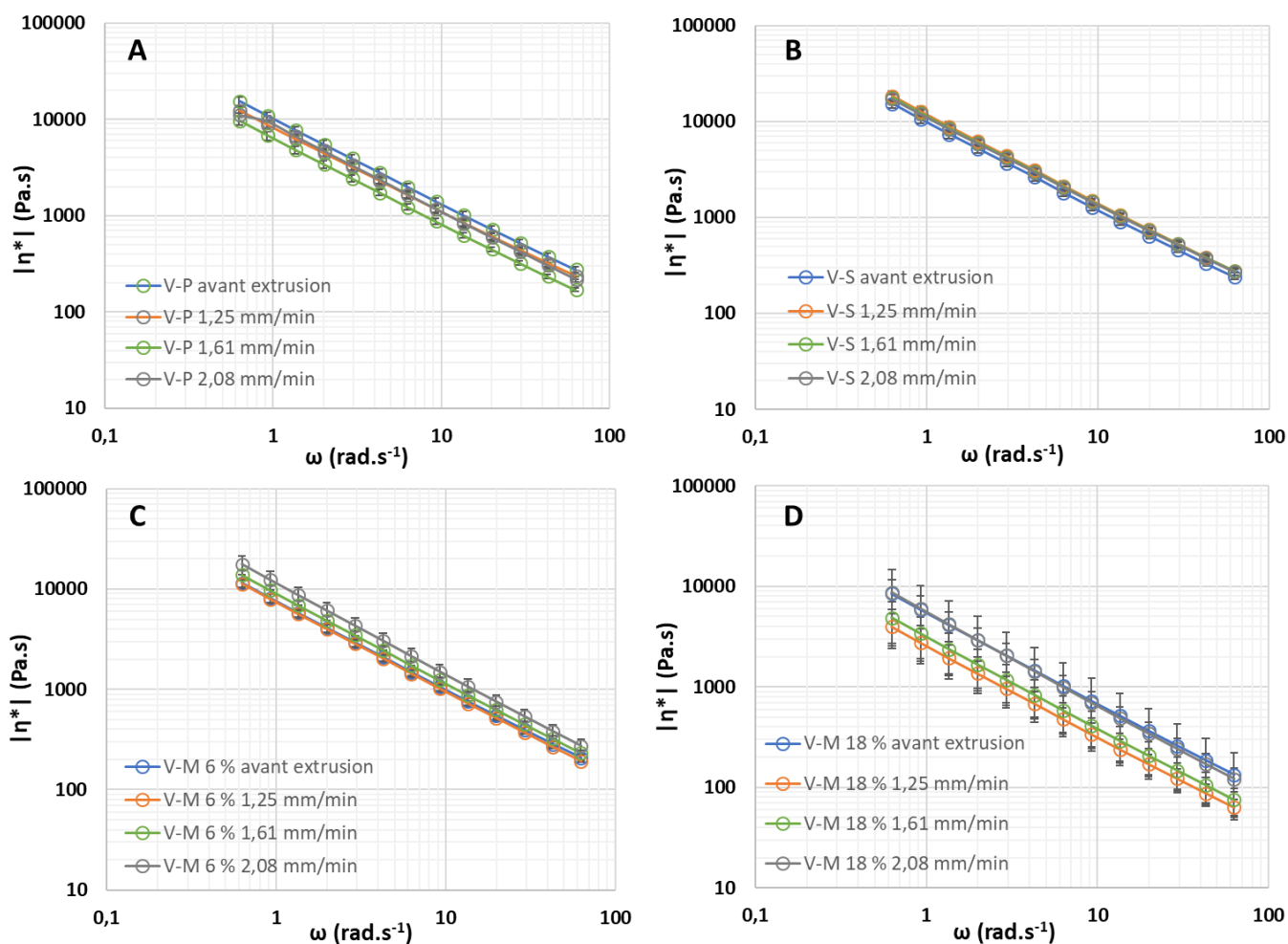
Figure 3.41. Effet de l'extrusion au travers d'une buse d'impression 3D, à des vitesses de 1,25 ; 1,61 et 2,08 mm.min -1 , sur la viscosité complexe de formulations à base de viande : A – viande pure (V-P) ; B – Viande salée (V-S) ; C – viande + 6 % de mucilage extrait à chaud ; D – viande + 18 % de mucilage extrait à chaud. Les barres d'erreur correspondent aux SEM, calculées à partir de 3 répétitions.
