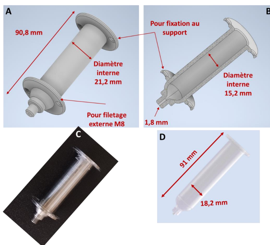
Figure 3.10. Prototype de seringue en acier inoxydable 316L développé au laboratoire. A – Vue entière de la modélisation CAO de la seringue ; B – Vue en coupe de la modélisation CAO ; C – Seringue après impression et reprise d'usinage ; D – Seringue plastique utilisée dans l'imprimante 3D alimentaire.
