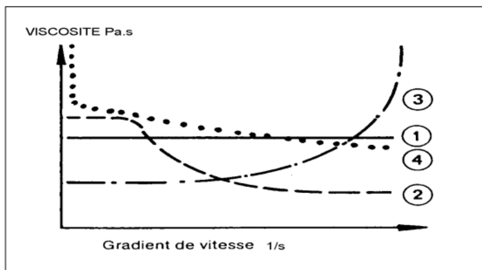
Figure 3.5. Allures des courbes de viscosité pour différents types de fluides : 1) fluides Newtoniens ; 2) fluides non-Newtoniens rhéofluidifiants ; 3) fluides non-Newtoniens rhéoépaississants ; 4) fluides non-Newtoniens plastiques (D'après Schramm, 1981).
