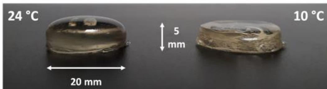
Figure 1.35. Effet de la température du plateau d'impression (10 et 24 °C) sur la géométrie de cylindres de gel de gélatine de 20 mm de diamètre et de 5 mm de hauteur.
