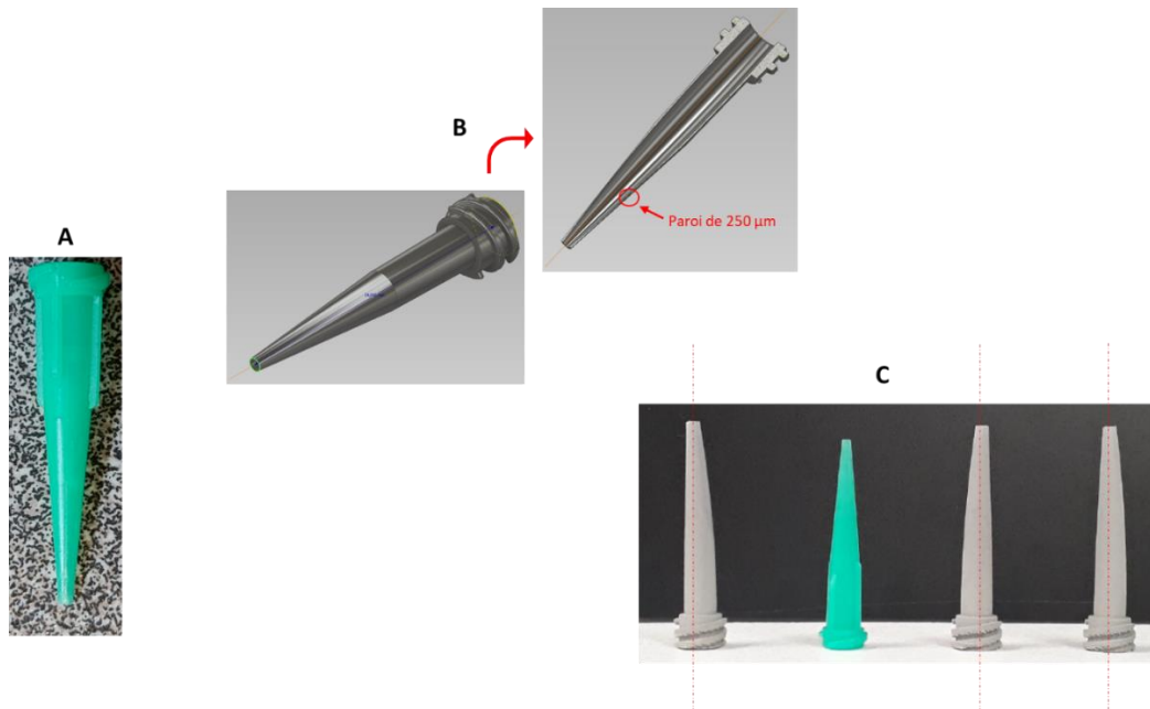
Figure 1.16. Conception et fabrication de buses d'extrusion métalliques. A – Exemple de buse en plastique du commerce ; B – Buse modélisée par CAO, et C – résultats d'impression de buses au moyen de l'imprimante 3D métal.
