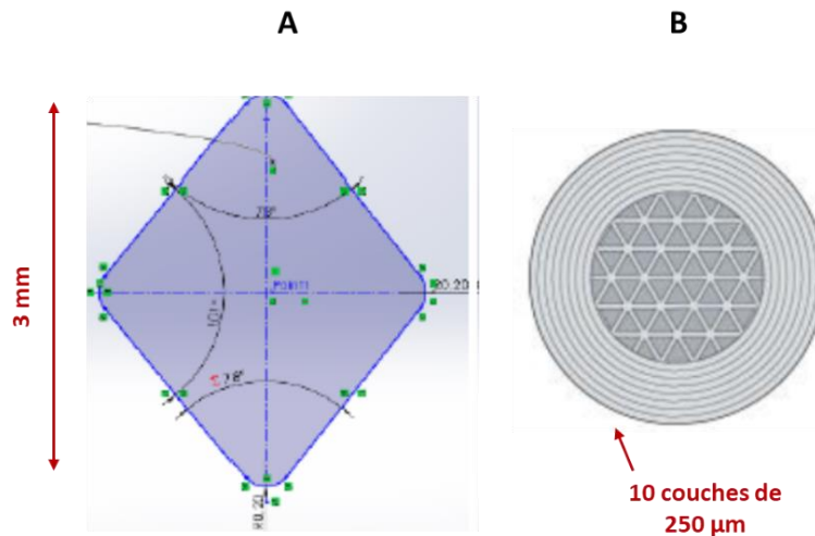
Figure 1.41. A – Modélisation de la section autoportante de la spirale interne de l'échangeur. B – Motif de remplissage interne et épaisseur de paroi du bloc de cuivre.
