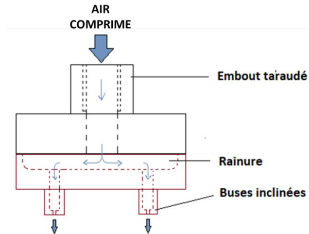
Figure 1.37. Schéma de principe du système de refroidissement additionnel par air comprimé, installé pour permettre au produit imprimé de conserver sa forme, au fur et à mesure de l'impression.
