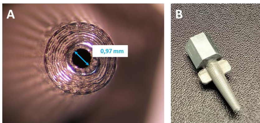
Figure 3.15. Buse d'extrusion imprimée en 3D métal et destinée au simulateur d'extrusion. A - Diamètre de l'extrémité de la buse après reprise d'usinage et mesuré au stéréo-microscope ; B – Buse soudée dans le raccord à vis.
