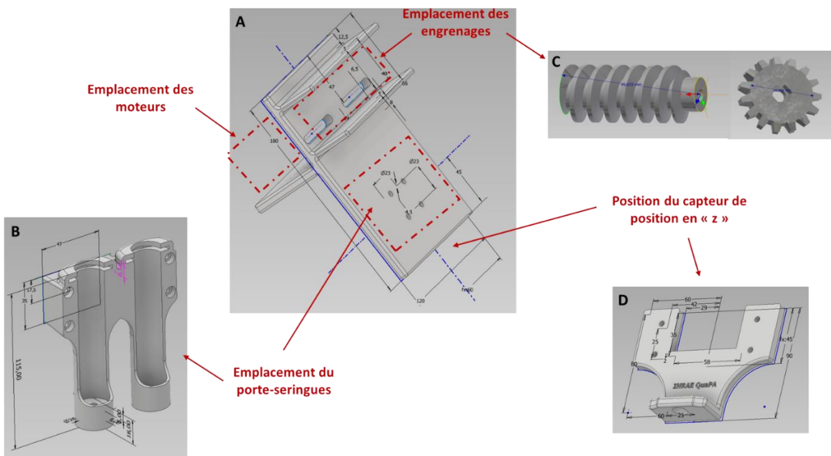
Figure 1.10. Plans de conception de la tête d'impression développée et adaptée sur une imprimante 3D du commerce (modèle Prusa i3). A – Support global ; B – Dispositif porte-seringue ; C – Vis sans fin et pignon de transmission ; D – Support du capteur de position selon l'axe z.
