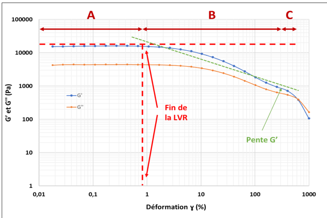
Figure 3.6. Représentation graphique de la Région Viscoélastique linéaire, d'un échantillon de viande de bœuf broyé et tamisé (à 30 °C), calculée à partir de courbes expérimentales de balayage en déformation. La déformation \gamma est ici exprimée en % sur une échelle logarithmique. Zone A – La déformation appliquée n'a pas d'effet sur la microstructure de l'échantillon ; Zone B – La déformation est réversible ; Zone C – La déformation est irréversible, l'échantillon s'écoule.
