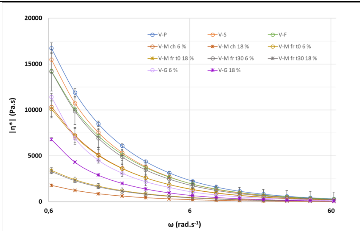
Figure 3.37. Visualisation du comportement d'amincissement par cisaillement des différentes formulations par représentation de leur viscosité complexe en fonction de la fréquence d'oscillation. Les barres d'erreur correspondent aux SEM, calculées à partir de 3 répétitions.
