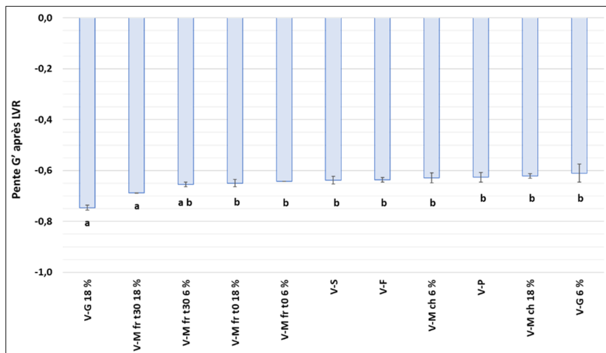
Figure 3.35. Classement des formulations selon la cohésion de la matrice (calcul de la pente de la courbe du module de conservation – G' après le seuil d'écoulement). Des lettres identiques signifient une absence de différence significative entre les formulations (analyse de variance, test Post-hoc de Tukey, P > 0,05 ). Les barres d'erreur correspondent aux SEM, calculées à partir de 3 répétitions.
