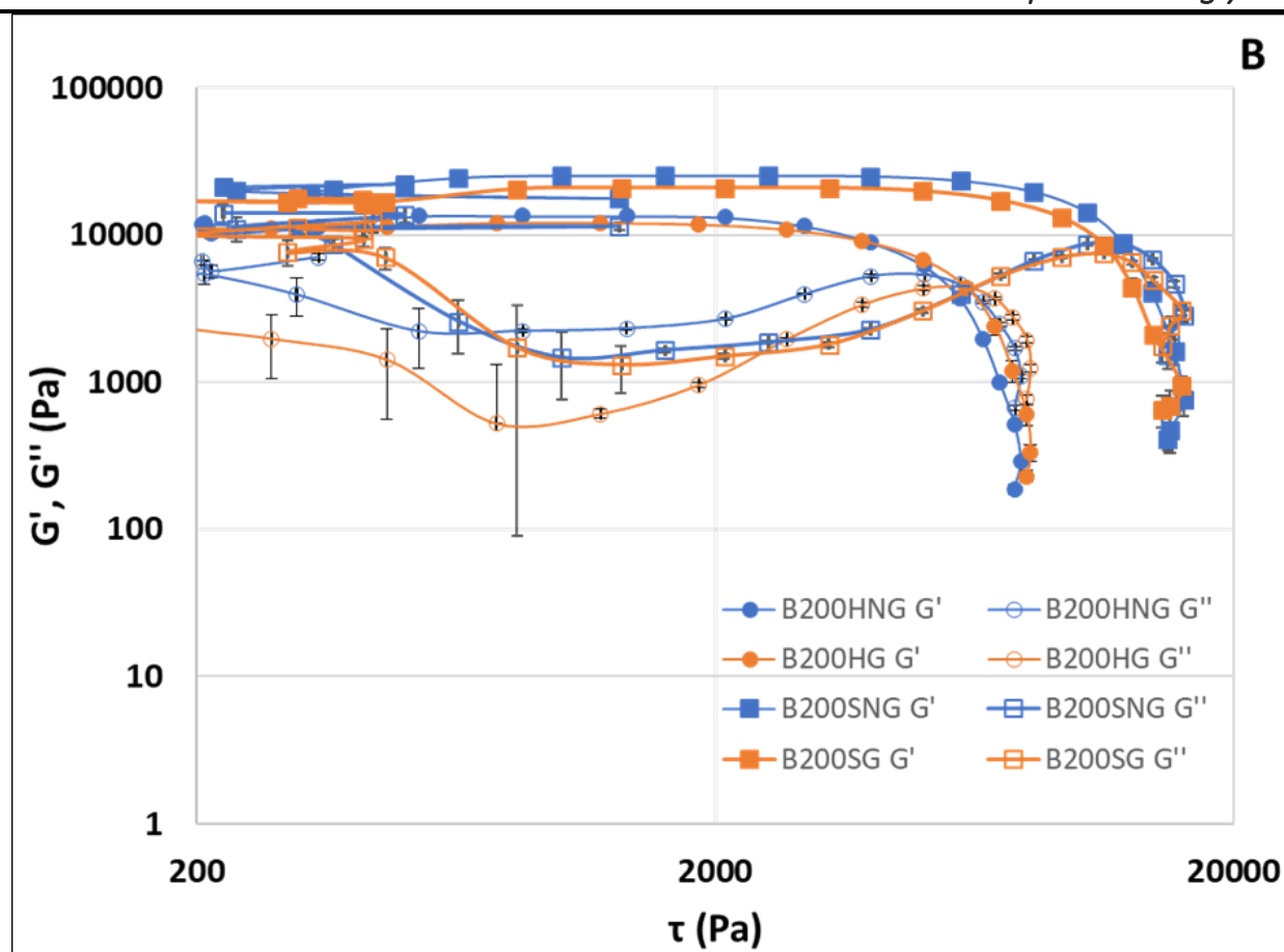
Figure 2.39. Courbes moyennes du module de stockage ( G' ) et du module de perte ( G'' ). A - Courbes moyennes G' et G'' pour les conditions Bloom 125-Humide et B125-Sèche. B - Courbes moyennes G' et G'' pour les conditions Bloom 200-Humide et B200-Sèche. Ces courbes ont été calculées à partir de la moyenne de 3 répétitions, les barres d'erreur correspondant à l'erreur standard à la moyenne (SEM).
