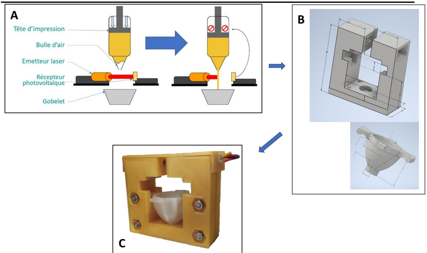
Figure 1.20. Barrière optique permettant la purge automatique du Precifluid®. A – représentation schématique du fonctionnement de la barrière optique, B – plan de conception et, C – la barrière optique imprimée en 3D.
