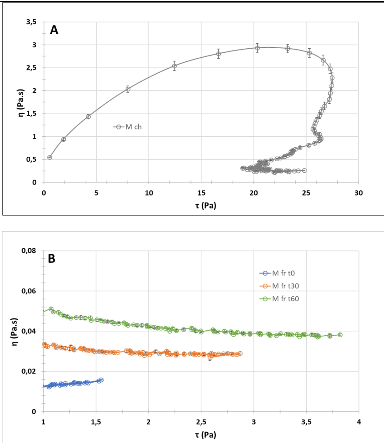
Figure 3.21. Evolution de la viscosité apparente des différents mucilages, à 30 °C, en fonction de la contrainte de cisaillement : A – Mucilage extrait à chaud ; B – Mucilages extraits à froid avec des durées de sonication de 0, 30 et 60 min, respectivement. Ces courbes ont été obtenues à partir de 3 répétitions. Les barres d'erreur correspondent aux SEM.
