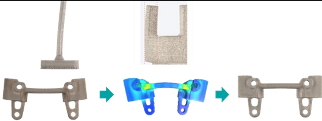
Figure 1.6. Exemple de déformations possibles au cours de l'étape de frittage, la géométrie et la position des supports doivent être optimisées en amont.
