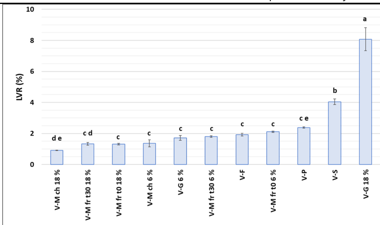
Figure 3.29. Classement des formulations selon la longueur de leur Région Viscoélastique Linéaire (LVR) lors d'un balayage en déformation ( 0-1000 \text{ s}^{-1} ). Des lettres identiques signifient une absence de différence significative entre les formulations (analyse de variance, test Post-hoc de Tukey, P > 0,05 ). Les barres d'erreur correspondent aux SEM, calculées à partir de 3 répétitions.
