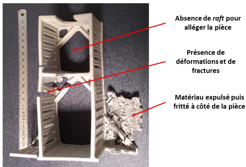
Figure 1.7. Exemple de pièce ayant subi de fortes contraintes thermiques lors de l'étape de frittage, à cause d'un défaut de conception.
