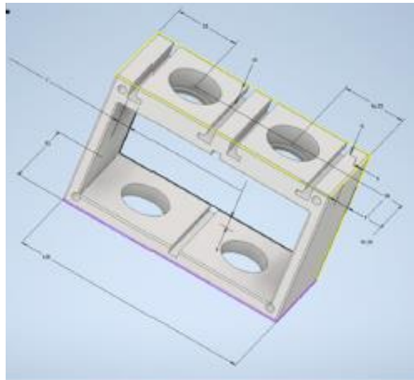
Figure 1.15. Modélisation par CAO du support d'extrudeur comprenant deux emplacements possibles, destinés à recevoir deux têtes d'impression, en vue de réaliser une impression bi-composants.
