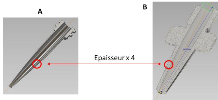
Figure 1.17. Vue en coupe de buses modélisées par CAO : A – buse d’extrusion, dont la paroi a une épaisseur de 0,25 mm ; et B – buse d’extrusion, dont la paroi a été renforcée à 1 mm d’épaisseur, de façon à éviter toute déformation lors de l’impression 3D métal.
