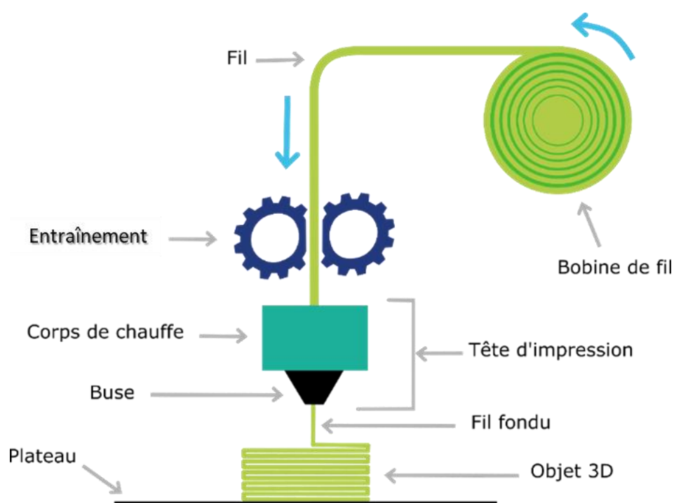
Figure A. Représentation schématique du principe de fonctionnement d'une imprimante 3D à dépôt de fil fondu (exemple d'un matériau polymère) (D'après myago3d.fr ).
