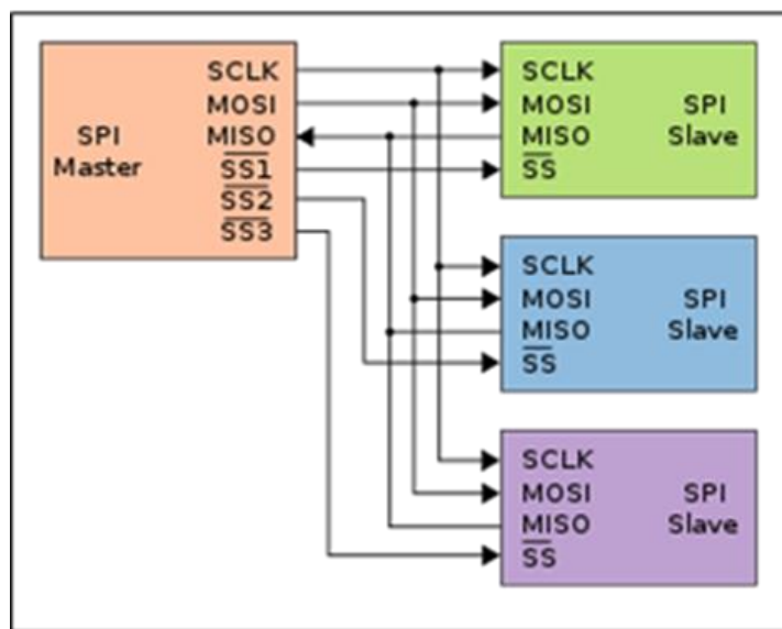
Figure 1.23. Représentation schématique d'une liaison de type SPI (Serial Peripheral Interface) entre un appareil maître et 3 appareils esclaves.
