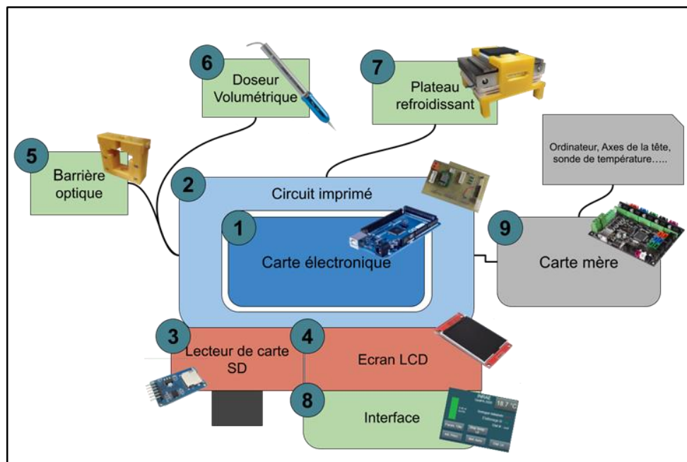
Figure 1.21. Représentation schématique des différents organes ajoutés lors du développement du second prototype d'imprimante 3D alimentaire et, de leurs liens avec le bloc électronique. 1) Carte électronique ; 2) Circuit imprimé (interfaçage de la carte électronique) ; 3) Lecteur de carte SD pour la gestion de l'interface « Homme-machine » ; 4) Ecran tactile LCD ; 5) Barrière optique pour la purge du doseur volumétrique ; 6) Doseur volumétrique Precifluid® ; 7) Plateau refroidissant par système à effet Peltier ; 8) Interface « Homme-machine » ; 9) Carte mère d'origine de l'imprimante.
