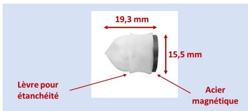
Figure 3.11. Photographie d'un piston en PTFE et acier. Modèle propriétaire, utilisable dans le doseur volumétrique Precifluid®.
