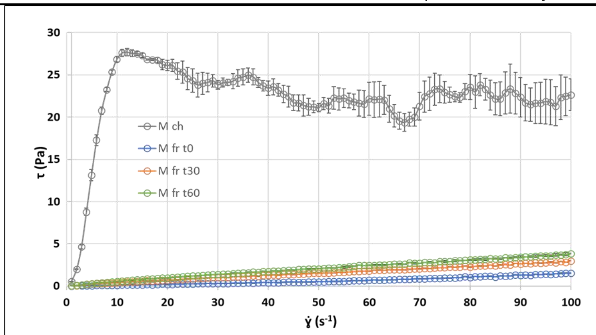
Figure 3.20. Comportement rhéologique à 30 °C du mucilage de graines de lin en fonction du mode d'extraction mis en œuvre. Les temps indiqués pour les mucilages extraits à froid correspondent à des durées de sonication (min). Ces courbes ont été obtenues à partir de 3 répétitions. Les barres d'erreur correspondent aux erreurs standards à la moyenne (SEM).
