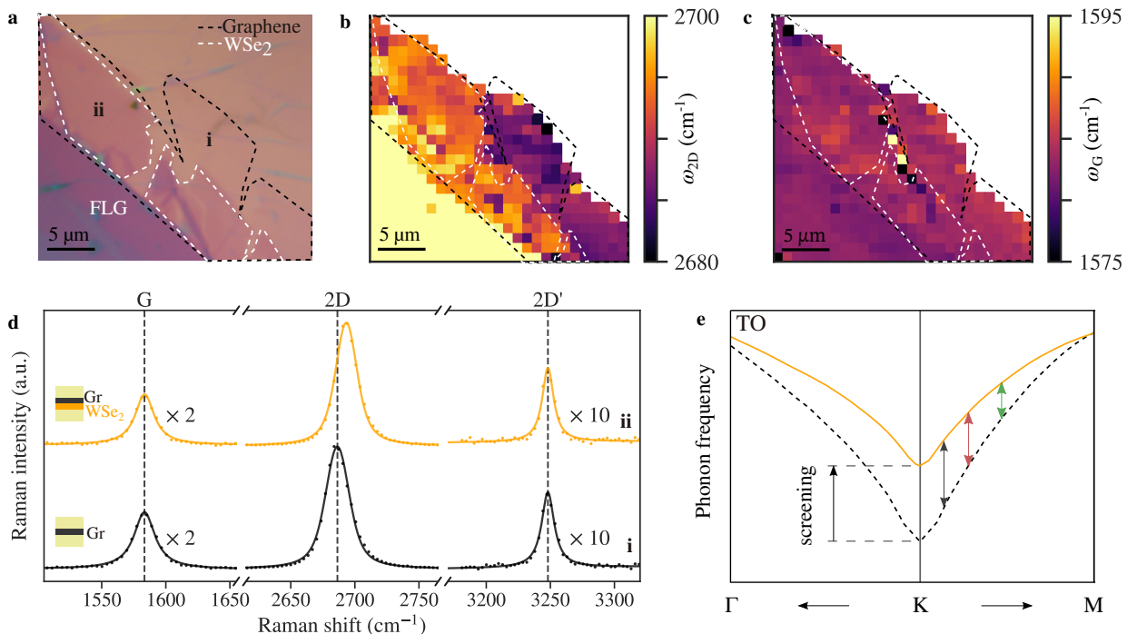
Figure F.9: Cartographie Raman d'un échantillon de graphène/WSe 2 encapsulé. a. Image optique de l'échantillon considéré. b. Cartographie de la fréquence du mode 2D. c. Cartographie de la fréquence du mode G. d. Spectres Raman typique de la zone de graphène encapsulé (i) et de graphène/WSe 2 encapsulé (ii). e. Schéma de l'effet d'adoucissement de l'anomalie de Kohn au point K, K' due à l'écrantage diélectrique.
