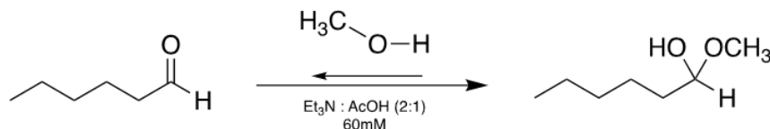
Figure 4. 43. Schéma réactionnel de la formation d l'hémiacétal.
