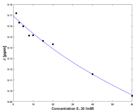
Figure 5. 22. Variation du déplacement chimique en fonction de la concentration. En utilisant le modèle standard d'un équilibre de dimérisation, la constante d'aggrégation est déterminée.
