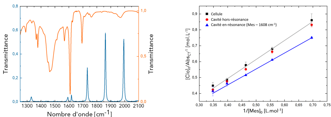
Figure 3. 15. Spectre FT-IR montrant le couplage de la bande située à 1608 cm -1 du mésitylène et le diagramme de Benesi-Hildebrand correspondant (les ■ noirs correspondent aux mesures en cellule, les ● rouges aux mesures de référence en cavité hors résonance et les ▲ bleus aux mesures en cavité en résonance avec la bande Mes - 1608 cm -1 ).
