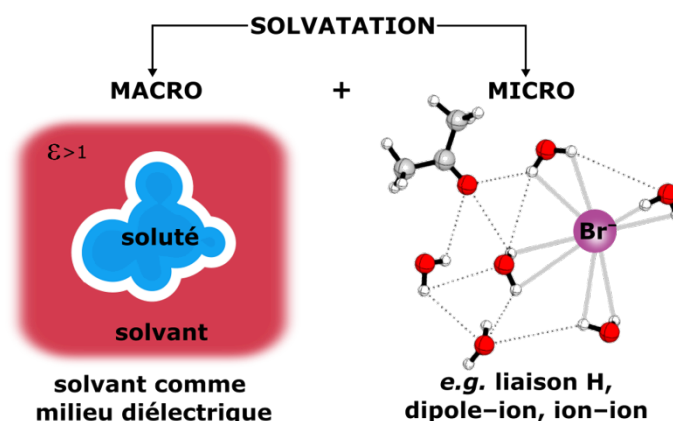
Figure 5. 2. Le concept de polarité peut être divisé en macrosolvatation (le solvant est considéré comme étant un milieu diélectrique) et en microsolvatation (interactions intermoléculaires).
