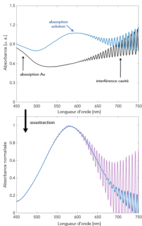
Figure 2. 9. Mesure du spectre d'absorption d'une solution à l'intérieur d'une cavité de Fabry-Pérot. Les spectres de la cavité avec le solvant (en noir) puis avec la solution (en bleu) sont acquis. Le spectre d'absorption du système étudié est obtenu après soustraction (en violet). La qualité du spectre peut être améliorée en utilisant une méthode de lissage (en bleu).
