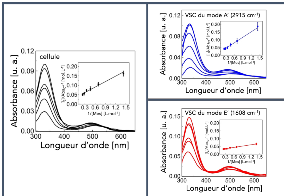
Figure 3. 7. Modification induite par le couplage fort dans les spectres d'absorption du complexe à transfert de charge Mes-I 2 en fonction de la concentration du mésitylène avec (en encadré) le diagramme de Benesi-Hildebrand correspondant. En noir - spectres et diagramme correspondant aux mesures de référence en cellule, en bleu - spectres et diagramme correspondant aux mesures lors du couplage fort de la transition vibrationnelle située à 2915 cm -1 ayant une symétrie A' et en rouge - spectres et diagramme correspondant aux mesures lors du couplage fort de la transition vibrationnelle située à 1608 cm -1 ayant une symétrie E'.
