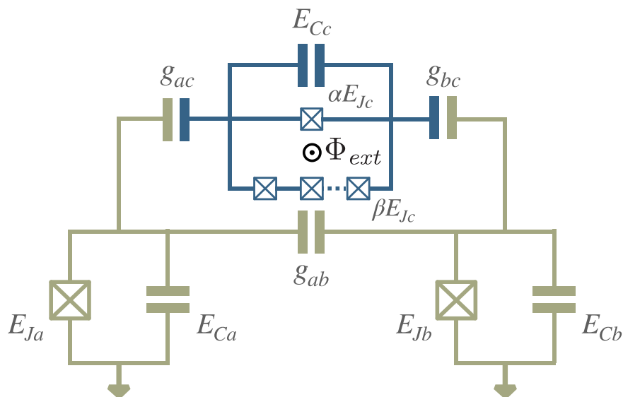
Figure 1 : Schéma du dispositif que nous avons conçu. Les paramètres du circuit sont indiqués en gris avec les indices a et b pour les qubits, et l'indice c pour le coupleur. Les transmons sont en vert et le coupleur en bleu.
