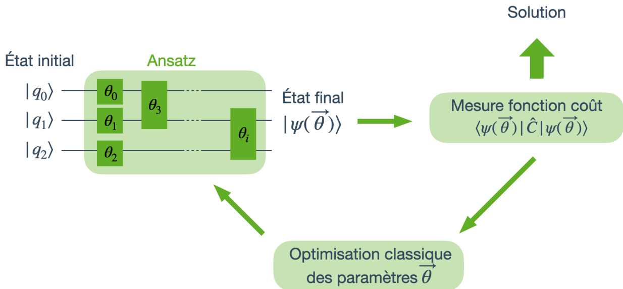
Figure 2 : Schéma du fonctionnement d'un algorithme quantique variationnel.
