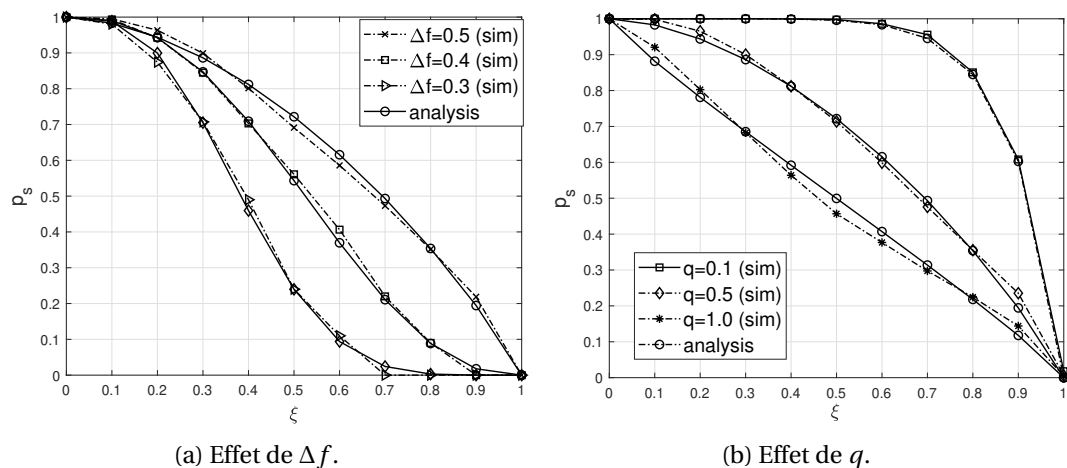
FIGURE 6 – Probabilité de stabilité avec la politique gloutonne.
