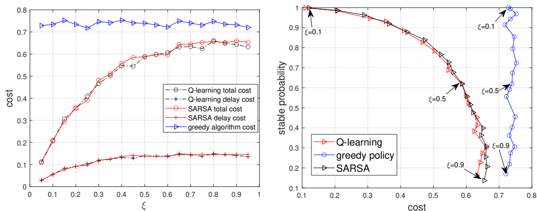
(a) Les coûts des différentes politiques.
