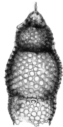
Eucyrtidium levisaltarix
