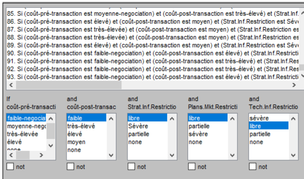
Figure 51. Interface de définition des règles d'inférences
