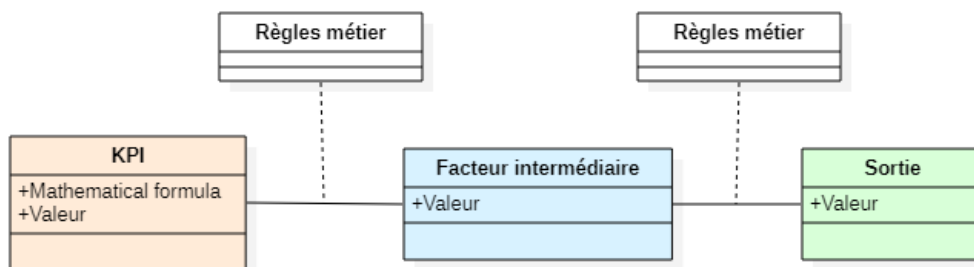
Figure 30. Diagramme de classes UML du modèle conceptuel
