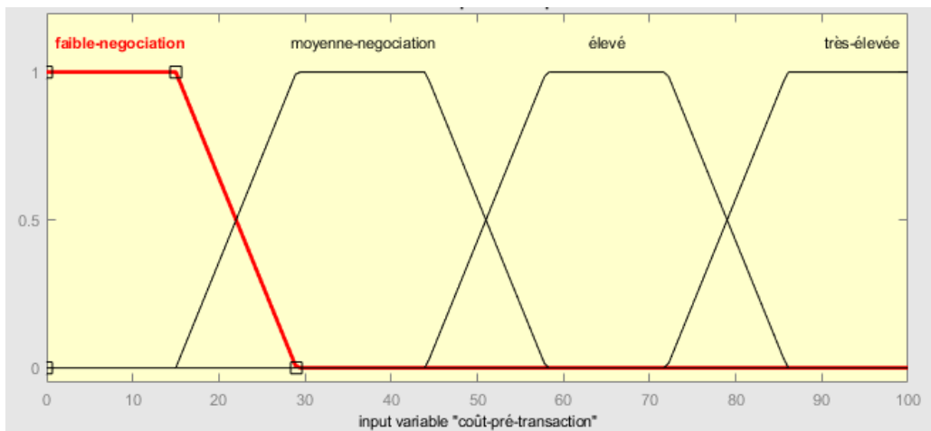
Fonctions d'appartenance pour la variable « coûts de pré-transaction »
