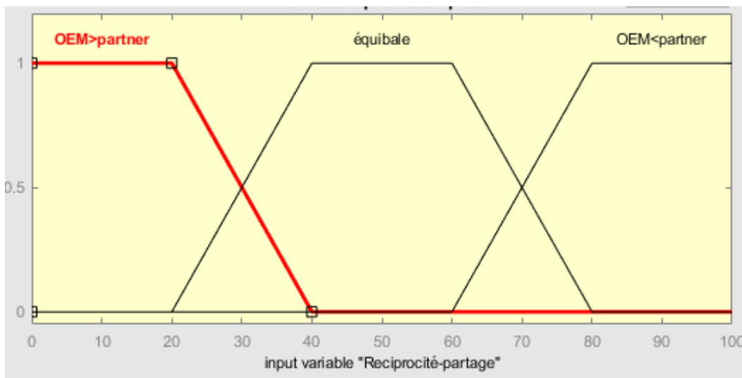
Fonctions d'appartenance pour la variable « Réciprocité dans le partage d'informations »
