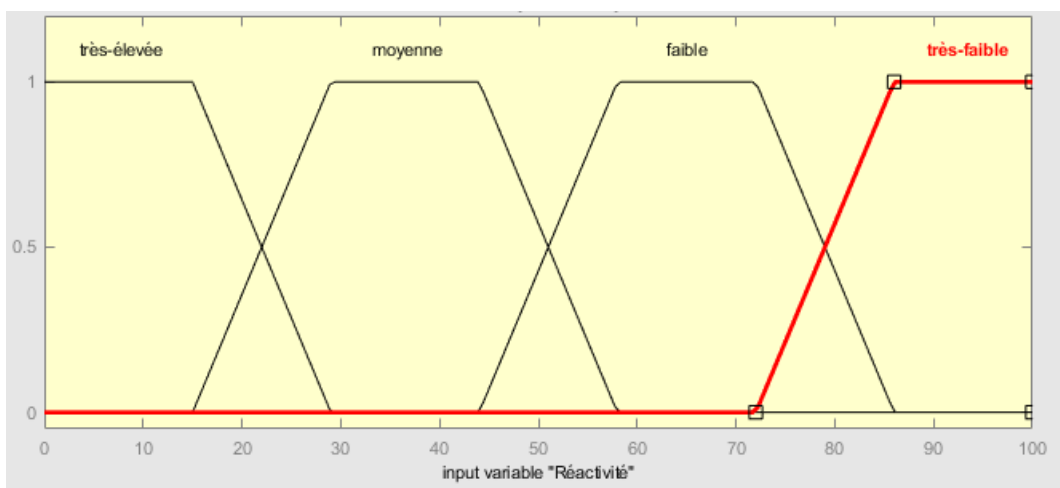
Fonctions d'appartenance pour la variable « Réactivité »
