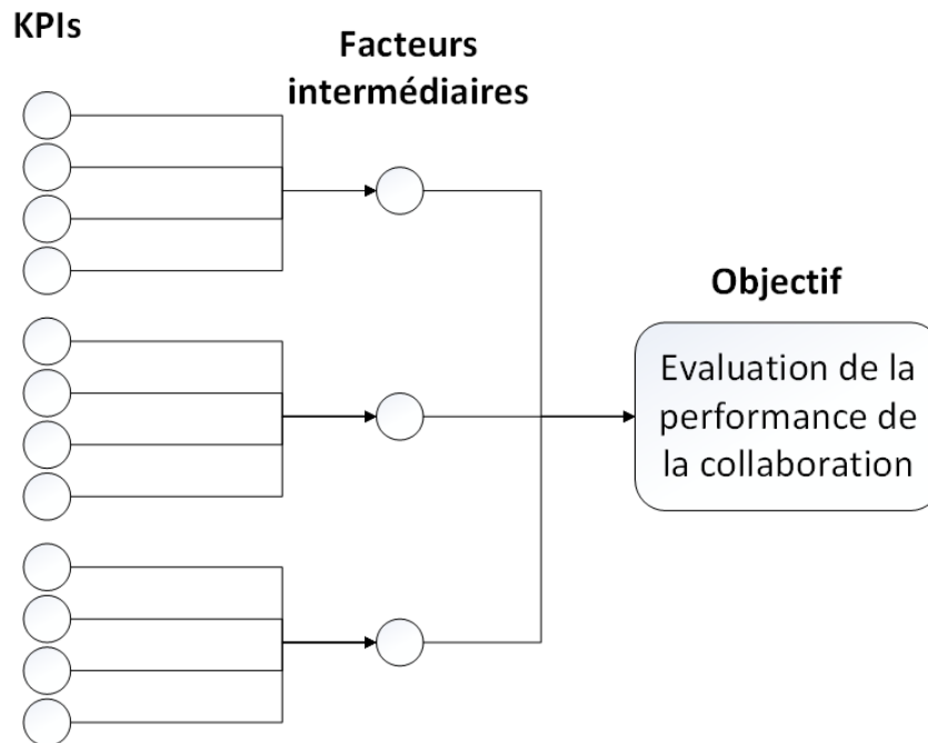
Figure 20. Framework conceptuel
