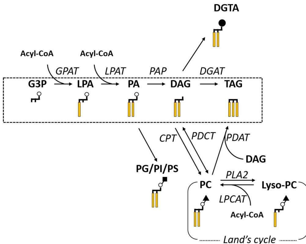
Figure 16 : Voies de biosynthèse des lipides extraplastidiaux. G3P, glycérol-3-Phosphate ; LPA, acide lyso-phosphatidique ; PA, acide phosphatidique ; PG, phosphatidylglycérol ; PI, phosphatidylinositol ; PC, phosphatidylcholine ; DAG, diacylglycérol ; TAG, triacylglycérol ; DGTA, diacylglycéryl-3-O-2'-(hydroxyméthyl)-(N,N,N-triméthyl)- \beta -alanine ; GPAT, glycérol-sn-3-phosphate acyltransférase ; LPAT, lysophosphatidate acyltransférase ; PAP, acide phosphatidique phosphatase ; DGAT, diacylglycérol acyltransférase ; CPT, DAG-cholinephosphotransférase ; PDCT, PC:DAG-cholinephosphotransférase ; PDAT, phospholipid:diacylglycérol acyltransférase ; LPCAT, acyl-CoA :lysophosphatidylcholine acyltransférase ; PLA2, phospholipase A2. Les rectangles jaunes représentent les chaînes d'acides gras. Les cercles blancs représentent les groupements phosphate. La voie de synthèse de novo dite de Kennedy est encadrée en pointillé tandis que la voie d'édition de la PC (Cycle de Lands) est représentée entre parenthèse.
