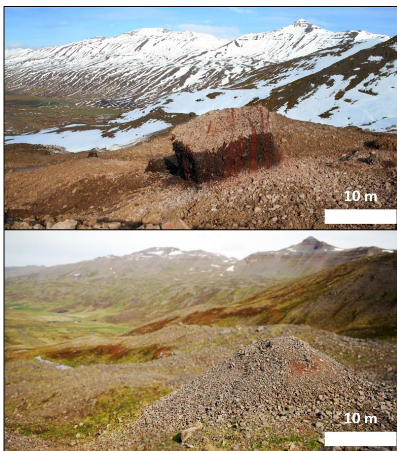
Figure 2 : dégradation d'un bloc de débris cimenté par la glace (Septembre 2012 ; Jón Kristinn Helgason), en un molard (Août 2022), en Islande.
