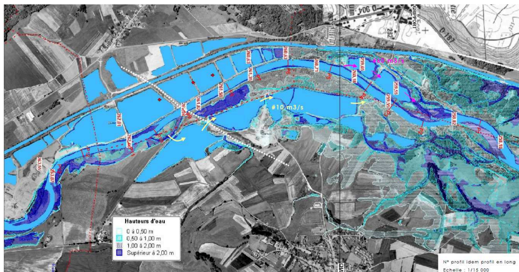
FIGURE 2.17 : Modélisation des surfaces inondées pour une crue décennale dans le secteur de Grippot (Atlas Sogreah)
