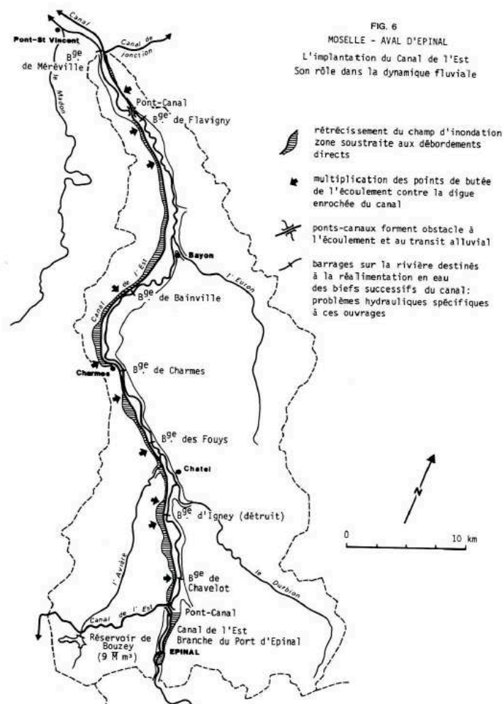
FIGURE 2.12 : Implantation du Canal de l'Est et son rôle dans la dynamique latérale de la Moselle, d'après Maire and Lasserre (1991)
