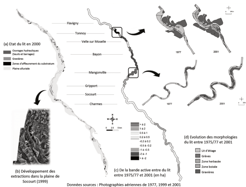
FIGURE 2.15 : Evolution de la dynamique de la Moselle à la suite de l'arrêt des extractions en lit mineur, d'après Beck and Corbonnois (2016)
