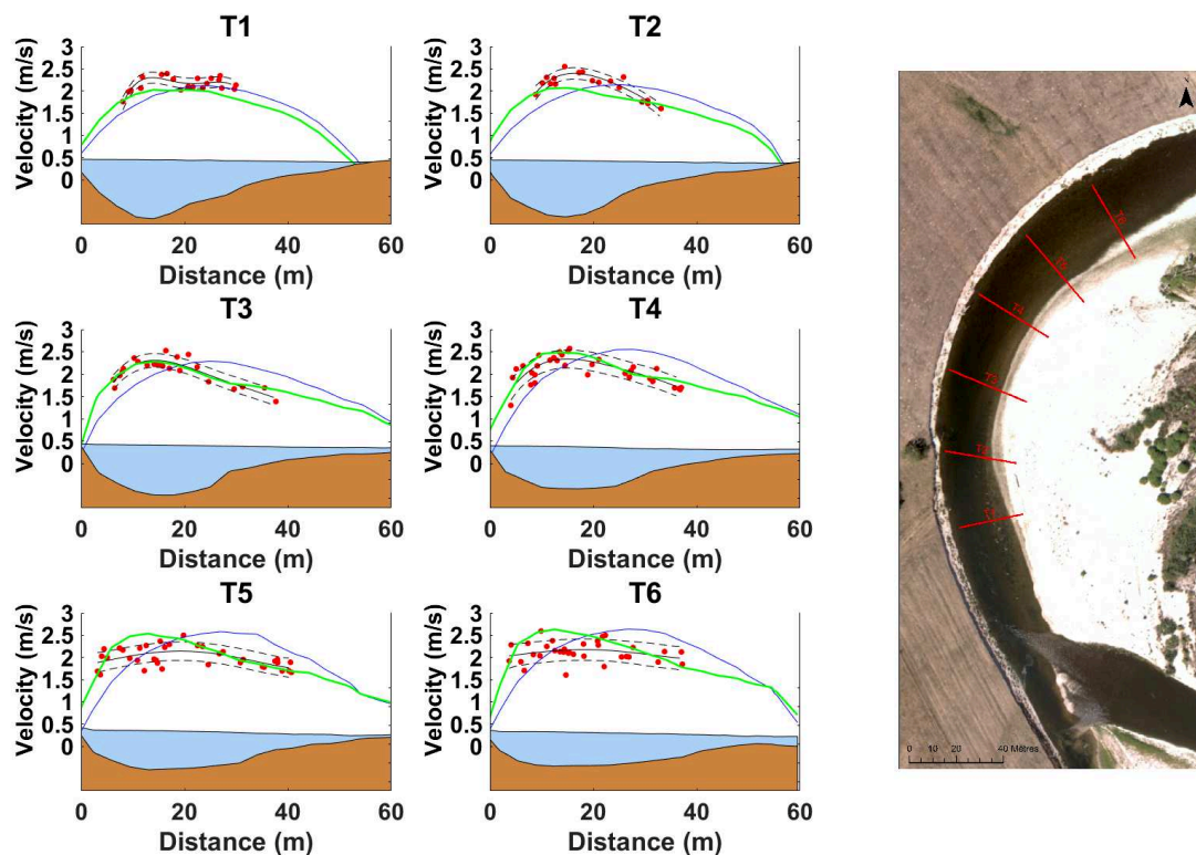
FIGURE 6.2 : Comparaison de profils de vitesse T_{n=1..6} mesur s par ADCP (points rouge) et mod lis s avec (lignes vertes) ou sans (lignes bleues) correction, le long du m andre de "la vache morte", lors d'une crue de p riode de retour d'un an ( Q = 180 m^3/s ).
