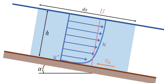
FIGURE 1.5 : Bilan des forces s'exerçant sur un volume d'eau en écoulement uniforme et répartition verticale des vitesses d'écoulement sur la colonne d'eau.
