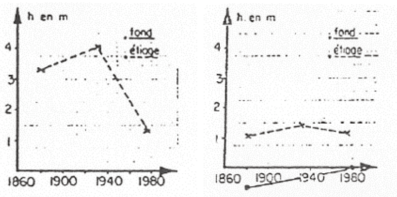
FIGURE 2.21 : Evolution du lit à Charmes (gauche) et Bainville (droite) (BCEOM, 1981)
