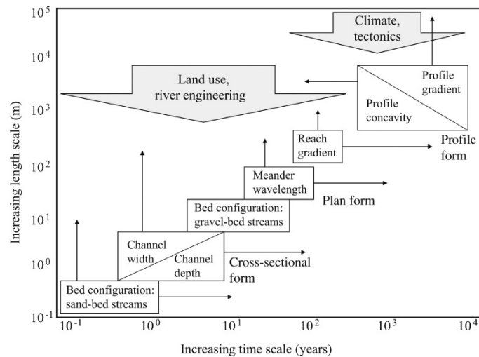
FIGURE 1.4 : Echelles temporelles et spatiales de l'ajustement des différentes composantes morphologiques du chenal. Les longueurs, indicatives, sont appliquées à un cours d'eau tempéré, d'après Knighton (1998).
