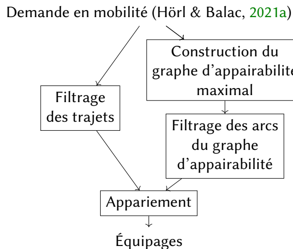
FIGURE 12.2 – Pipeline de données de MEPCEL (gros grain)
