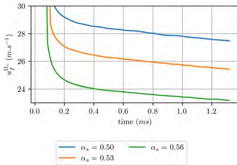
FIGURE 43 – Profils temporels des vitesses de réaction w_f^{\Omega_c} pour différentes compactions en tenant compte des réactions gazeuses via l'équilibre
