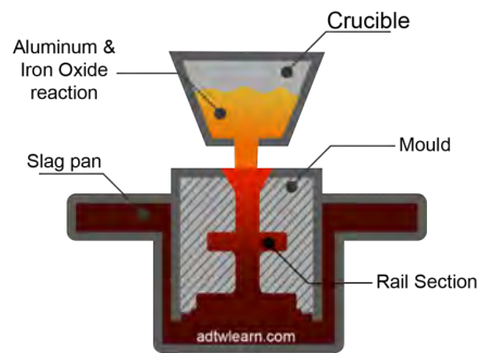
FIGURE 1.4 – Procédé de soudure thermitique pour application ferrovière 2
