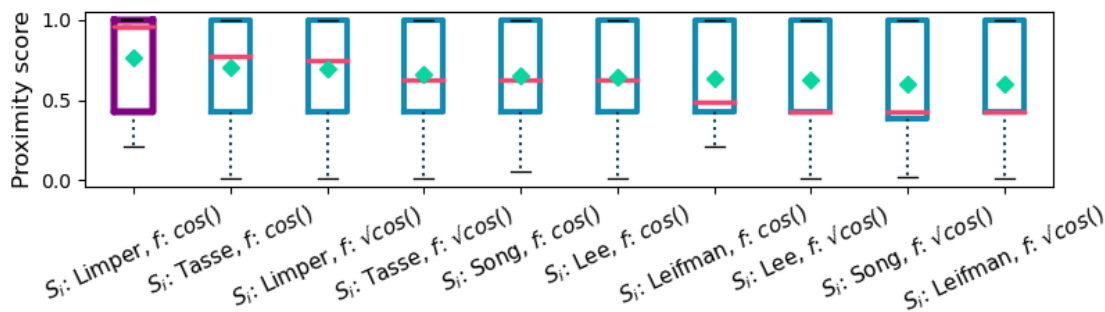
FIGURE IV.11. – Résultats quantitatifs de l'étape d'optimisation. Nous présentons les données statistiques des scores de proximité PS obtenus par les dix meilleures versions de la formule proposée IV.4, en spécifiant la méthode de saillance intrinsèque S_i et la fonction d'angle f utilisées dans le terme \mathbf{S}_a . Les scores de proximité sont calculés sur les 26 modèles de [Lavoué 18].
