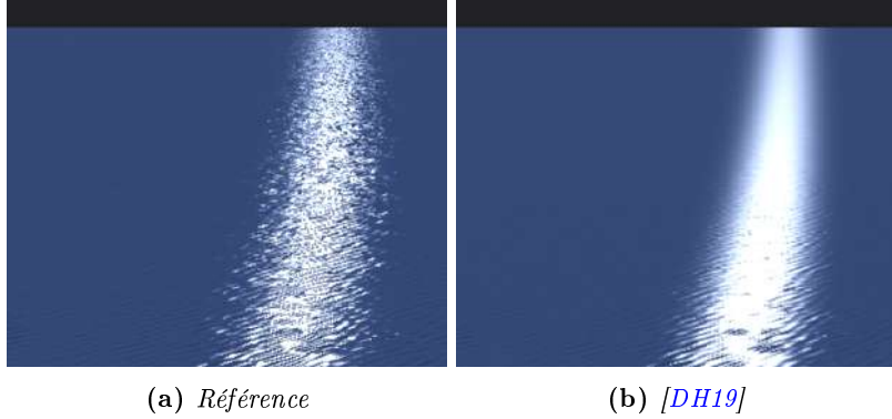
FIGURE 3.6 – Filtrage de vagues sur un plan horizontal. à gauche la référence, à droite la matrice de covariance est constante par niveau de filtrage ce qui provoque une perte de détails dans le résultat.
