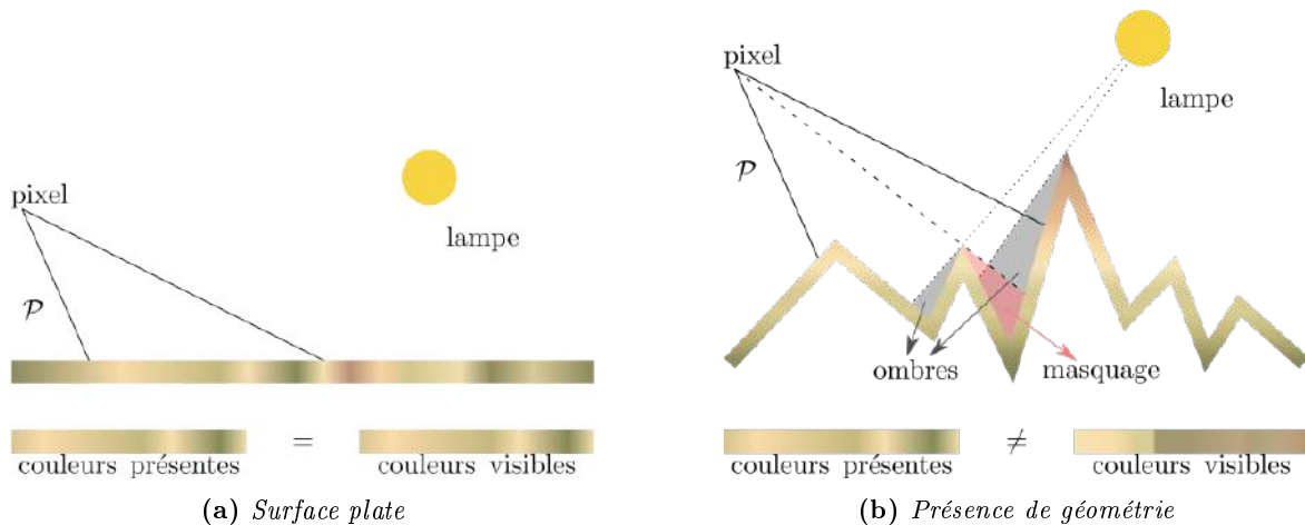
FIGURE 5.14 – L’ajout de géométrie nécessite de prendre en compte les ombres et les zones masquées pour déterminer la couleur moyenne dans l’empreinte d’un pixel.
