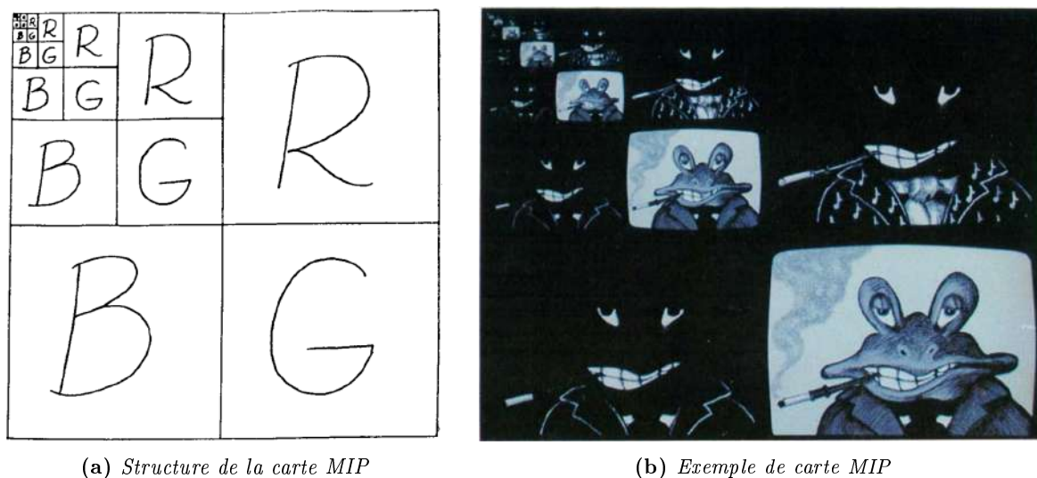
FIGURE 2.38 – Description de la carte MIP . Les trois canaux (Rouge, Vert, Bleu) de l'image d'entrée sont considérés et stockés indépendamment dans la carte. Images issues de [Wil83].
