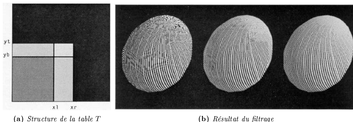
FIGURE 2.39 – Utilisation d'un tableau d'aire totale pour le filtrage. Dans la figure 2.39b, à gauche : sans filtrage, au milieu : filtrage par carte MIP, à droite : utilisation d'un tableau stockant les valeurs d'aire sous la courbe du signal. Images issues de [Cro84].
