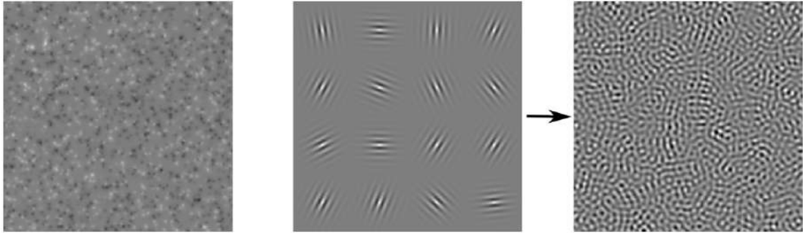
FIGURE 2.9 – À gauche, les positions aléatoires et leur pondération dans le domaine spatial. Au centre, le résultat avec quelques noyaux. À droite, le résultat final de la convolution. Image issue de [GSV + 14].
