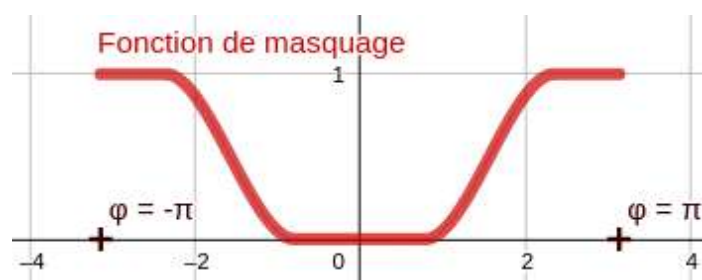
FIGURE 4.27 – Profil de la fonction de masquage \text{Smoothstep}(|\text{Atan2} \circ \mathbf{N}_{f,\theta}|) permettant de contrôler l'amplitude du bruit ajouté au sommet des crêtes.
