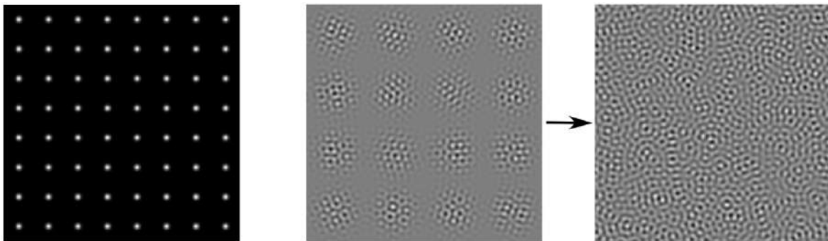
FIGURE 2.11 – À gauche, les positions sur une grille régulière dans le domaine spatial. Au centre, le résultat avec quelques noyaux. À droite, le résultat final de la convolution. Image issue de [GSV + 14].
