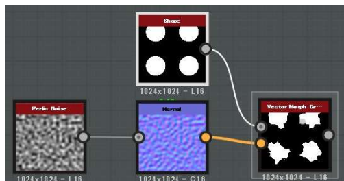
FIGURE 2.2 – Représentation en graphe de l’algorithme 1. Capture d’écran du logiciel Adobe Substance Designer.
