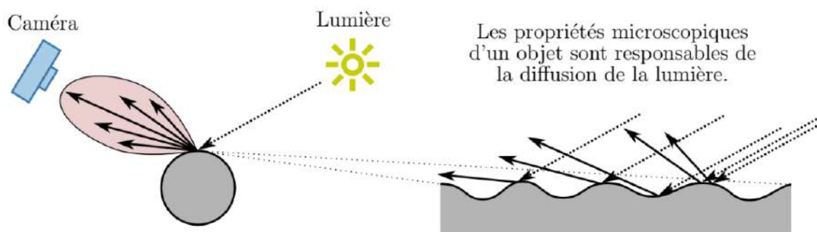
FIGURE 2.36 – La micro-géométrie de la surface (à droite) impacte l'interaction lumineuse et détermine sa couleur. Image issue de [Che19].
