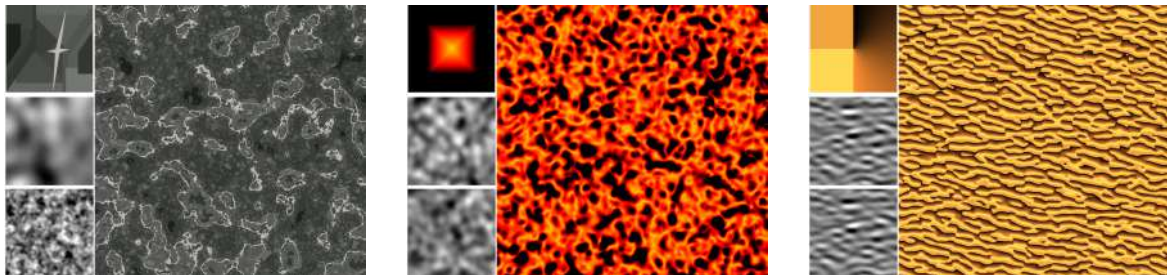
FIGURE 1.14 – Composition de bruits vectoriels par des cartes de couleurs bi-dimensionnelles. Pour chaque texture, la carte de couleurs (en haut à gauche) est appliquée sur les composantes du bruit vectoriel (au milieu et en bas à gauche) pour obtenir le résultat (à droite). Images issues de [GSDT22].
