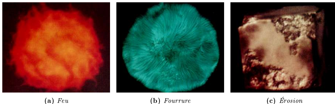
FIGURE 2.32 – Représentation de phénomènes par des hypertextures. Images issues de [PH89].
