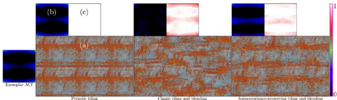
FIGURE 2.28 – À gauche, le pavage périodique préserve bien l'auto-covariance, mais fait apparaître des répétitions. Au centre, le pavage et mélange [HN18] crée de la variété par le tirage aléatoire des tuiles dans l'exemple. À droite, le tirage basé sur un échantillonnage préférentiel permet de mieux préserver l'auto-covariance de l'exemple. Pour chaque vue : (a) résultat de la synthèse, (b) auto-covariance du résultat, (c) similarité avec l'auto-covariance de l'exemple. Image issue de [LSD23].
