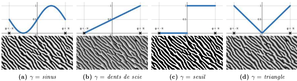
FIGURE 4.3 – Exemples de profils \gamma , tracés pour \varphi \in [-\pi, \pi] en haut, et les résultats de \gamma \circ \Phi(\mathbf{u}) correspondants (en bas).
