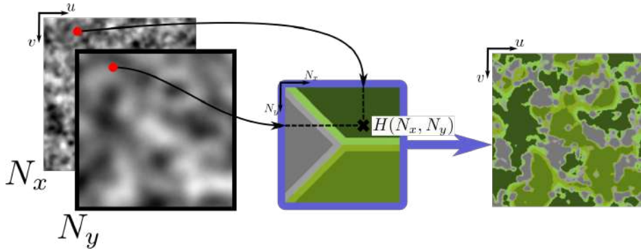
FIGURE 3.1 – Le modèle est défini par une composition. À gauche, le bruit vectoriel \mathbf{N} est représenté sous la forme de deux bruits scalaires pour des raisons de visibilité. Au centre, la fonction de transfert est stockée sous la forme d'une carte de couleurs. À droite, le résultat de la composition de \mathbf{N} par H .
