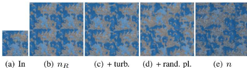
FIGURE 2.23 – Génération d'une texture à partir d'un exemple (a) présentant des éléments structurés. Une forte périodicité est observable dans le premier résultat (b). Celle-ci est cassée par l'ajout de turbulences (c), en ajoutant de l'aléatoire dans le positionnement des noyaux (d) et en introduisant une part d'aléatoire dans les phases. Image issue de [GSV + 14].
