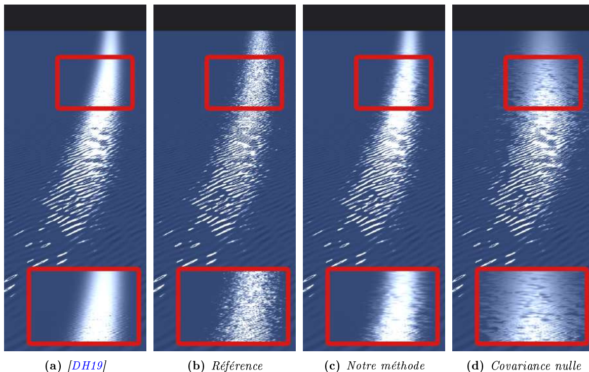
FIGURE 5.9 – Comparaison du filtrage de cartes de normales représentant des vagues sur l’océan. La précédente méthode utilisait des valeurs de variance constantes par niveau de détail (figure 5.9a). Notre méthode permet de retrouver les détails à mi-distance et de se rapprocher de la référence (figure 5.9c). En utilisant une covariance nulle (approximation faite pour les couleurs dans la section 3.4.1), les détails à mi-distance sont conservés, seul la forme du lobe globale est modifiée (figure 5.9d).
