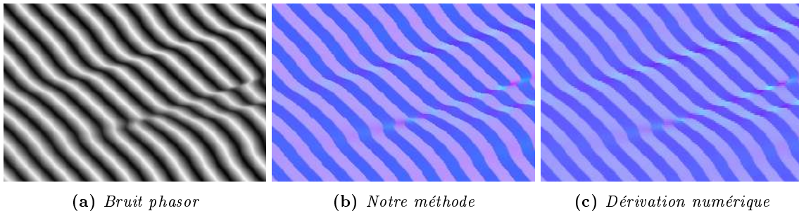
FIGURE 5.8 – Dérivation du bruit phasor 5.8a par notre méthode analytique 5.8b et par différences finies 5.8c. La méthode numérique est très dépendante de la résolution choisie, en particulier lors de forte variation dans les valeurs du champ scalaire.
