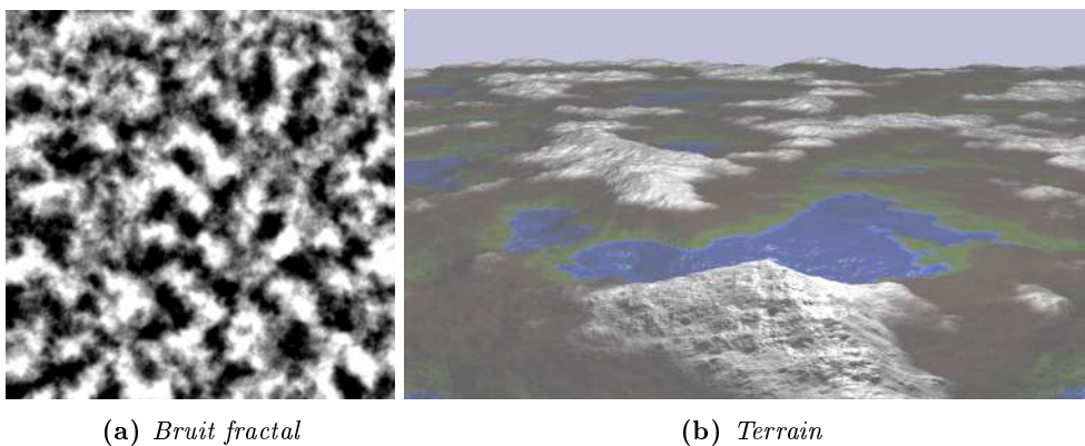
FIGURE 1.5 – Utilisation d'un bruit fractal pour générer un terrain procéduralement. Le champ scalaire 1.5a est utilisé comme information de hauteur pour créer le terrain 1.5b.
