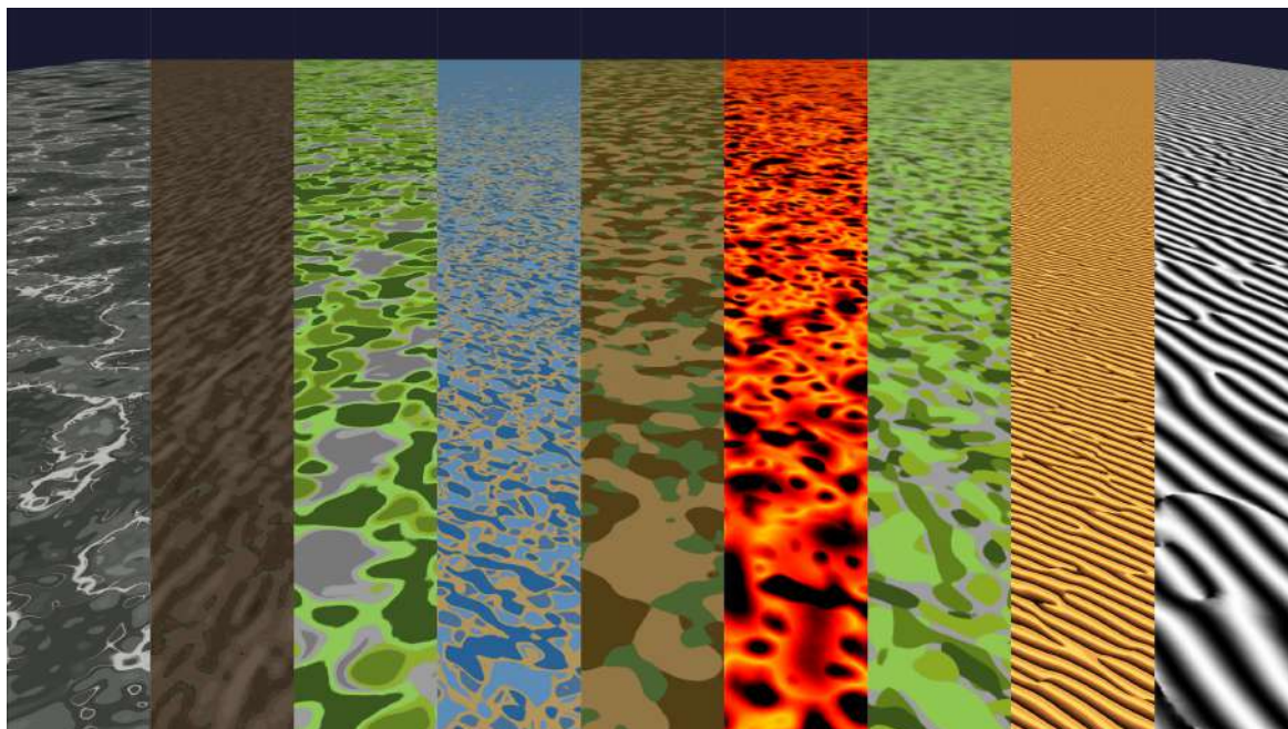
FIGURE 3.23 – Résultat du filtrage de différents motifs, appliqués sur un plan dans un espace 3D.
