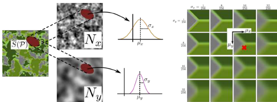
FIGURE 5.5 – L'estimation de la couleur moyenne dans une empreinte dans le résultat de la composition (à gauche) est fait en estimant la répartition des intensités des bruits dans cette empreinte (au centre). Ces répartitions sont utilisées dans une version pré-filtrée de la carte H (à droite).
