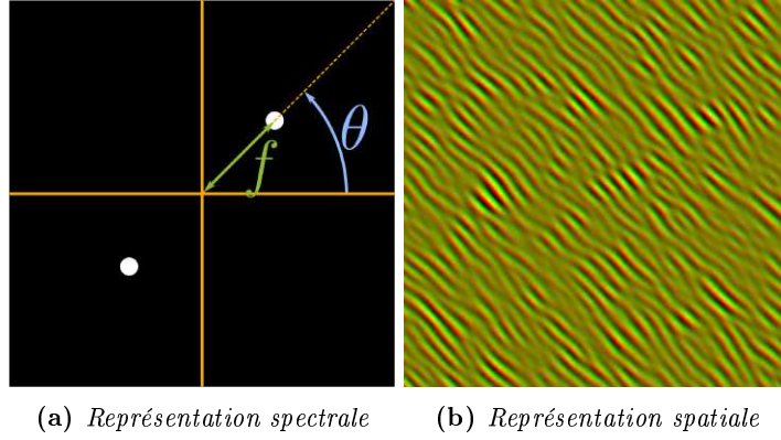
FIGURE 4.4 – Un bruit gaussien complexe et sa représentation spectrale dans le domaine de Fourier.
