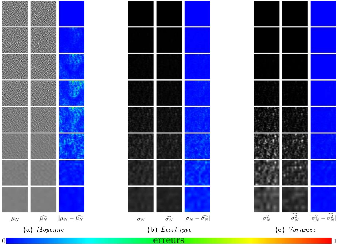
FIGURE 3.13 – Comparaison entre la référence et l'estimation des moyenne, écart-type et variance pour différents niveaux de filtrage. En ligne, les différents niveaux de filtrage en fonction de la taille de l'empreinte \mathbb{P} . De |\mathbb{P}| = 1 \times 1 , sur la première ligne, à |\mathbb{P}| = 128 \times 128 , sur la dernière ligne.
