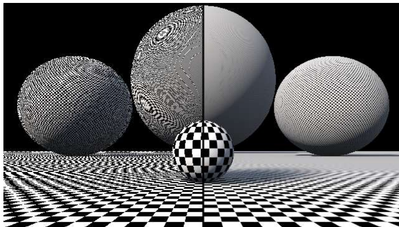
FIGURE 1.12 – Rendu d’une scène virtuelle avec filtrage (à droite) et sans filtrage (à gauche). En l’absence de filtrage, des artefacts visuels apparaissent sur le résultat. Image issue de iquilezles.org 2 .
