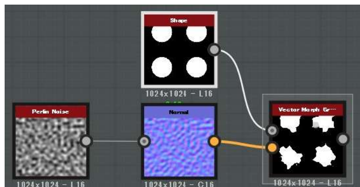
FIGURE 1.10 – Un graphe simple permettant d'obtenir une texture procédurale (à droite) à partir de deux champs scalaires (un bruit de Perlin à gauche et une forme en haut). Capture d'écran du logiciel Adobe Substance Designer.
