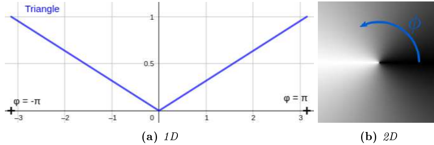
FIGURE 4.7 – Tracé de la fonction de profil \gamma en fonction de \varphi . À gauche en 1D et à droite selon la coordonnée angulaire de la carte représentant la fonction H .
