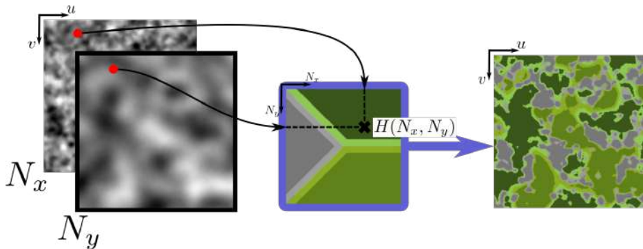
FIGURE 5.1 – Le modèle est défini par une composition. À gauche, le bruit vectoriel \mathbf{N} est représenté sous la forme de deux bruits scalaires pour des raisons de visibilité. Au centre, la fonction de transfert est stockée sous la forme d'une carte de couleurs. À droite, le résultat de la composition de \mathbf{N} par H .
