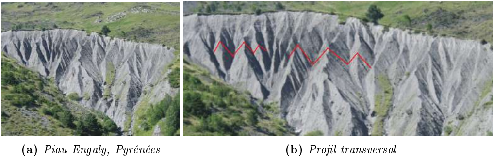
FIGURE 4.6 – Un profil transversal possible pour des ravines d’érosion dues à de l’écoulement d’eau.
