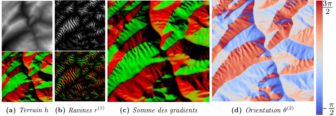
FIGURE 4.23 – Calcul du champ d'orientation \theta^{(2)} du second niveau de ravines en utilisant le gradient du terrain initial (figure 4.23a bas) et celui du premier niveau de ravines (figure 4.23b bas).
