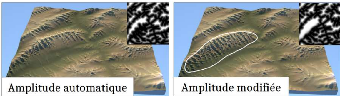
FIGURE 4.22 – Utilisation de l’amplitude calculée automatiquement (à gauche) et modification de cette amplitude afin d’ajouter plus de ravines sur une des pentes (entourée en blanc, à droite).
