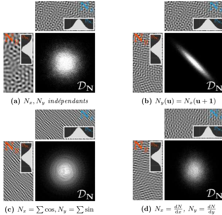
FIGURE 3.10 – Tracer réels de distributions conjointes de bruits gaussiens. Lorsque les bruits N_x et N_y sont parfaitement indépendants (figure 3.10a), la distribution conjointe est le produit des distributions marginales. Lorsque les bruits ne sont pas indépendants (figure 3.10b), la distribution conjointe est déformée en raison de la covariance entre les bruits. L'hypothèse d'indépendance peut être considérée à partir de la distribution conjointe également dans le cas où l'indépendance des bruits d'entrée n'est pas triviale à vérifier (figure 3.10c et 3.10d).
