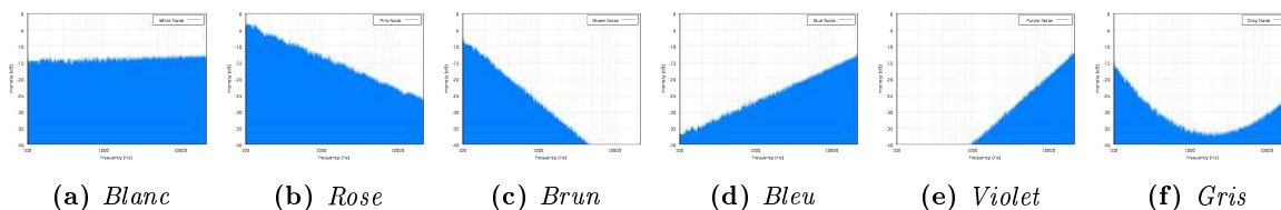
FIGURE 2.5 – Représentation spectrale de bruits colorés. Images issues de Wikipedia 1 .
