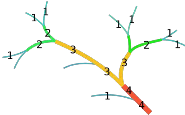
FIGURE 4.24 – Ordre des flux d'un réseau en fonction de leur position dans la hiérarchie. Les flux d'ordre 1 sont situés les plus en altitude. Image issue de Wikipedia 3 .
