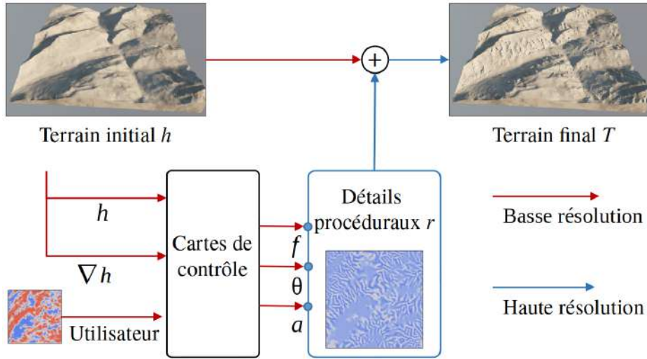
FIGURE 4.2 – Pipeline du modèle. Le terrain initial h (en haut à gauche) est augmenté pour obtenir le terrain final T (en haut à droite). Les détails d’augmentation r sont guidés par des cartes de contrôle dépendant du terrain initial, de son gradient et d’éventuelles cartes données par l’utilisateur.
