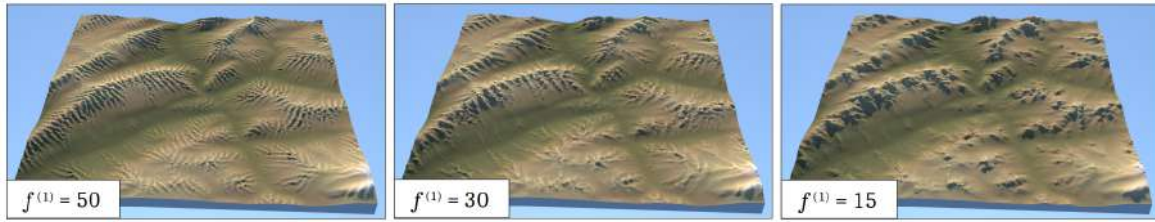
FIGURE 4.19 – Le choix de la valeur choisie pour la fréquence à une forte influence sur l'apparence du résultat. Cette valeur doit donc être cohérente avec la fréquence des éléments présents dans le terrain initial.
