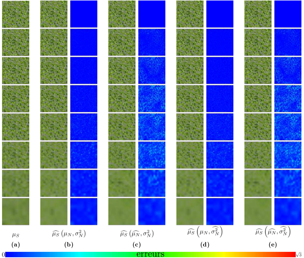
FIGURE 3.14 – Utilisation des estimateurs des statistiques pour faire le filtrage de la composition. Pour chaque étape d'approximation, nous mesurons la distance avec le filtrage de référence dans la colonne de droite. En ligne, les différents niveaux de filtrage en fonction de la taille de l'empreinte \mathbb{P} . De |\mathbb{P}| = 1 \times 1 , sur la première ligne, à |\mathbb{P}| = 128 \times 128 , sur la dernière ligne.
