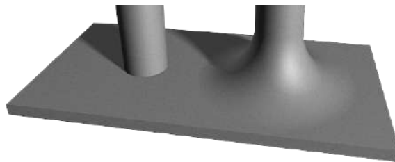
FIGURE 4.9 – Jonction entre un plan et un cylindre, sans congé de raccordement (à gauche) et avec un congé de raccordement (à droite). Image issue de Wikipedia 2 .
