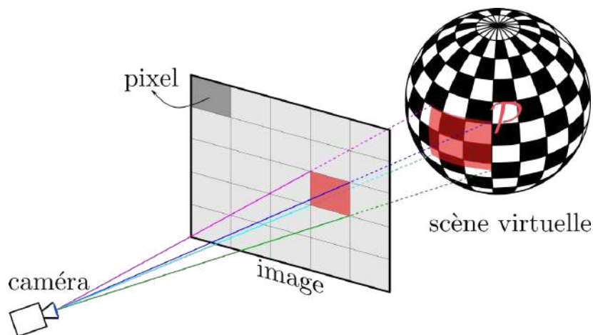
FIGURE 2.4 – Projection de l'empreinte \mathcal{P} d'un pixel de l'écran dans la scène virtuelle. Le pixel surligné en rouge dans l'image doit prendre la couleur moyenne des éléments de la scène virtuelle présents dans son empreinte \mathcal{P} .
