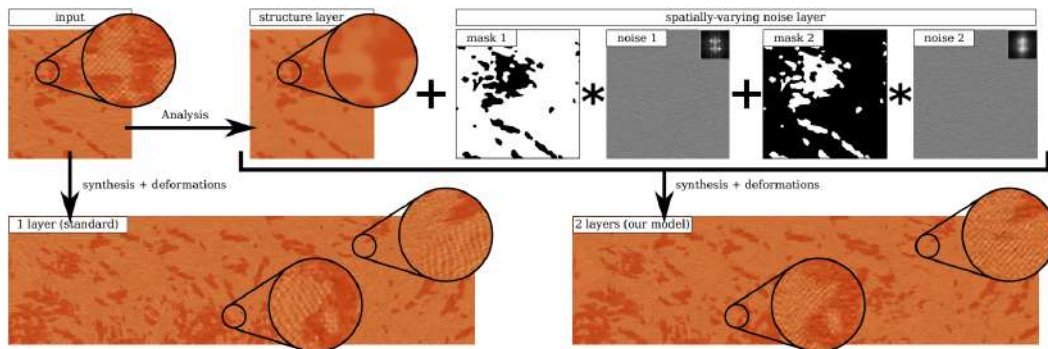
FIGURE 2.20 – Décomposition d'un exemple d'entrée (en haut à gauche) en plusieurs couches. Cette décomposition permet d'appliquer des déformations sans observer d'étirement des micro-détails (en bas). Image issue de [GSDC17].
