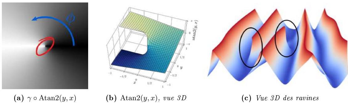
FIGURE 4.12 – La fonction Atan2 présente une singularité au point (0, 0) qui provoque l'apparition de variations brusques aux intersections des ravines générées.
