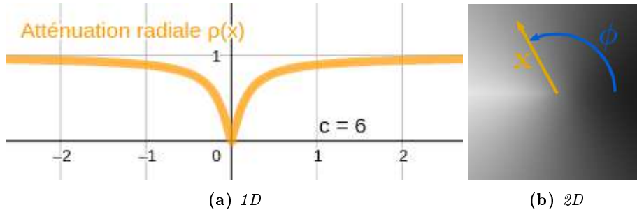
FIGURE 4.13 – Tracer de la fonction de profil \rho en fonction de \mathbf{x} . À gauche en 1D et à droite selon la coordonnée radiale de la carte représentant la fonction H .
