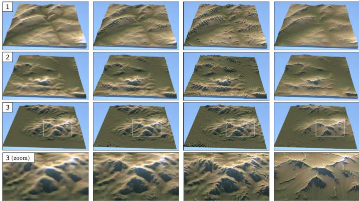
(a) Terrain initial (b) Bruit fBm (c) Notre augmentation (d) Simulation
