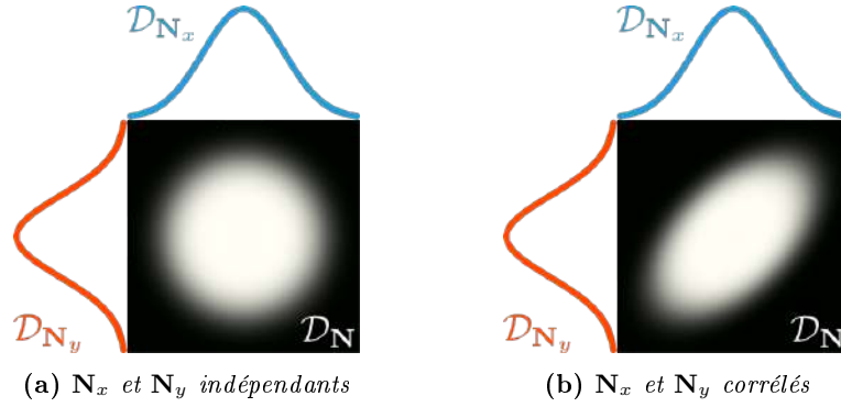
FIGURE 3.9 – Tracer théoriques de distributions conjointes de couples de variables aléatoires. Les distributions marginales sont représentées en haut (bleu) et à gauche (rouge) de la distribution conjointe. Dans le cas où les variables sont indépendantes (figure 3.9a) la distribution conjointe est le produit des distributions marginales. Dans le cas contraire (figure 3.9b), la distribution conjointe est déformée.
