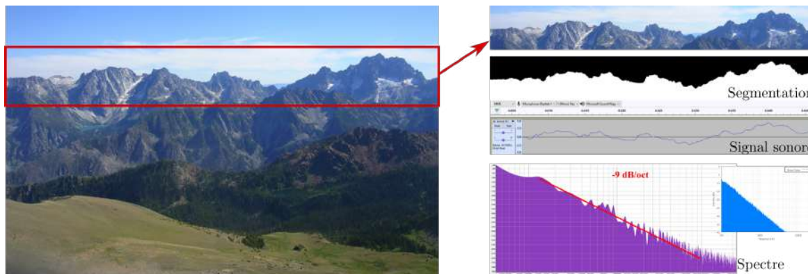
FIGURE 4.26 – Comparaison spectrale entre les crêtes d'une montagne réelle et un bruit brun. Image issue de iquilezles.org 4 .
