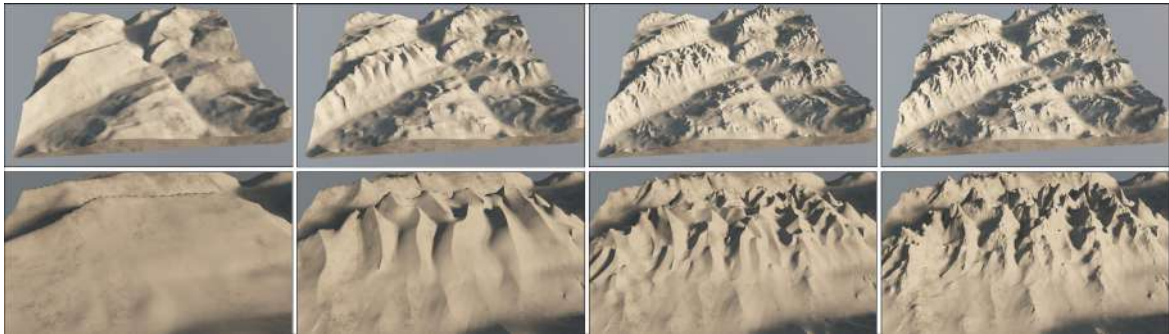
FIGURE 4.29 – Résultat final de notre augmentation de terrain. La première ligne montre le terrain dans sa globalité alors que la seconde montre une vue de plus près. De gauche à droite, les vignettes montrent : le terrain initial, l’ajout du premier niveau de ravines, l’ajout du second niveau de ravines et l’ajout du bruit au sommet de crêtes.
