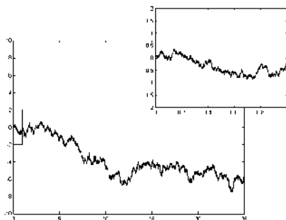
FIGURE 2.29 – Réalisation d'un processus de Wiener à une dimension. L'encadré à droite montre un zoom sur le processus pour des valeurs entre 0 et 1. Image issue de Wikipedia 3 .
