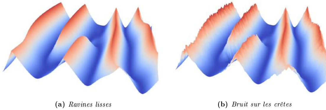
FIGURE 4.28 – Comparaison des crêtes du premier niveau de ravines sans (gauche) et avec (droite) le bruit C . L’ajout de ce bruit permet de casser le côté lisse des lignes de crêtes et d’ajouter du réalisme.
