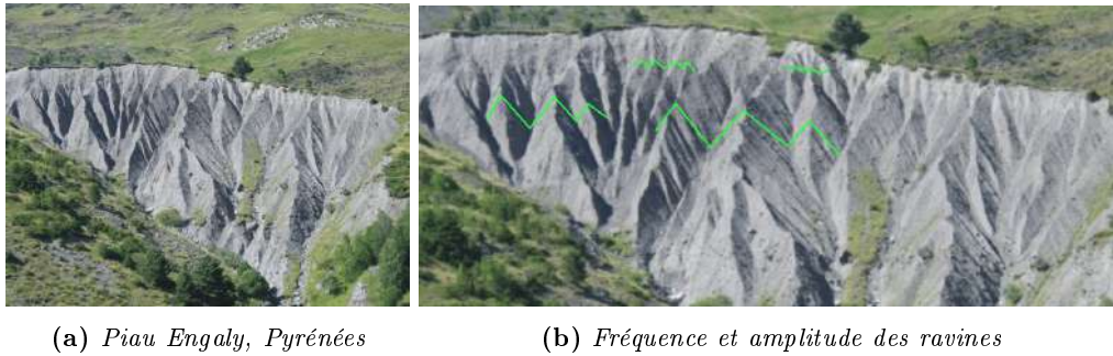
FIGURE 4.20 – Observation de la fréquence de ravines sur un terrain réel.
