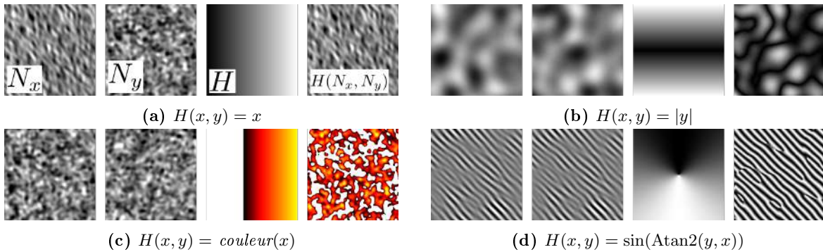
FIGURE 3.2 – Reproduction de résultats déjà existant par une composition avec une carte de couleurs à deux dimensions.
