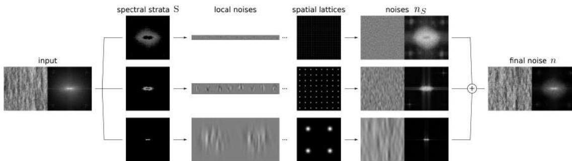
FIGURE 2.17 – Décomposition du spectre d'un exemple d'entrée (à gauche) pour reproduire ses caractéristiques dans la texture de sortie (à droite). Image issue de [GSV + 14].
