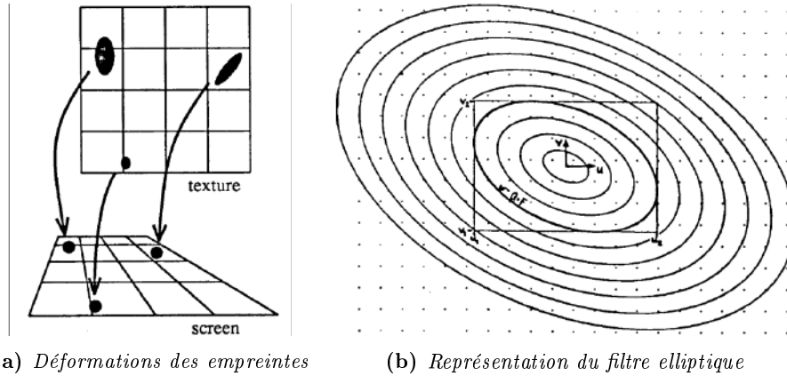
FIGURE 2.40 – Représentation elliptique des empreintes de pixel. Figure 2.40a la texture observée dans l'espace écran (en bas) est déformée par rapport à l'espace texture (en haut) et des empreintes qui apparaissent rondes sont en réalité elliptiques. Figure 2.40b, Représentation du filtre Q . Cette présentation permet une meilleure estimation de la moyenne que ne le ferait le calcul sur la boîte englobante (rectangle sur l'image). Images issues de [Hec89].
