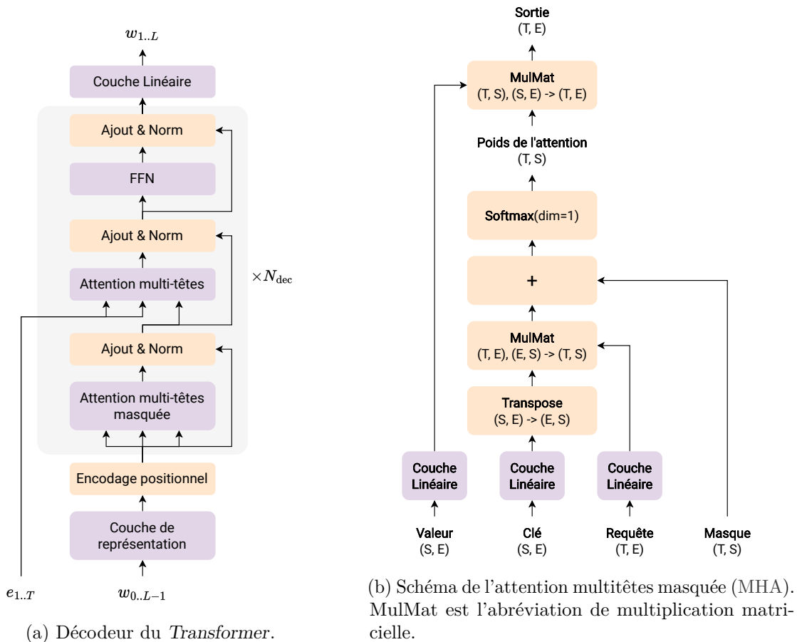
FIGURE 3.4 – Schéma du décodeur de type Transformer et du module MHA.
