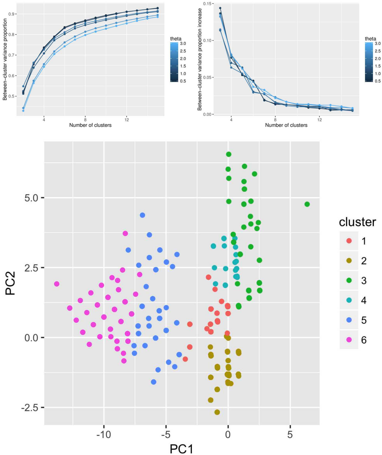
FIGURE 81: Identification de régimes d'interactions endogènes par classification non-supervisée. ( Haut Gauche ) Variance inter-cluster comme fonction du nombre de clusters. ( Haut Droite ) Dérivée de la variance inter-cluster. ( Bas ) Features dans un plan principal (81% de variance expliquée par les deux premières composantes).
