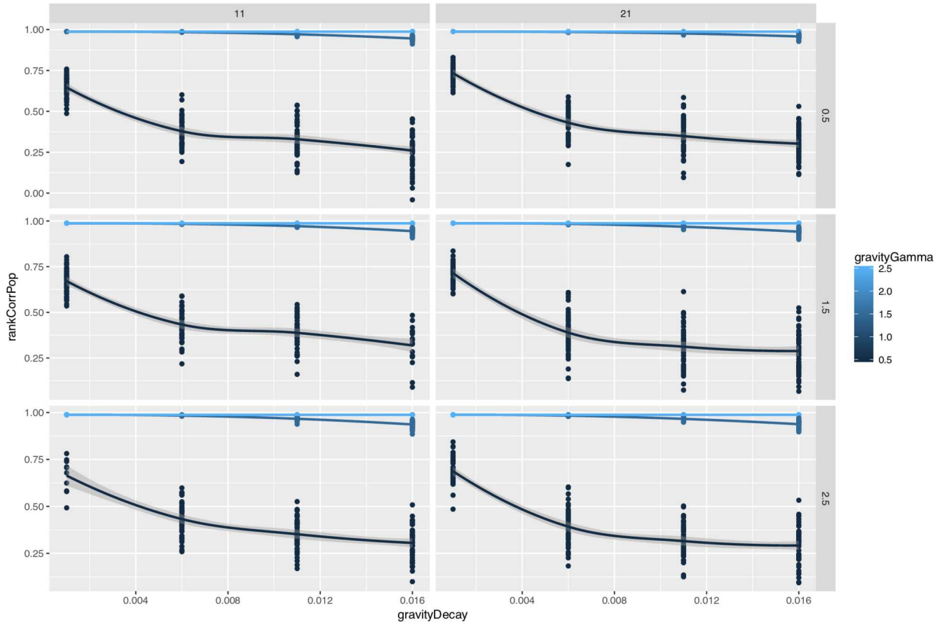
FIGURE 93: Corrélations de rang pour la population. Nous donnons \rho_r[\mu_i] en fonction de d_G , pour \gamma_N variable (couleur), \theta_N variable (colonnes) et \gamma_N variable (lignes).
