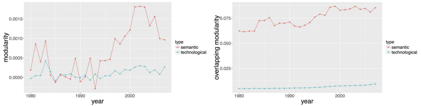
FIGURE 149: Evolution temporelle des modularités sémantique et technologique du réseau de citation. (Gauche) Modularité dirigée simple, calculée avec les classes principales des brevets (classe technologique principale et classe sémantique avec la plus grande probabilité). (Droite) Modularité multi-classes, calculée selon [NICOSIA et al., 2009].
