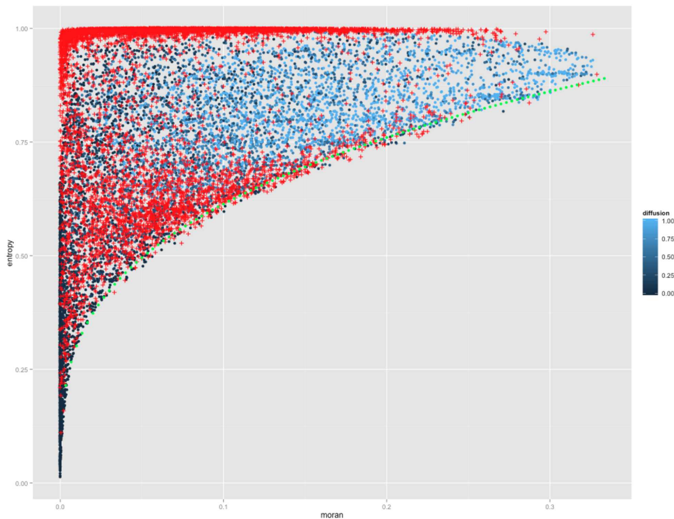
FIGURE 40 : Exploration par PSE. Scatterplot de l'entropie \mathcal{E} en fonction de l'indice de Moran I . Les points bleus, dont le niveau de couleur donne la valeur du paramètre de diffusion \beta , sont obtenus par criblage LHS, tandis que les points rouges sont obtenus par l'algorithme PSE. La ligne pointillée verte donne la borne inférieur faisable (qui peut être qualifiée telle quelle grâce aux propriétés de PSE), qu'il n'est pas possible d'obtenir de manière simple analytiquement. Sa forme en loi d'échelle suggère des directions de recherche, par exemple par la détermination de bornes morphologiques pour des distributions de population, et les relations fonctionnelles entre ces bornes.
