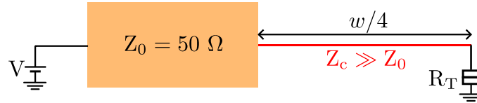
Figure E.2: Schéma d'un convertisseur de photons en électrons. Pour détecter les photons de longueur d'onde w , un résonateur w/4 , représenté en rouge, est terminé d'un côté par une jonction tunnel supraconductrice polarisée en tension. L'impédance caractéristique Z_c du résonateur est comparable au quantum de la résistance. Le résonateur est couplé galvaniquement au reste du circuit par une ligne de transmission d'impédance caractéristique 50 \Omega .
