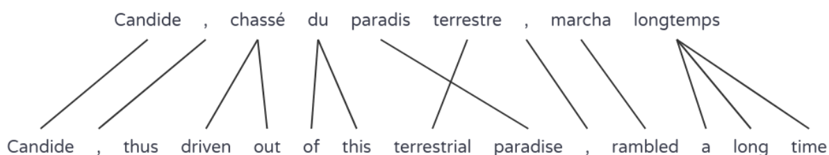
FIGURE 9 – Exemple d'alignement
