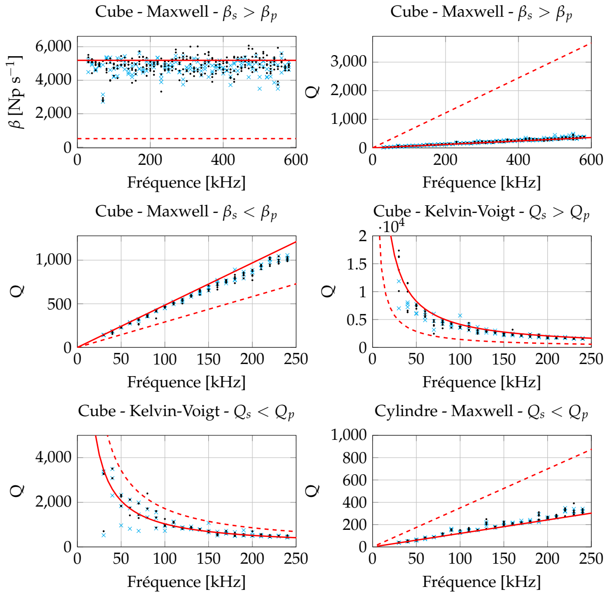
Figure VII.5: Détermination de l'atténuation \beta et du facteur qualité Q en fonction de la fréquence sur des simulations numériques à travers un cube de 7 cm de côté ou un cylindre de 9 cm de haut pour 5 cm de diamètre qui suivent des lois viscoélastiques de Maxwell ou de Kelvin-Voigt. [---] \beta_p ou Q_p analytique. [—] \beta_s ou Q_s analytique. [.] Récepteurs R2 et R3 situés à la surface et enregistrant dans les 3 composantes u_x , u_y et u_z . [x] Récepteur R1 situé à l'intérieur et enregistrant dans les 3 composantes u_x , u_y et u_z .
