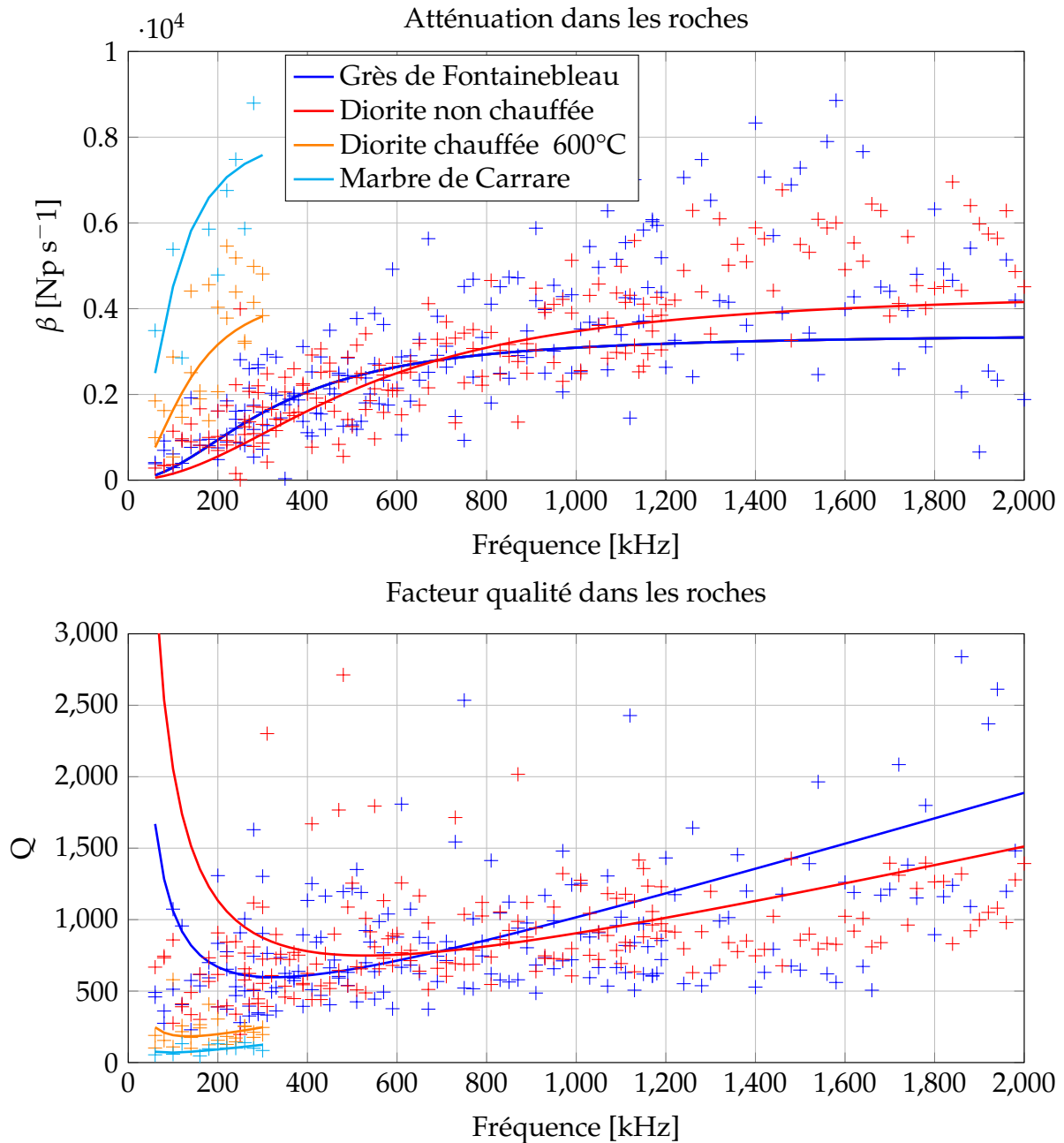
Figure VII.7: Détermination de l'atténuation et du facteur qualité Q sur des roches. [ + ] atténuation pour une fréquence centrale donnée. [ — ] Modèle viscoélastique de Zener pour des paramètres donnés en Table IV.9 .
