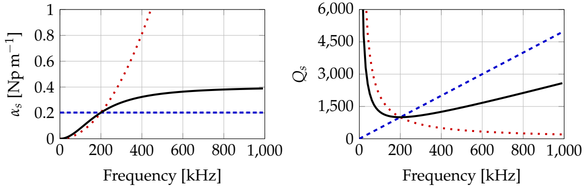
Figure VII.2: (gauche) Atténuation et (droite) facteur qualité des ondes S en fonction de la fréquence pour respectivement un modèle viscoélastique de [---] Maxwell avec \eta_\mu = 20.65 MPa s, [· · ·] Kelvin-Voigt avec \eta_\mu = 20.65 Pa s et [—] Zener avec \tau_c = 796.57 ns et \tau_\sigma = 794.98 ns. Ici, le paramètre élastique \mu est de 25.95 GPa.
