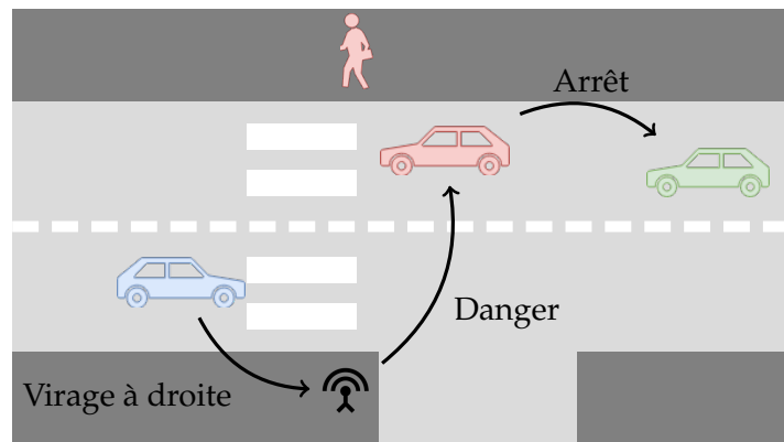
FIGURE 2.2 – Exemple de situation routière où des échanges entre des véhicules et l'infrastructure améliorent leur connaissance de la route.
