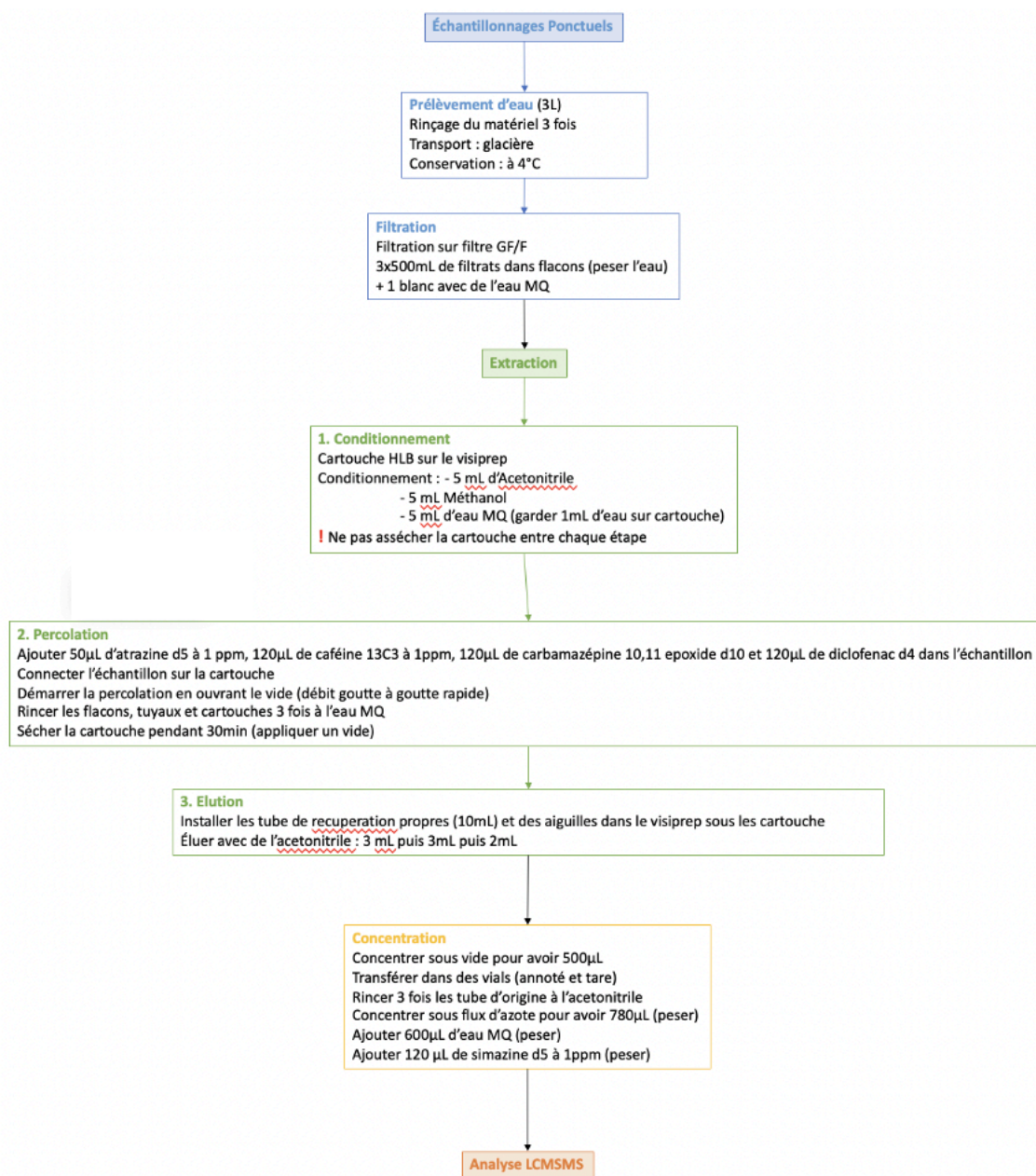
Annexe 1.9: Protocole utilisé pour les extractions des échantillons ponctuels.
