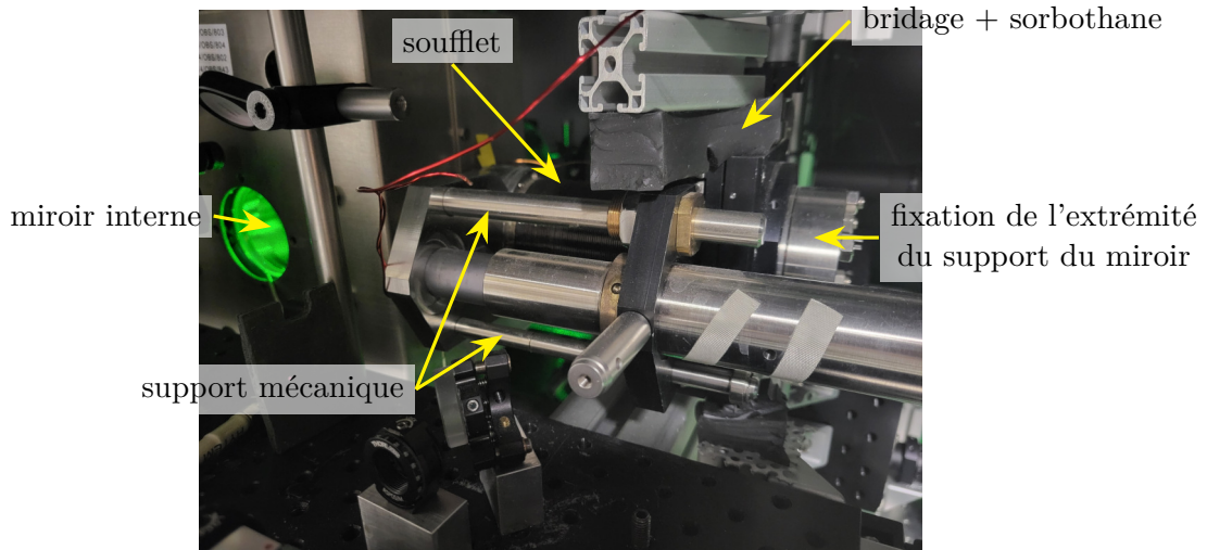
FIGURE IV.16 – Photographie du système mécanique de support du miroir interne.
