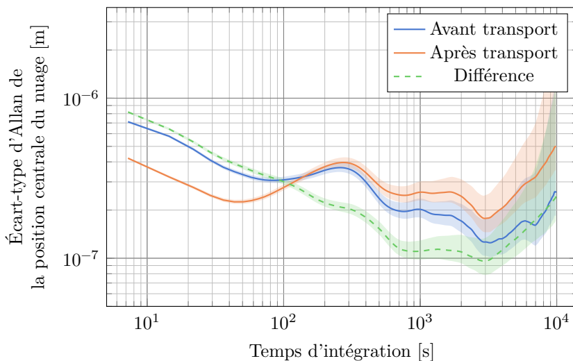
FIGURE V.1 – Stabilité de la distance de transport \Delta z . En bleu et en orange sont représentées les stabilités respectivement des positions z_i initiale et z_f à l'issue du transport. En vert est représenté l'écart-type d'Allan de la différence entre les deux positions z_f - z_i .
