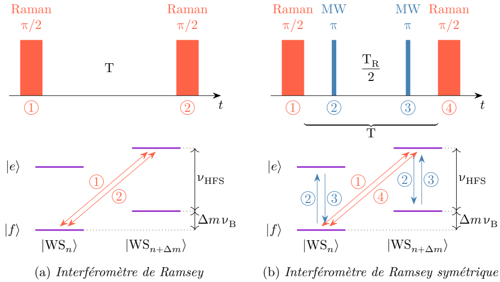
FIGURE II.9 – Séquences interférométriques de Ramsey à gauche et de Ramsey symétrisé par l'ajout d'impulsion \pi micro-onde à droite.
