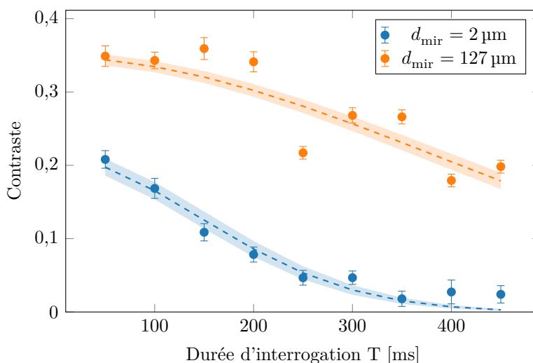
FIGURE IV.2 – Amortissement du contraste interférométrique avec la durée d'interrogation. Mesure pour une puissance du laser de confinement P_{\text{IR}} = 0,6 \text{ W} . Les courbes en pointillés représentent l'ajustement du contraste par l'équation (IV.3). On en déduit la valeur des inhomogénéités représentées figure IV.3.
