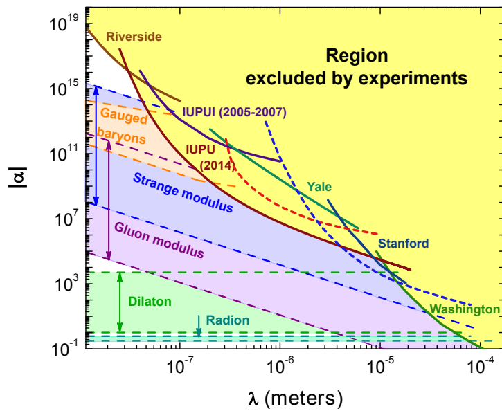
FIGURE I.2 – Diagramme d'exclusion ( \lambda; \alpha ) centré autour des portées microscopiques. Figure adaptée de [Che16]. Différentes prédictions théoriques sont représentées par des zones colorées. Les courbes en pointillés représentent les contraintes visées au début de l'expérience ForcaG il y a dix ans [Mes11; Sol16b], en soustrayant aux mesures de force un modèle théorique de la force de Casimir-Polder précis à quelques pour cent (en bleu) ou réalisant une mesure différentielle entre isotopes du rubidium (en rouge).
