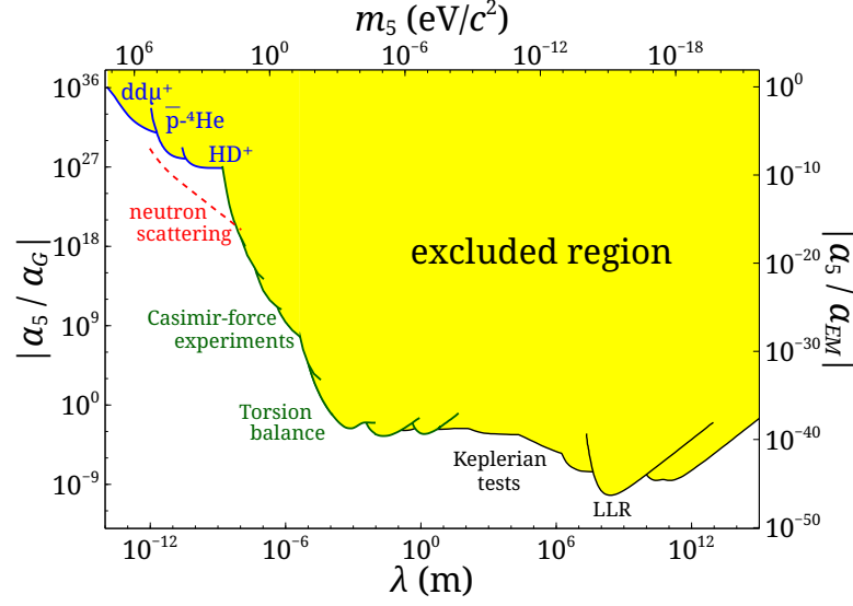
FIGURE I.1 – Diagramme d'exclusion (\lambda; \alpha) , des distances astrométriques aux interactions entre particules. Figure extraite de [SUK14].
