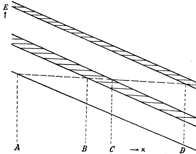
FIGURE II.2 – Figure extraite de l'article original de Zener [Zen34]. Les bandes d'énergie sont localement inclinées sous l'effet du potentiel -Fz . Les zones hachurées représentent les gaps en énergie entre deux bandes.
