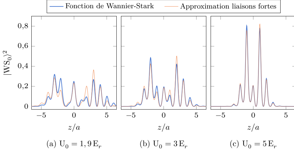
FIGURE II.3 – Fonctions d’onde de Wannier-Stark, pour trois profondeurs de réseau différentes. Les fonctions d’onde présentent des maxima locaux au niveau des puits de potentiel du réseau, et sont d’autant moins étalées que le réseau est profond. Le calcul a été effectué soit complètement (éq. (II.24) et (II.25)), soit dans l’approximation des liaisons fortes (éq. (II.27)).
