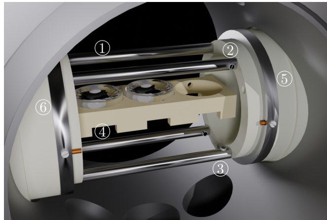
(a) Rendu 3D de la chambre à vide supérieure, avec le support céramique des miroirs (en jaune), entouré de six électrodes métalliques.
