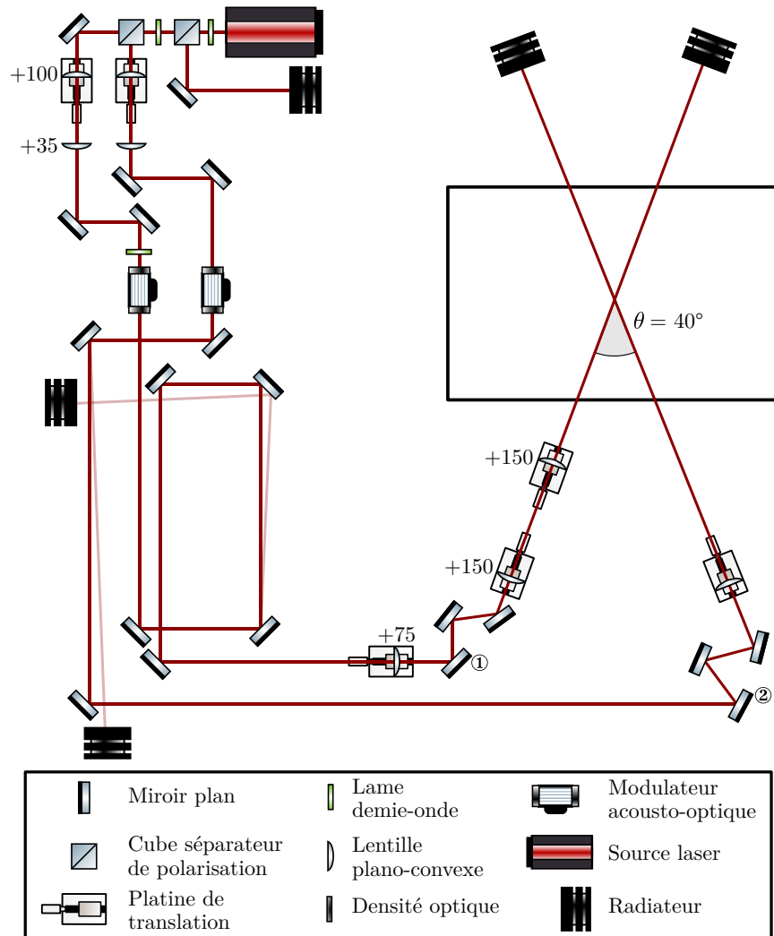
FIGURE III.3 – Schéma du banc optique du piège dipolaire évaporatif.
