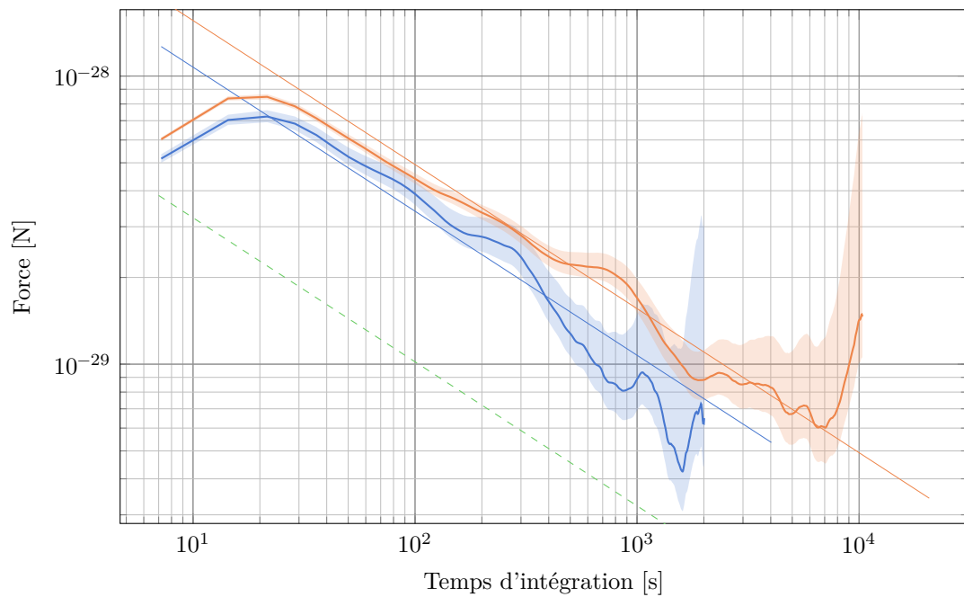
FIGURE IV.22 – Écart-types d'Allan de mesures de force à quelques centaines de micromètres du miroir, avec l'ajustement en 1/\sqrt{\tau} correspondant. Les courbes représentent, en bleu, des mesures avec T = 150 ms et avec correction des vibrations, et, en orange, des mesures avec T = 100 ms et sans corrections des vibrations. La courbe bleue présente une sensibilité de 340 \times 10^{-30} N à 1 s et la courbe orange se moyenne sur les 20 000 s de mesure jusqu'à 4 \times 10^{-30} N. En vert est représentée la limite quantique estimée dans la situation actuelle de l'expérience.
