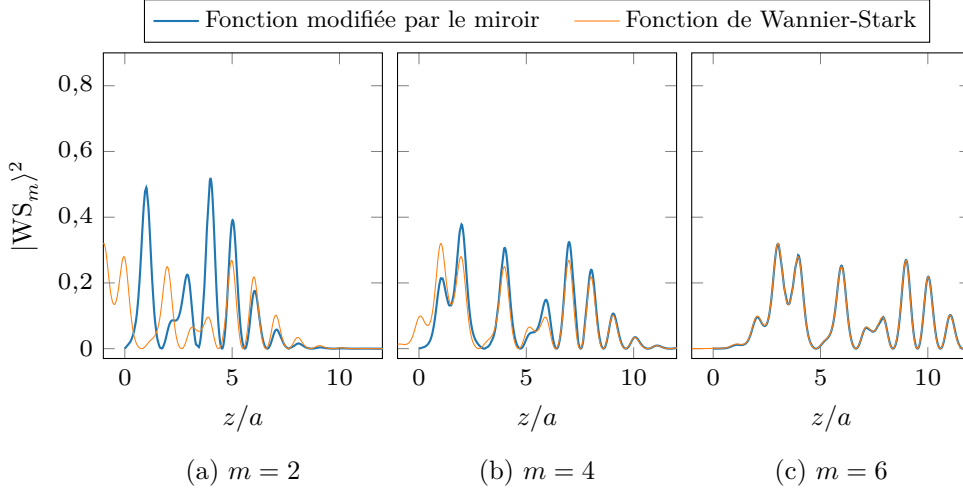
FIGURE II.14 – Fonctions d’onde de Wannier-Stark modifiées par le mur de potentiel de la surface du miroir et la fonction d’onde non modifiée correspondante, pour une profondeur de réseau de U_0 = 1,9 E_r .
