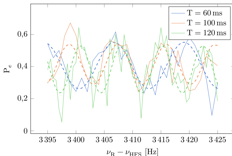
FIGURE V.7 – Franges interférométriques pour des durées d’interrogation T différentes, avec l’ajustement sinusoïdal correspondant en pointillés. La phase nulle est située aux alentours de 3409 Hz. Les franges sont décalées d’une fraction d’interfrange par rapport à la fréquence de phase nulle à cause du déplacement lumineux différentiel des faisceaux Raman \delta_{AC} .
