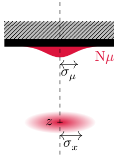
FIGURE V.14 – Schéma de la modélisation de la distribution de moments dipolaires
