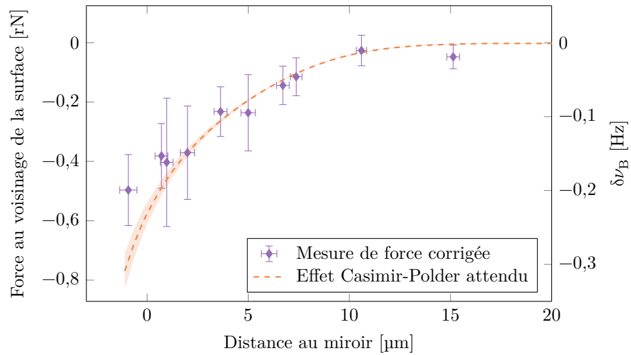
FIGURE V.18 – Corrections des mesures des forces par le modèle de force électrostatique. Les incertitudes sur les mesures de force prennent en compte l'incertitude du modèle issue de l'ajustement. La zone d'incertitude sur l'effet Casimir est liée à l'incertitude sur l'épaisseur du nuage.
