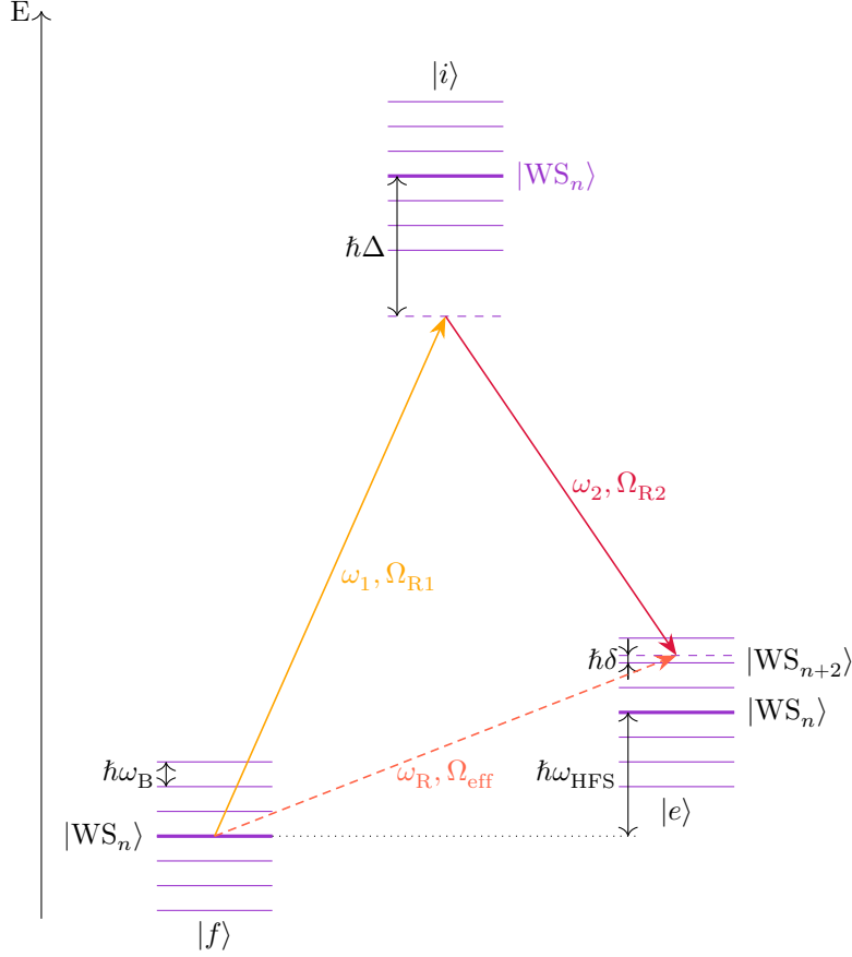
FIGURE II.5 – Processus de transition Raman à deux photons, pour un atome à trois niveaux piégé dans une échelle de Wannier-Stark. Si \Delta \gg \Omega_{1,2} et \omega_B \gg \Omega_{\text{eff}}, \delta , ce système est équivalent à un système à deux niveaux |f, \text{WS}_n\rangle et |e, \text{WS}_{n+\Delta m}\rangle , couplés par une transition de pulsation \omega_R = \omega_1 - \omega_2 et de pulsation de Rabi effective \Omega_{\Delta m} = \Omega_1^* \Omega_2 / 2\Delta \langle \text{WS}_m | e^{ik_{\text{eff}}z} | \text{WS}_{m+\Delta m} \rangle .
