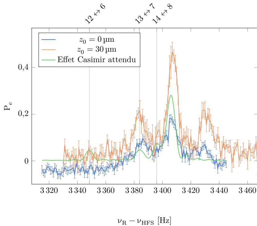
FIGURE V.20 – Spectroscopie Raman de la transition \Delta m = -6 au contact du miroir, comparée à celle pour des atomes à 30 \mu\text{m} de distance du miroir. Le spectre attendu compte tenu des différentes transitions possibles, perturbées par les interactions de Casimir-Polder (sec. II.3.1), est représenté en vert. Les fréquences de résonance de quelques transitions m \leftrightarrow m + \Delta m sont indiquées. Mesures effectuées pour \tau_\pi = 130 \text{ ms} .
