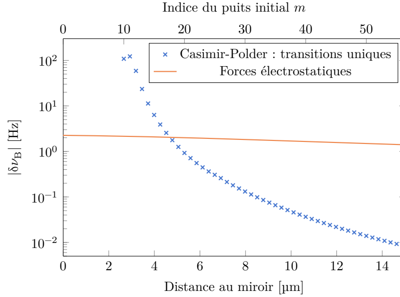
FIGURE V.19 – Décalage de la fréquence de Bloch attendu sous l’effet des interactions de Casimir-Polder pour des transitions entre puits uniques et sous l’effet des forces électrostatiques parasites (modélisées à la section précédente), pour une transition \Delta m = -6 .
