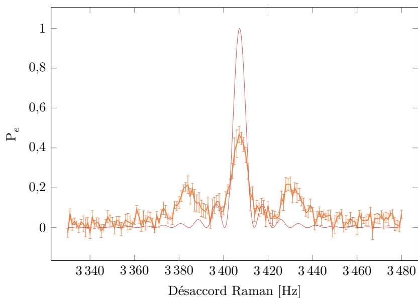
FIGURE III.11 – Spectroscopie Raman de la transition \Delta m = -6 à 30 \mu\text{m} de distance du miroir. Les bandes latérales sont visibles à \pm 23 \text{ Hz} autour du pic central, ce qui correspond à peu près à la fréquence attendue du piège de 20 \text{ Hz} . En rouge est représentée la probabilité de transition attendue pour une impulsion \pi parfaite.
