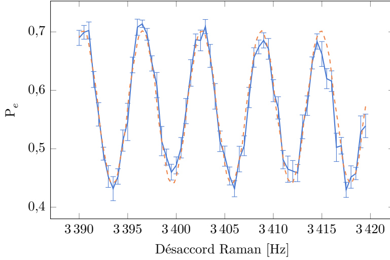
FIGURE IV.9 – Franges interférométriques typiques obtenues sur une transition \Delta m = -6 pour un temps d'interrogation T = 150 ms, et l'ajustement sinusoïdal correspondant en pointillés.
