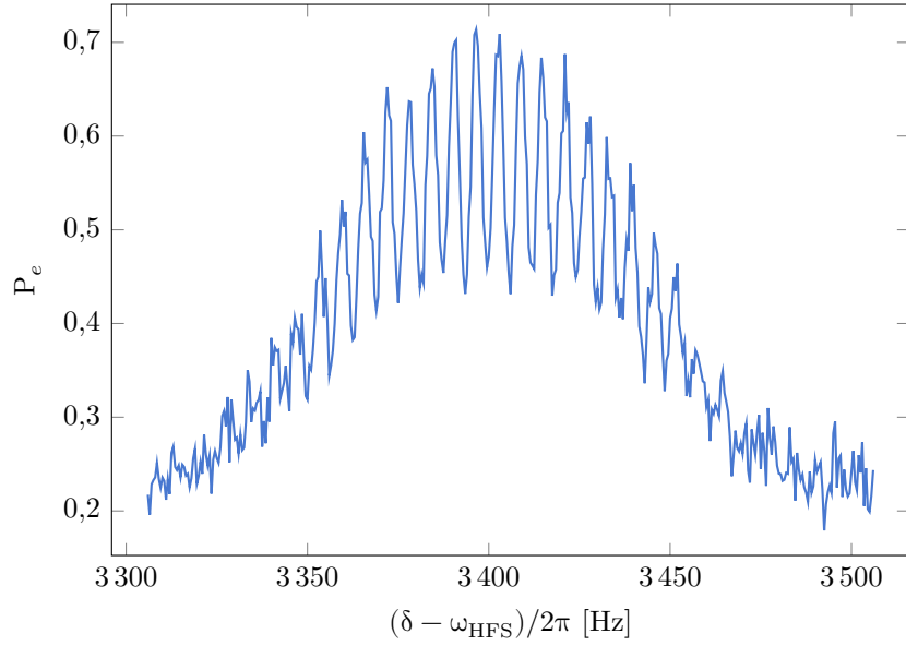
FIGURE II.11 – Franges de Ramsey expérimentales, pour la transition \Delta m = -6 . L'amortissement du contraste des franges à C \approx 0,3 est dû aux inhomogénéités de force et de déplacement lumineux différentiel (sec. IV.1). T = 150 ms et \tau_\pi = 22 ms.
