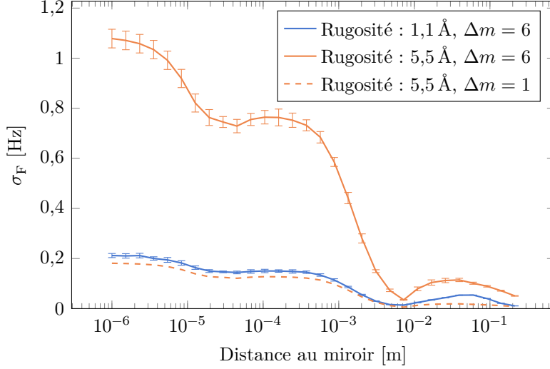
FIGURE IV.8 – Simulation des inhomogénéités de force dues aux tavelures créées par la rugosité de surface du miroir trichroïque. Le calcul a été effectué pour une moyenne quadratique de rugosité de 1,1 \text{ \AA} , correspondant à la rugosité mesurée dans [Str15], ou de 5,5 \text{ \AA} , et des distances de transitions entre deux puits \Delta m = 1 ou 6 . Paramètres de simulation : grille de 1860 \times 1860 \text{ \mu m} avec un pas de 1 \text{ \mu m} , waist incident de 190 \text{ \mu m} au niveau du miroir avec une puissance de 0,5 \text{ W} , moyenne de 10 simulations de rugosité.
