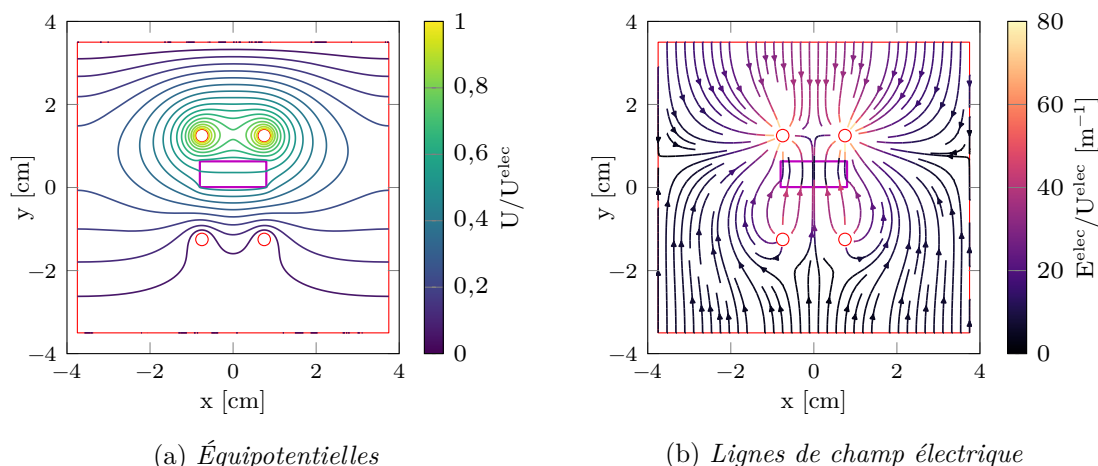
FIGURE VI.11 – Équipotentiels et lignes de champ électrique simulés par une méthode d'éléments finis. Les quatre électrodes et l'enceinte en vide (en rouge) servent de référence de potentiel. Ici, nous sommes dans une configuration de champ vertical, avec les deux électrodes supérieures polarisées à U^{\text{elec}} et les deux autres électrodes ainsi que l'enceinte à la masse. Le miroir et son support sont modélisés par une zone (en magenta) de permittivité diélectrique relative \varepsilon_r = 5 .
