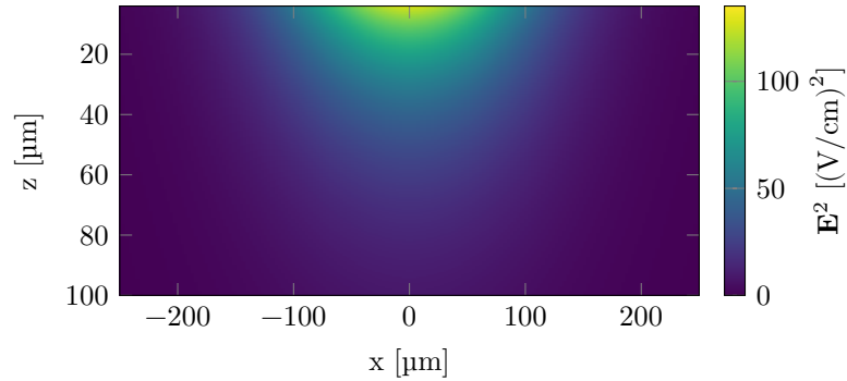
FIGURE V.15 – Norme quadratique du champ électrique produit par une distribution gaussienne de N moments dipolaires répartis à la surface du miroir sur une taille \sigma_\mu . Calcul effectué pour N\mu = 10^9 \times 3,2 \text{ D} et \sigma_\mu = 100 \mu\text{m} .
