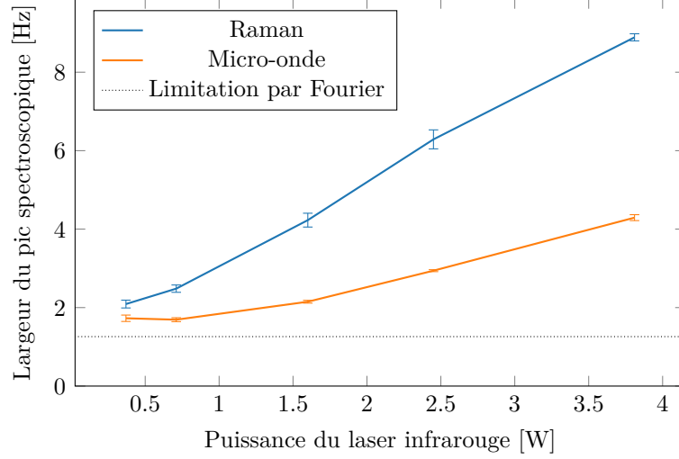
FIGURE IV.5 – Élargissement des pics spectroscopiques en augmentant la puissance IR, pour de la spectroscopie Raman sur une transition \Delta m = -6 et micro-onde sur la transition hyperfine. La largeur a été obtenue par l'ajustement d'une gaussienne sur les données de spectroscopie. La ligne pointillée correspond à la largeur attendue en cas d'une transition parfaite, issue de l'ajustement d'une gaussienne sur le sinus cardinal pour une impulsion \pi d'une durée de 495 ms.
