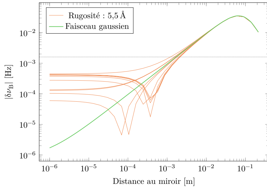
FIGURE V.8 – Simulation de la valeur absolue de la force moyenne générée par la diffusion d'un faisceau gaussien par une rugosité de surface du miroir de moyenne quadratique 5,5 Å. Chaque ligne orange représente la force dipolaire moyenne calculée pour un tirage aléatoire donné de profil de rugosité (en conservant toujours la même densité spectrale de bruit de rugosité). En vert est représentée la force dipolaire créée par la forme d'un faisceau gaussien idéal. La ligne en pointillés représente la meilleure sensibilité atteinte de l'expérience. Les paramètres de simulation sont les mêmes que pour la figure IV.8, avec waist incident de 190 \mu\text{m} au niveau du miroir et une puissance de 0,5 W.
