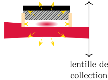
FIGURE III.13 – Illustration de l'ombre portée par le support du miroir (en beige) qui empêche d'imager les atomes au voisinage immédiat du miroir en bloquant la lumière d'imagerie rasante (en rouge). Nous pouvons vérifier la présence d'atomes dans cette ombre en collectant de la lumière diffusée par fluorescence (en jaune) lors de la détection par fluorescence.
