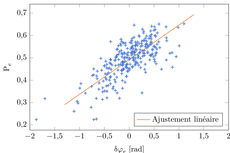
FIGURE IV.20 – Corrélations entre la probabilité de transition mesurée à mi-frange pour un interféromètre de 100 ms et l'estimation de la phase Raman due aux vibrations du miroir. L'ajustement linéaire en orange permet de déterminer le facteur de proportionnalité entre les deux, ici de 0,13.
