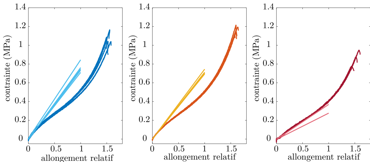
FIGURE 4.29 – Affichage de la relation entre contrainte dans l'éprouvette et allongement relatif pour les éprouvettes imprimée selon \vec{x} (gauche), \vec{y} (centre) et \vec{z} (droite). Pour chaque essai est représentée, dans une couleur plus claire, la droite de régression obtenue entre 0 et 0.1 d'allongement relatif.
