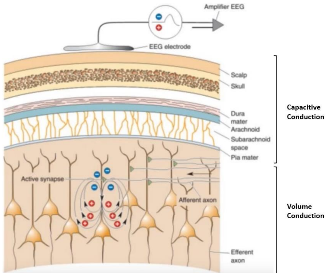
Figure 9 Schéma d'enregistrement des rythmes cérébraux : du neurone à l'électrode. Adapté de Mike X Cohen from zero to hero
