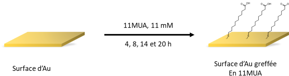
Figure VI. 4: Processus de greffage des surfaces d'Or en 11MUA.
