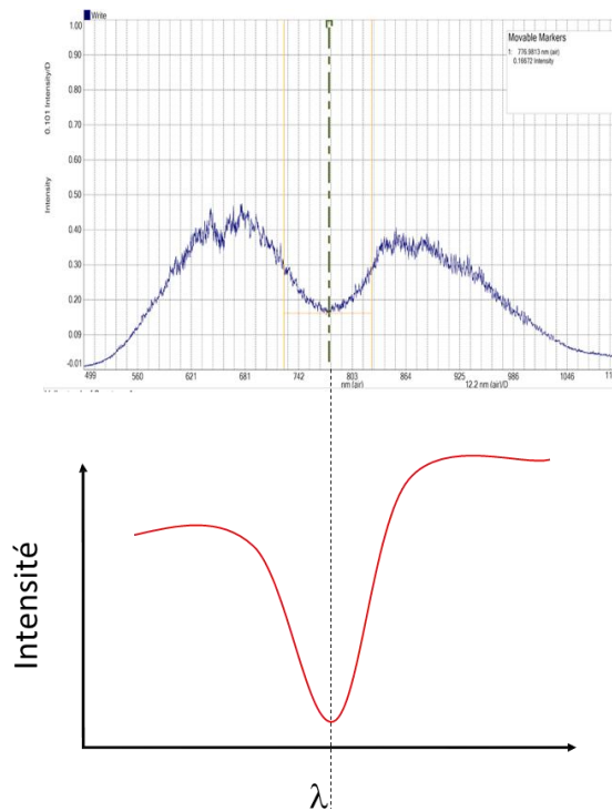
Figure III. 4 : Réponse SPR en interrogation spectrale expérimentale: spectrogramme (haut) et schématique (bas).
