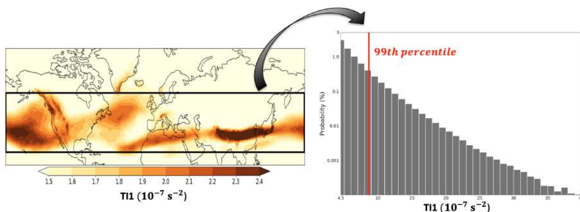
Figure 2.11 – Distribution spatiale de la moyenne des valeurs journalières de l’indice TI1. PDF des valeurs journalières extrêmes dans les moyennes latitudes (20-60°N) de l’indice TI1 (échelle logarithmique). La ligne verticale rouge indique le 99e percentile (seuil pour la MOG-CAT). Données de la réanalyse ERA5 (saison DJF, 1981-2010).
