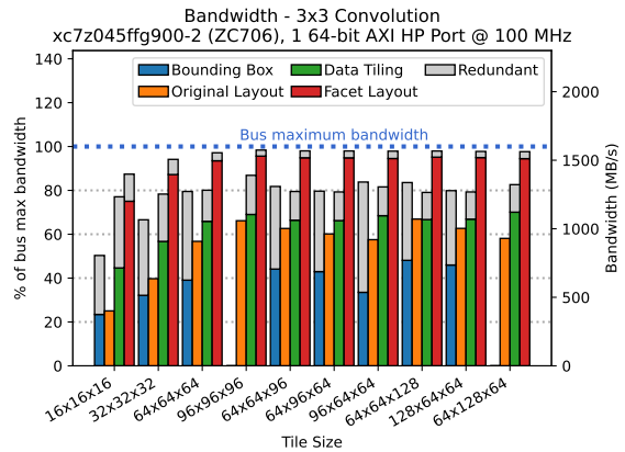
(d) jacobi2d9p
