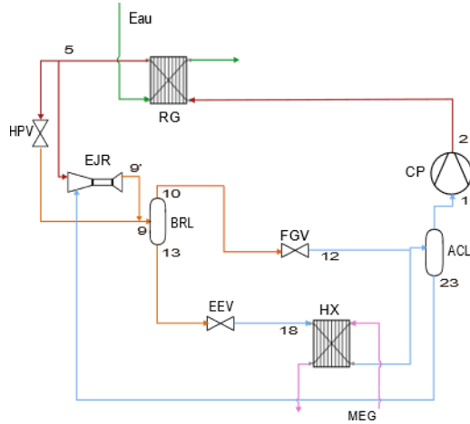
a) Schéma du système
