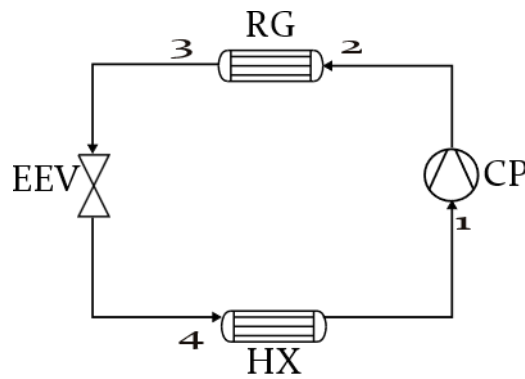
a) Schéma du système
