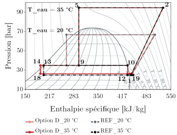
b) Option D représentée sur le diagramme de Mollier.
