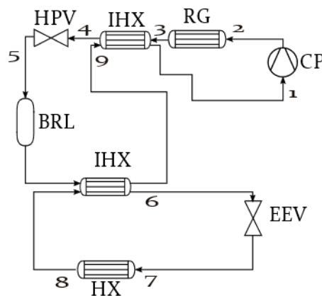
a) Schéma du système
