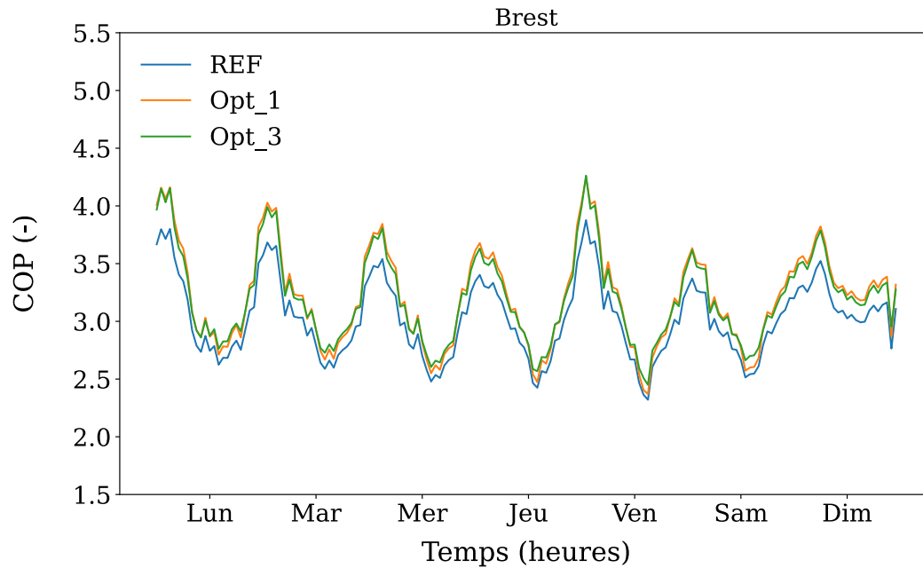
Figure 3.38. Performances calculées d'une installation frigorifique au \text{CO}_2 transcritique, pour la ville de Brest pour une semaine en été pour le système de référence et trois configurations différentes : avec économiseur (Opt_1), avec économiseur et compresseur parallèle (Opt_2), et avec sous-refroidisseur et économiseur (Opt_3).
