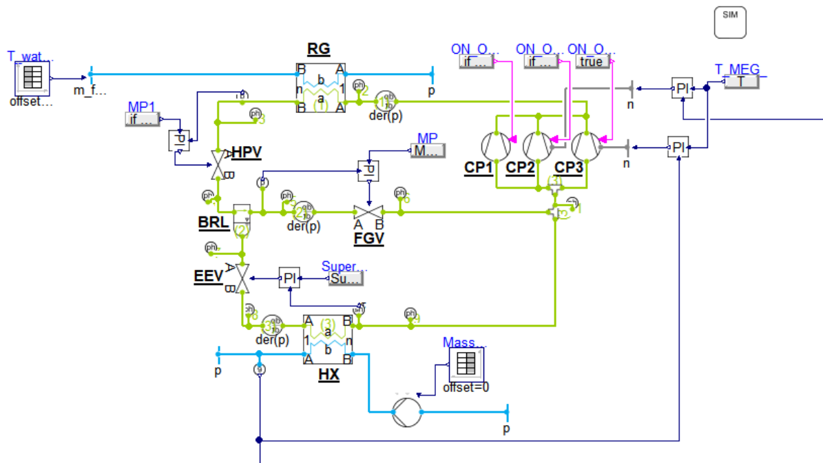
Figure 4.1. Modèle du système de référence sous Dymola en utilisant la bibliothèque TIL
