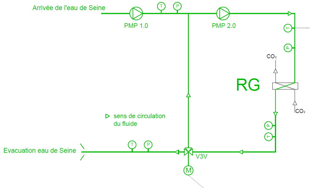
Figure A.1. Ancien schéma simplifié du circuit de réjection de chaleur
