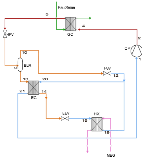
a) Schéma de l'option D
