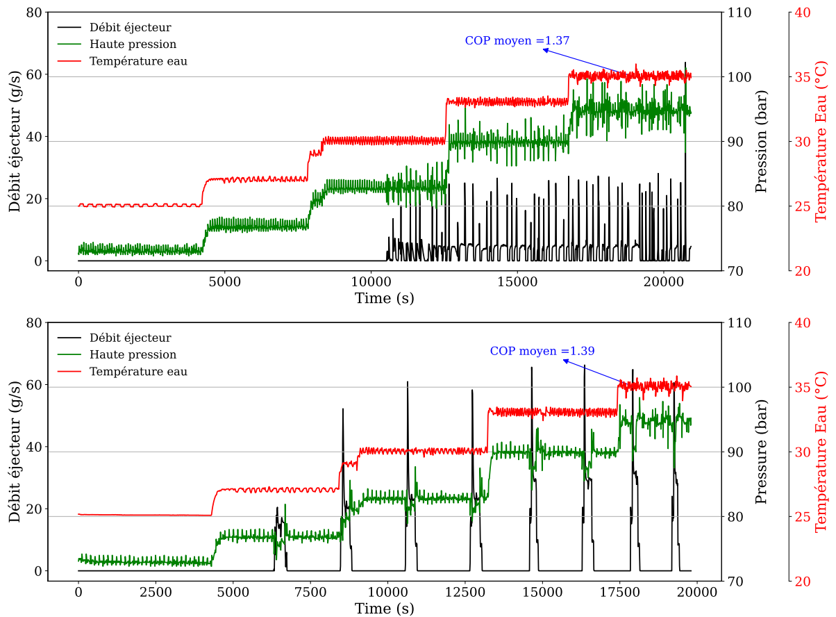
Figure A.3. Contrôle d'arrêt et de démarrage de l'éjecteur en régimes de transition et transcritique. En haut : mesures obtenues avec le contrôle fourni avec l'installation ; en bas : mesures obtenues après modification des paramètres de contrôle.
