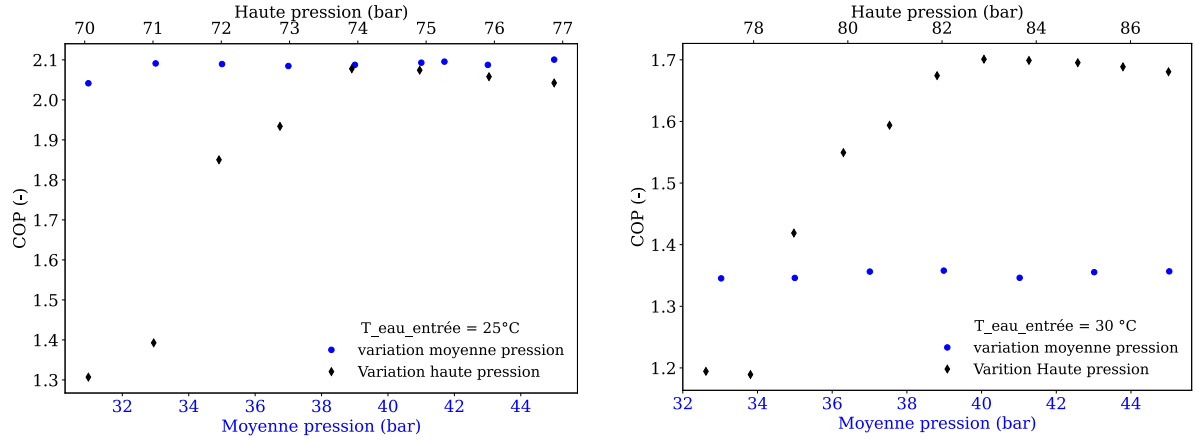
a) Impact de la haute et de la moyenne pressions sur le COP à 25 °C
