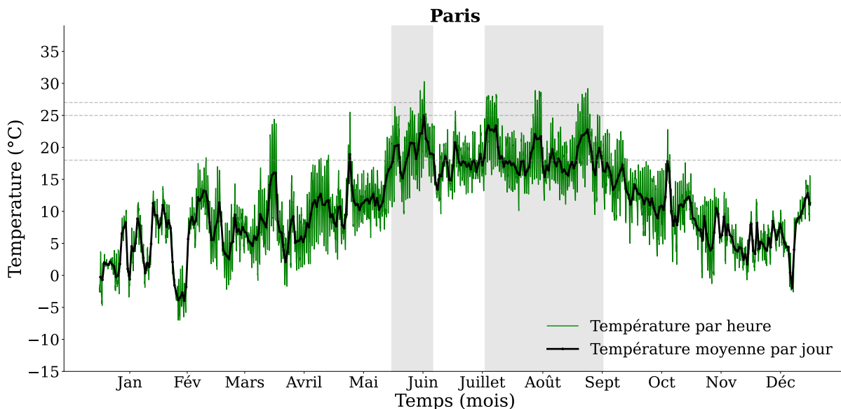
Figure 3.43. Températures extérieures à Paris en 2021. Les zones grises correspondent aux températures les plus élevées. Le début de la zone transition est marqué par la ligne pointillée grise
