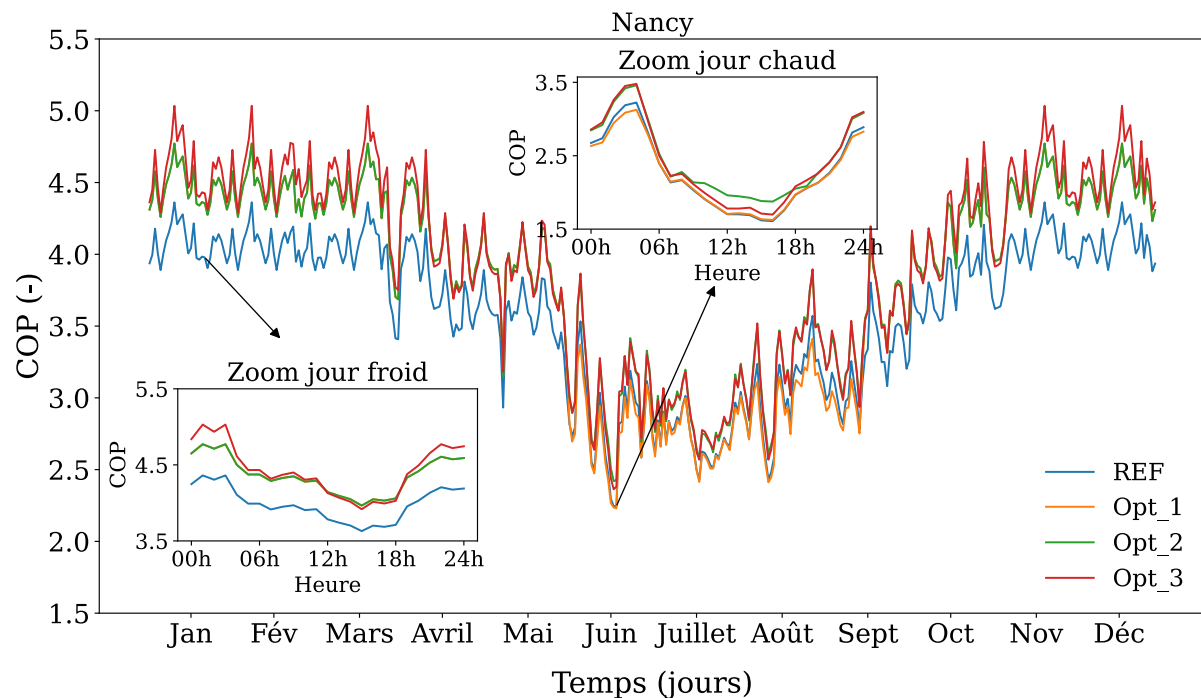
Figure 3.33. Coefficient de performance annuel pour la ville de Nancy pour le système de référence et trois configurations différentes : avec économiseur (Opt_1), avec économiseur et compresseur parallèle (Opt_2), et avec sous-refroidisseur et économiseur (Opt_3).
