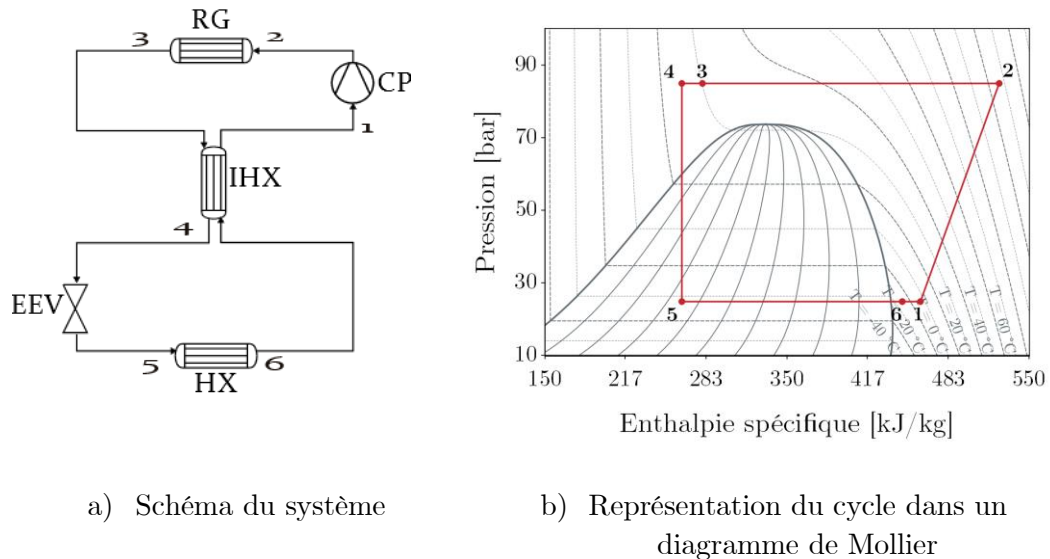
Figure 1.7. Système avec échangeur de chaleur interne
