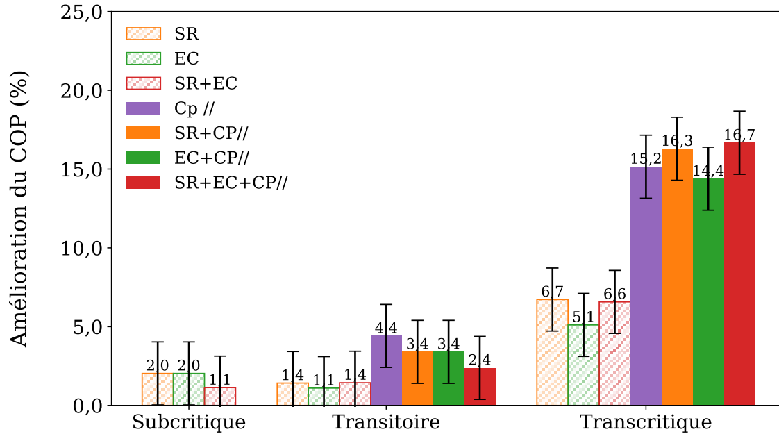
Figure 3.27. Comparaison de l'amélioration du COP avec les différentes configurations en utilisant la vanne flash gaz (barres hachées) et le compresseur parallèle (barres pleines), pour une surchauffe de 8 °C et une puissance frigorifique de 30 kW, par rapport au système de référence
