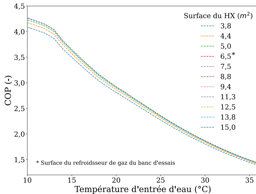
Figure 4.10. Influence de la surface de l'évaporateur sur le COP à différentes températures d'entrée d'eau pour le système de référence
