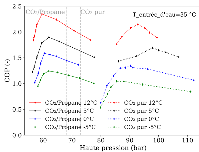
Figure 5.20. Coefficient de performance (COP) à température d'entrée d'eau de 35^\circ\text{C} et à températures d'entrée du fluide secondaire à l'évaporateur de 12^\circ\text{C} , 5^\circ\text{C} , 0^\circ\text{C} et -5^\circ\text{C} .
