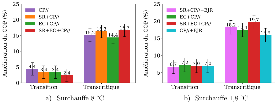
Figure 3.26. Amélioration du COP avec compresseur parallèle avec une puissance frigorifique de 30 kW
