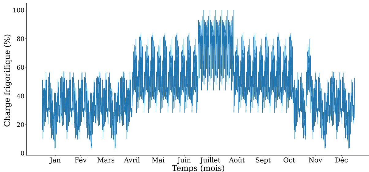
Figure 3.30. Représentation graphique de la charge frigorifique typique d'un supermarché en France
