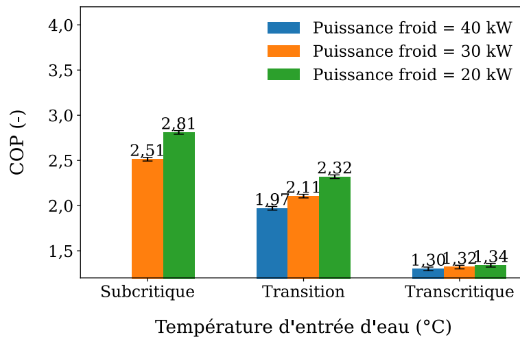
b) COP type pour chaque régime
