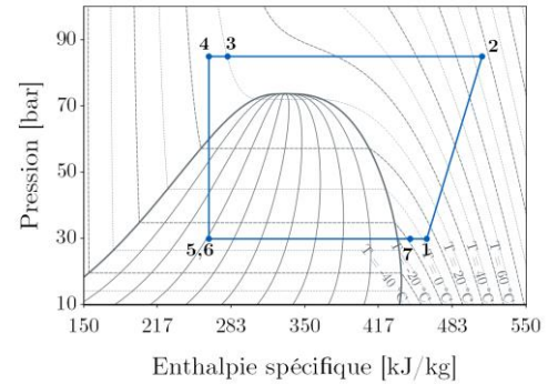
(b) Cycle représentée sur le diagramme de Mollier
