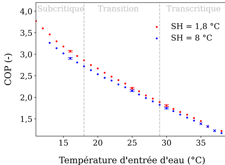
Figure 3.13. Coefficient de performance en fonction de la température d'entrée d'eau du refroidisseur de gaz pour deux surchauffes : 8 °C et 1,8 °C à une puissance frigorifique de 30 kW. Points = résultats sans oscillations. Croix = résultats avec oscillations.
