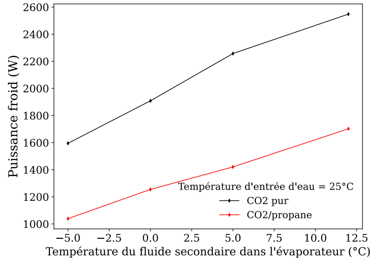
Figure 5.23. Puissance frigorifique à température d'entrée d'eau de 25 °C
