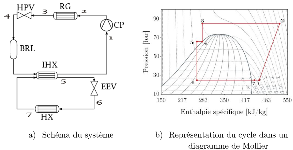
Figure 1.10. Autre configuration avec échangeur de chaleur interne
