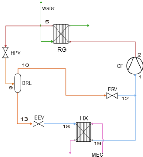
a) Schéma du système
