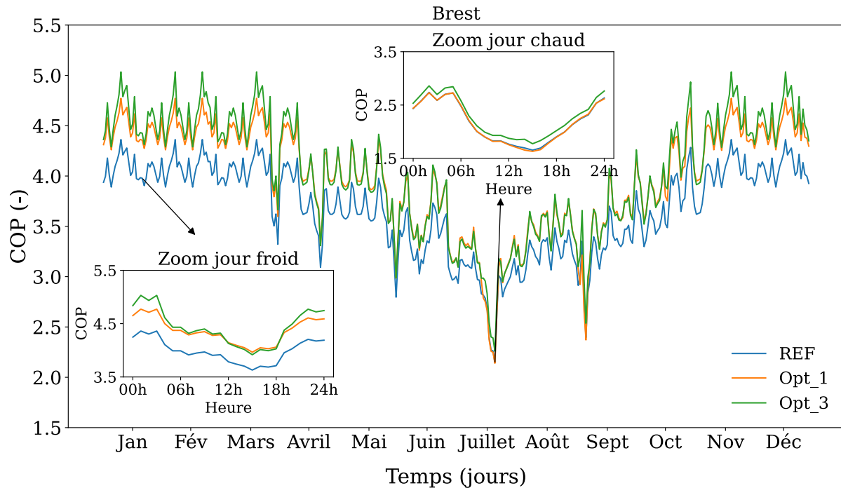
Figure 3.37. Coefficient de performance annuel pour la ville de Brest pour le système de référence et deux configurations différentes : avec économiseur (Opt_1), avec et avec sous-refroidisseur et économiseur (Opt_3).
