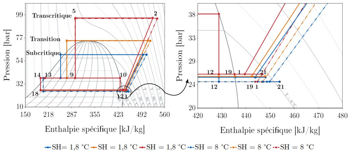
Figure 3.11. Cycle avec économiseur représenté sur le diagramme de Mollier (pression-enthalpie) pour trois régimes : subcritique (bleu), transition (orange) et transcritique (rouge).
