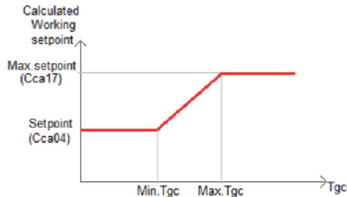
Figure B.5. Représentation graphique de la fonction d'optimisation de la moyenne pression pour le compresseur parallèle
