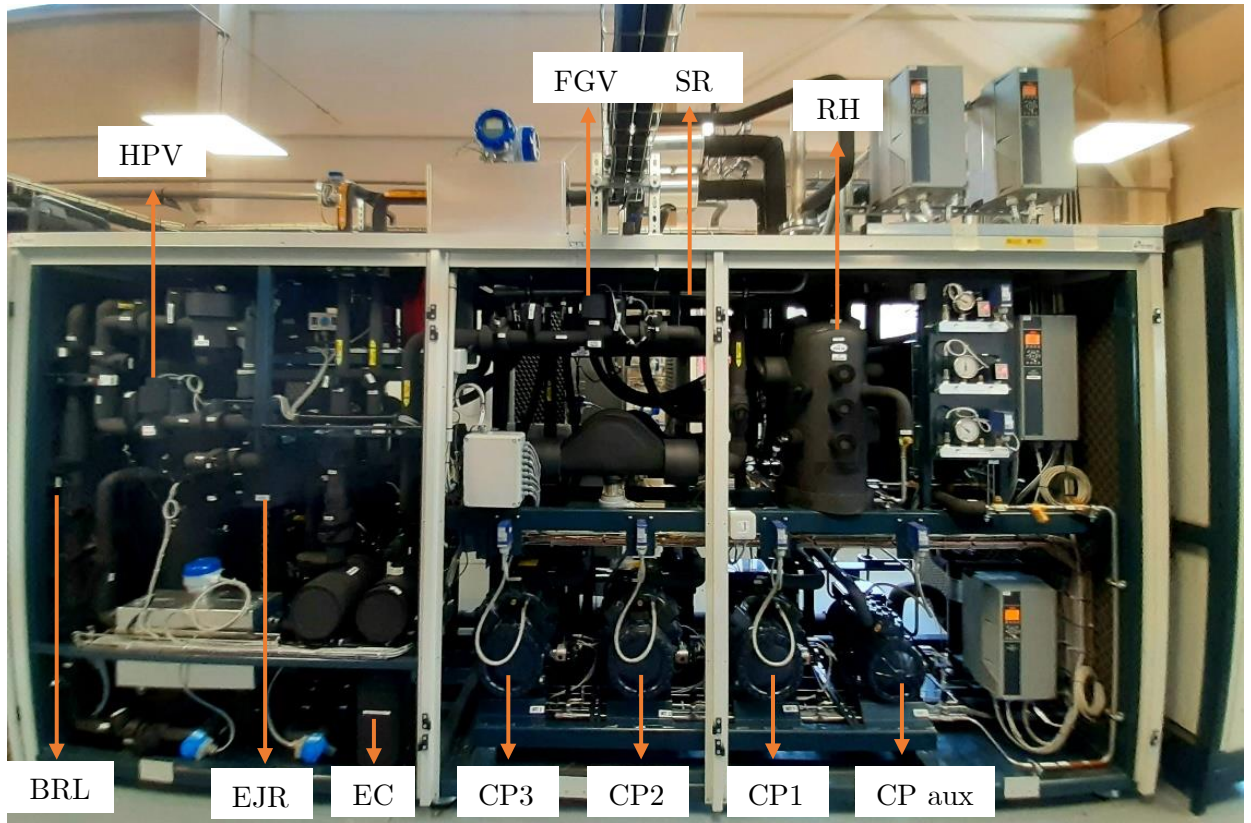
Figure 2.5. Groupe de production de froid au CO 2 (A)
