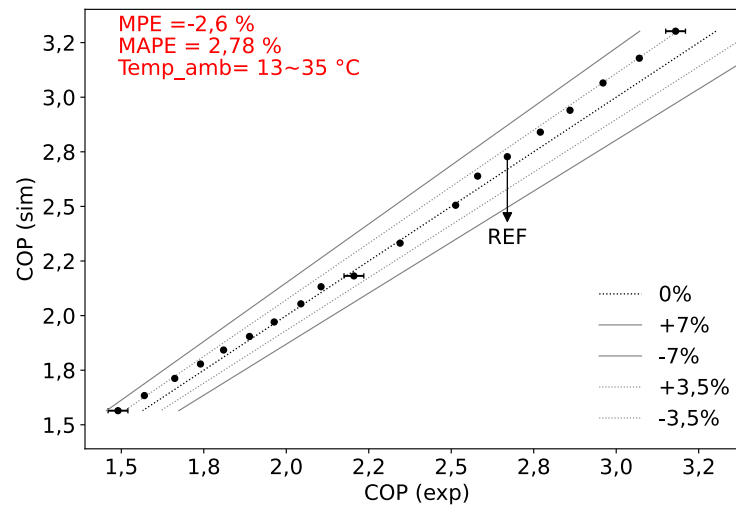
Figure 4.3. Coefficient de performance expérimental et simulé pour différentes températures d'entrée d'eau au refroidisseur de gaz, comprises entre 13 °C et 35 °C.
