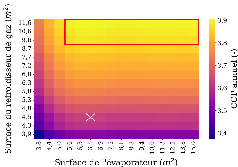
Figure 4.11. COP annuel en fonction de la surface du refroidisseur de gaz et de l'évaporateur. La croix représente les surfaces du banc d'essais du laboratoire. Le rectangle rouge présente la zone sans une variation significative du COP annuel.
