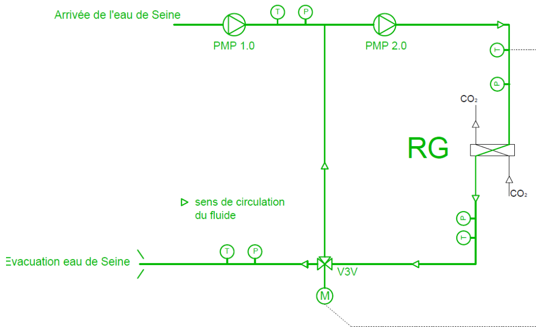
Figure 2.3. Schéma simplifié du réseau d'eau. T et P sont respectivement des capteurs de température et de pression. M représente une vanne motorisée. Le refroidisseur de gaz est représenté par RG.
