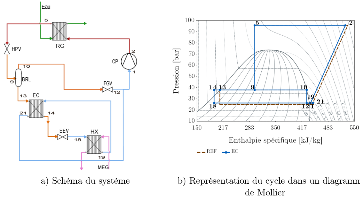
Figure 2.9. Système avec économiseur
