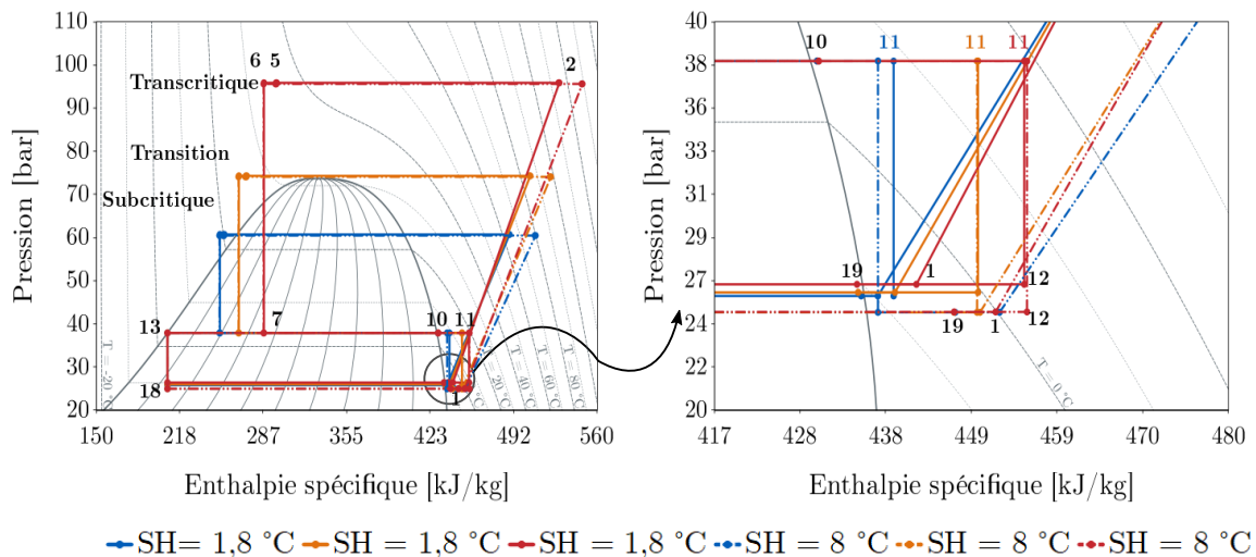
Figure 3.7. Cycle avec sous-refroidisseur représenté sur le diagramme de Mollier (pression-enthalpie) pour trois régimes : subcritique (bleu), transition (orange) et transcritique (rouge).
