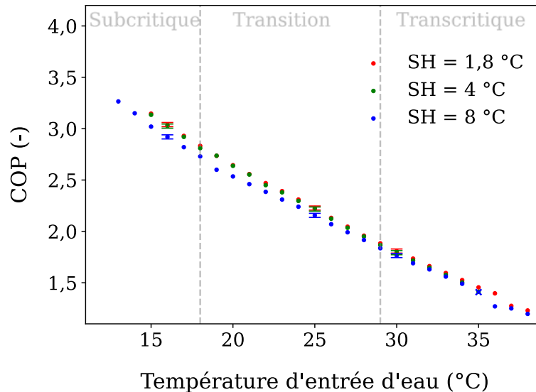
a) Comportement du COP à différentes températures d'entrée d'eau et pour différentes surchauffes. Points = résultats sans oscillations. Croix = résultats avec oscillations.
