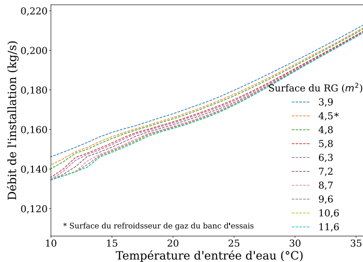
Figure 4.9. Débit de l'installation en fonction de la température d'entrée d'eau à différentes surfaces du refroidisseur de gaz
