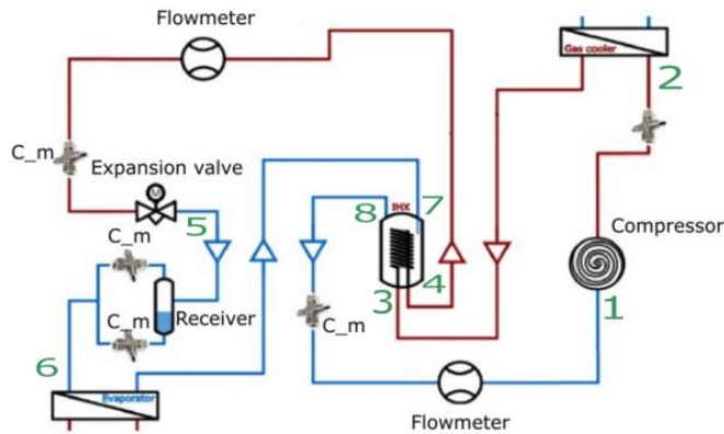
(a) Schéma du banc d'essais
