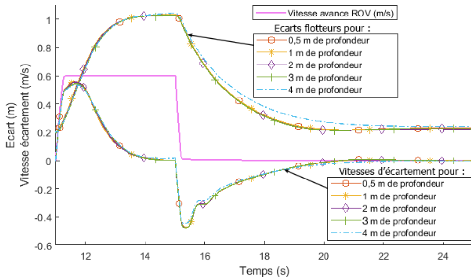
Figure III.22 – Écartement et vitesse d'écartement des flotteurs lorsque le ROV avance à une vitesse constante à différentes profondeurs
