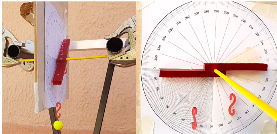
Figure B.2 – Photo de la mesure expérimentale de la raideur en torsion pour le câble Fathom Slim
