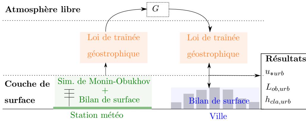
FIGURE 6.7 – Principe du prétraitement météorologique ( u_* : vitesse de friction, L_{ob} : longueur d’Obukhov, h_{cla} : hauteur de la CLA, G : vitesse géostrophique)
