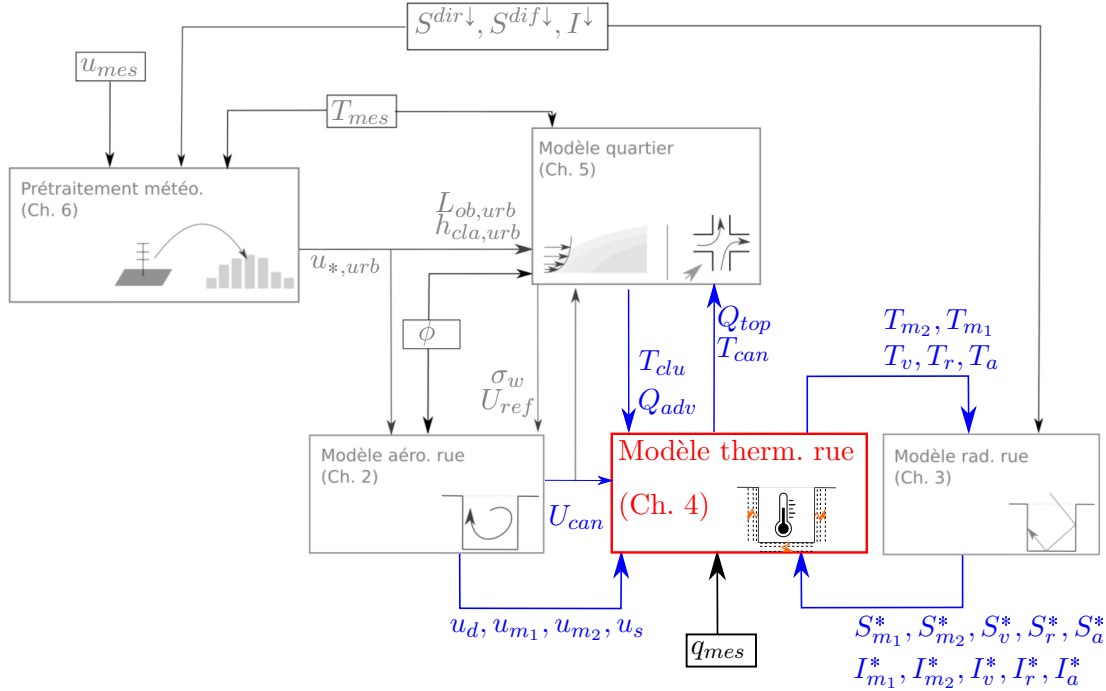
FIGURE 4.1 – Données d'entrée et résultats du modèle thermo-énergétique de rue ( U_{can} [m/s] : vitesse moyenne longitudinale ; u_d [m/s] : vitesse d'échange rue/clu ; u_{m_1} , u_{m_2} , u_s [m/s] : vitesses proche paroi ; S_i^* , I_i [ W/m^2 ] : densités de flux solaire et infrarouge nettes ; T_i [K] : températures ; Q_{top} , Q_{adv} [ W/m^2 ] : échanges de chaleur vertical et horizontal aux limites de la rue ; q_{mes} [kg/kg] : humidité absolue mesurée à la station météorologique).
