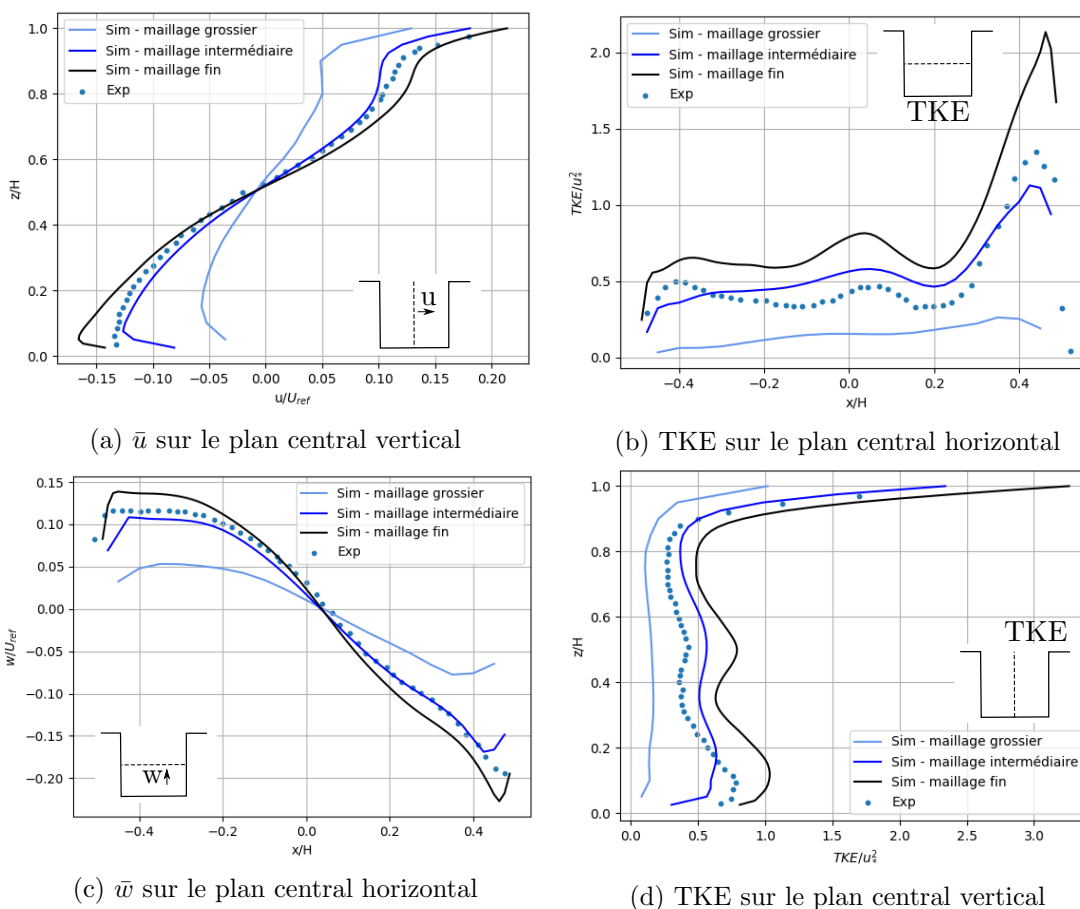
FIGURE 2.16 – Écoulement dans la rue dans la configuration A ( \bar{u} [m/s] : Vitesse moyenne selon x ; \bar{w} [m/s] : Vitesse moyenne selon z )
