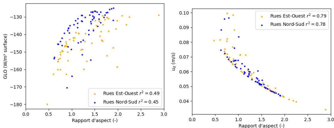
(a) Densité de flux infrarouge ramené aux surfaces urbaines (murs + route)
