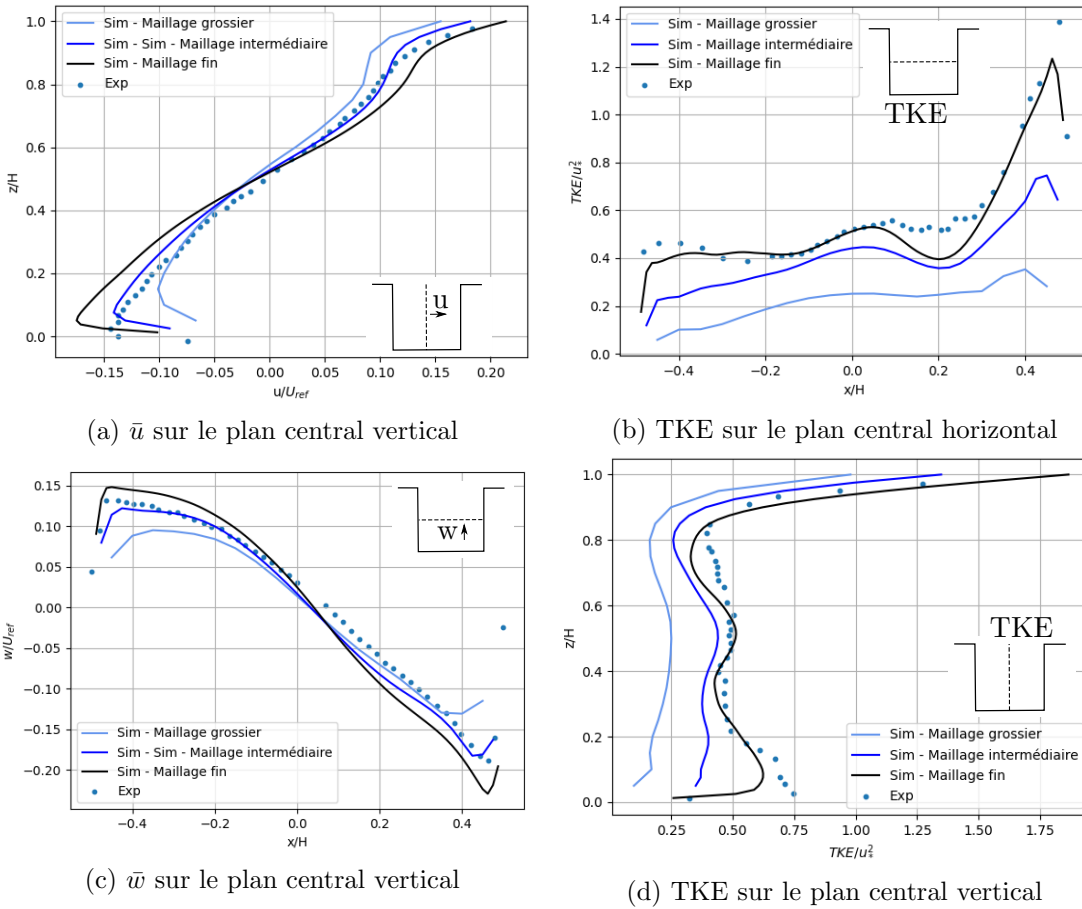
FIGURE 2.18 – Écoulement dans la rue dans la configuration D ( \bar{u} [m/s] : Vitesse moyenne selon x ; \bar{w} [m/s] : Vitesse moyenne selon z )
