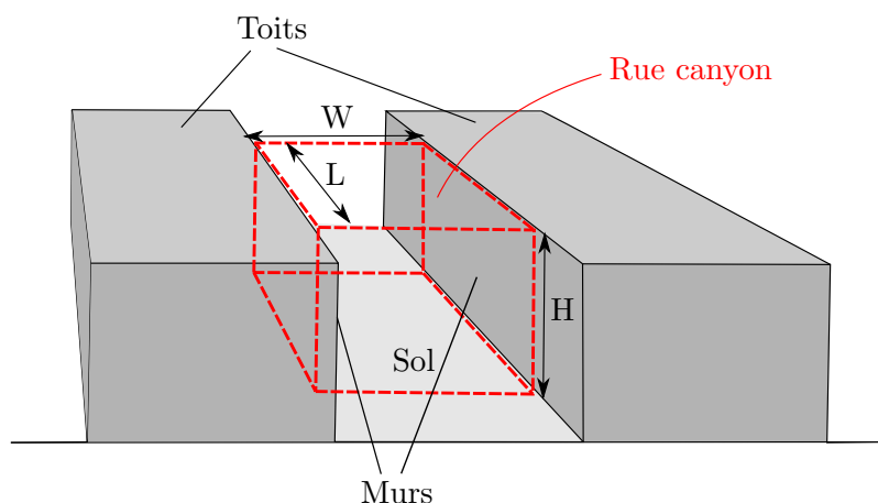
FIGURE 1.5 – Définition d'une rue canyon selon [Nunez & Oke 1977]
