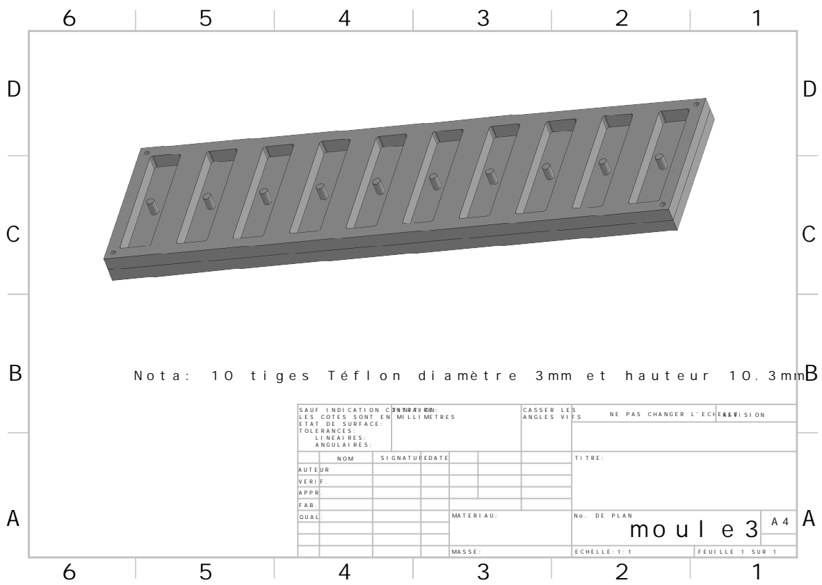
FIGURE A.1 – Moule échantillon DCDC - vue 3D.
