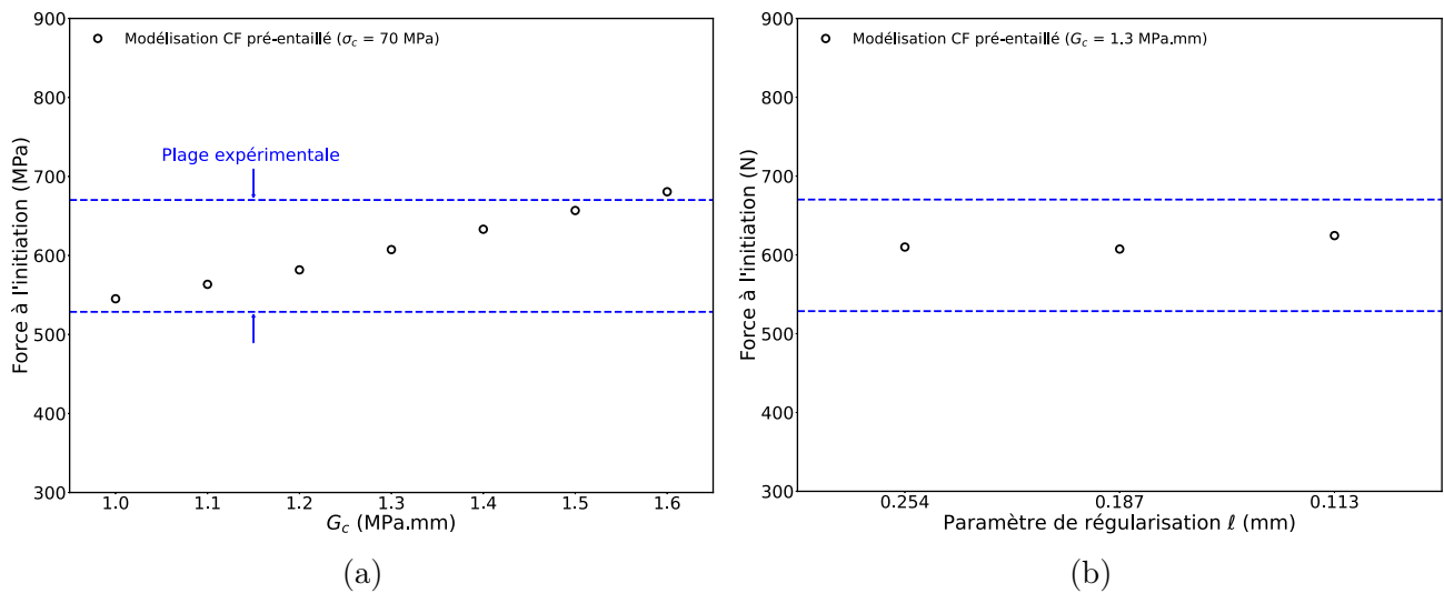
FIGURE 5.8 – Modélisation de l'essai SENB pré-entaillé sur PMMA par approche de champ de phase (a) Impact de la variation de G_c et (b) Impact de la variation de \ell , sur l'effort à l'initiation.
