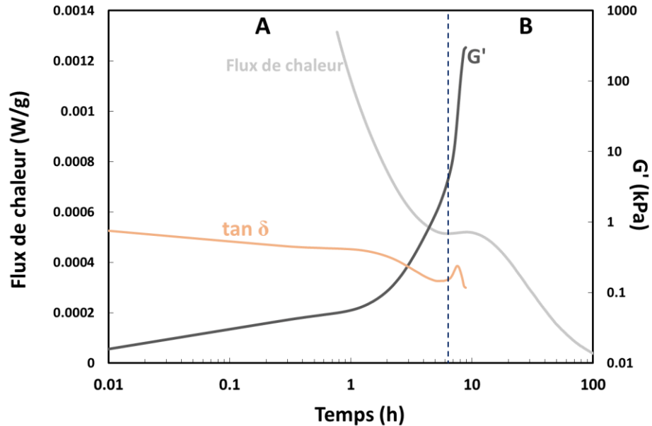
Figure III. 6 Evolution de G', tan δ et flux de chaleur du MK21 en fonction du temps
