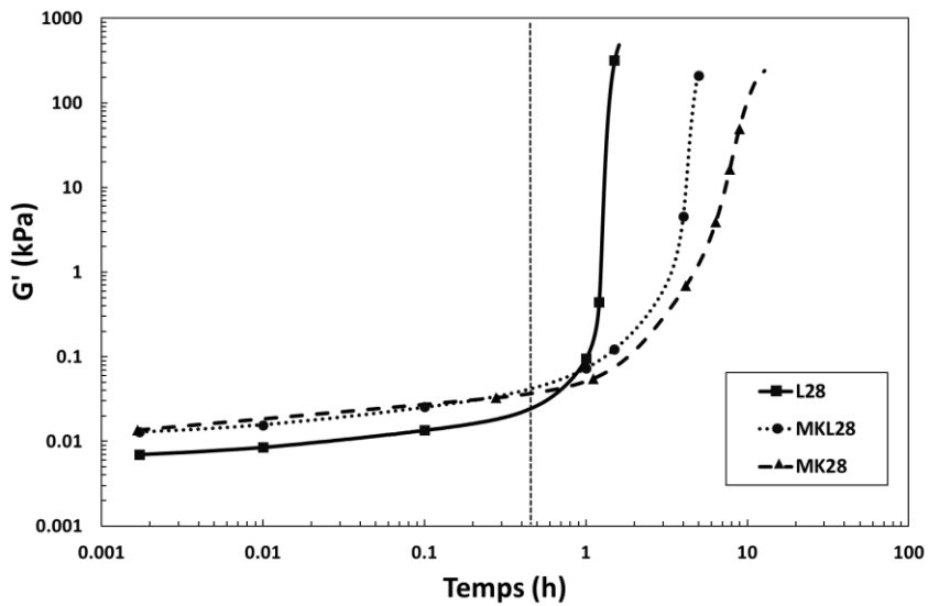
Figure IV. 2 Evolution du module G' en fonction du temps
