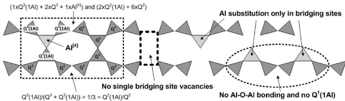
Figure I. 5 Illustration du modèle CSTM, incluant les hypothèses et contraintes prises en compte [6]
