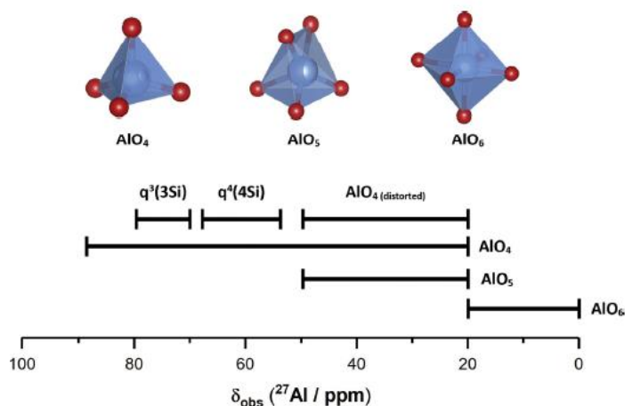
Figure II. 24 Gammes typiques de déplacements chimiques ^{27}\text{Al} pour différents sites d'aluminium. Les atomes de Al et O sont représentés par des sphères bleues et rouges respectivement [11], [118]
