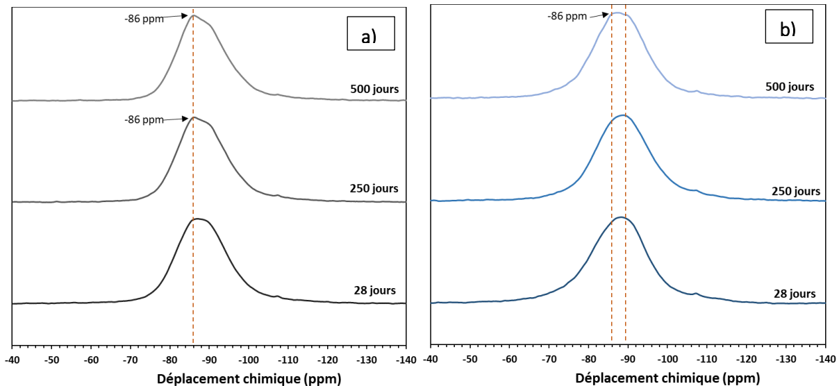
Figure IV. 23 Spectres ^{29}\text{Si} des coulis binaires MKL21 (a) et MKL34 (b) à 28, 90 et 250 jours
