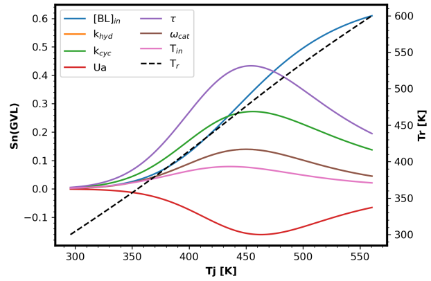
(d) GVL PSA for Ua=5000 \text{ W/m}^3/\text{K} .
