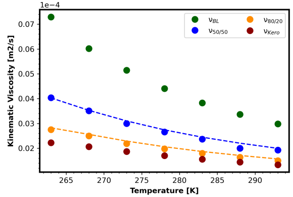
(d) Kinematic Viscosity vs Temperature.
