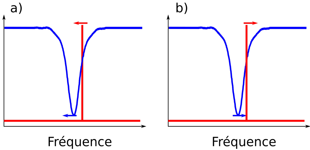
FIGURE 4.19 – Schéma explicatif d'un asservissement thermique. a) lorsque la fréquence du laser diminue la fréquence de résonance diminue également, b) lorsque la fréquence du laser augmente la fréquence de résonance augmente pour compenser la variation
