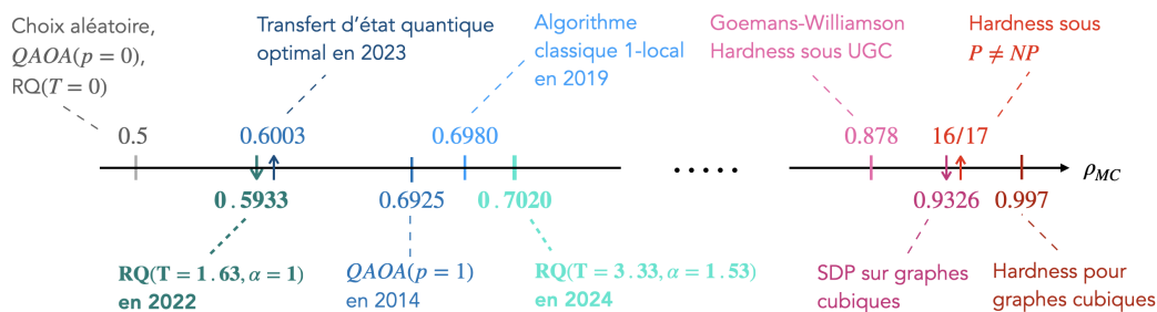
Figure 8: Ratio d’approximation atteint par différent algorithmes que nous détaillons par la suite. En gras sont indiquées nos contributions.
