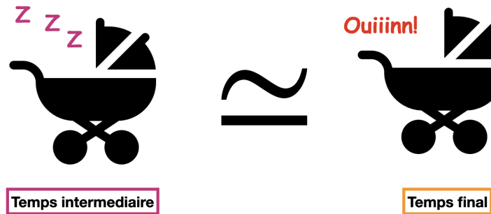
Figure 3: Le phénomène de localisation d’Anderson avec notre illustration. L’état d’énergie le plus bas à un moment intermédiaire est le bébé endormi au milieu du voyage. Ce dernier état est proche au bébé qui pleure à la fin du voyage. Ici le terme “proche” est légèrement tiré par les cheveux et montre une limite de notre analogie.
