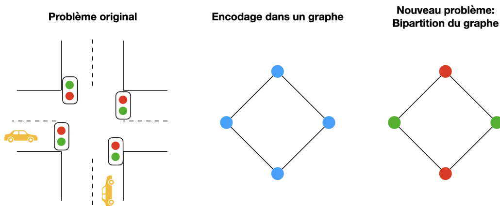
Figure 4: Illustration du problème de la coupe maximale. À gauche, le problème original. Au milieu, son encodage dans une instance de graphe. À droite, une solution possible au problème de la coupe maximale sur le graphe donné. Cette dernière solution est également une solution au problème original.
