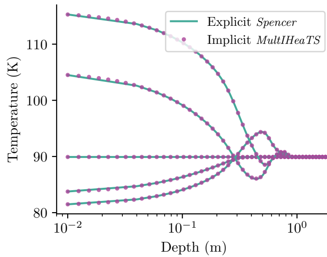
Figure 6.14: Validation de MultiIHeaTS par rapport à l'algorithme explicite de Spencer. Les profils de température pour différents moments sont tracés à i = 0, 200, 14050, 34959, 49000 . MultiIHeaTS est aussi précis que le solveur explicite de Spencer avec l'avantage de la stabilité. L'espaceur inégal de la grille de MultiIHeaTS, plus dense à la surface est montré par l'axe horizontal logarithmique.
