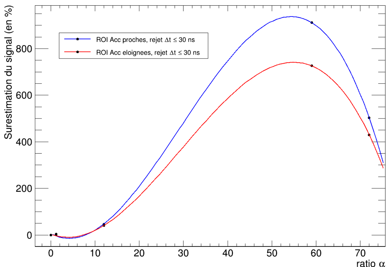
Figure 89. Surestimation du signal utile en fonction du ratio alpha, en présence des sources neutroniques seules ( ^{252}\text{Cf} ou ^{240}\text{Pu} + AmBe) pour la matrice organique.
