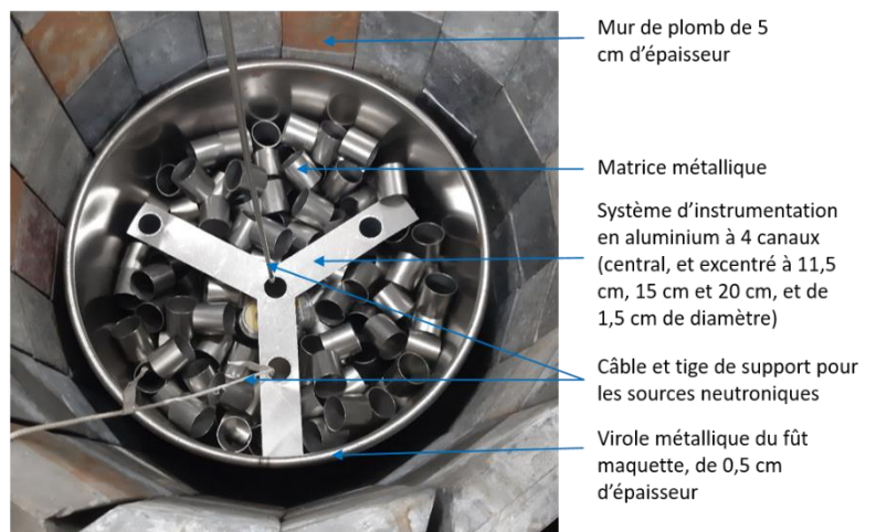
Figure 49. Dispositif de mesure maquette pour fûts de déchets radioactifs de 100 à 220 L.
