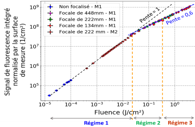
figure 114 : Evolution du signal de fluorescence en fonction de l'influence du laser dans trois zones distinctes.
