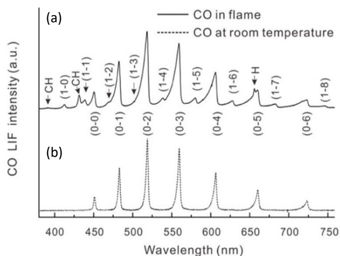
figure 18 : Spectre de fluorescence de CO en régime fs dans a) flamme laminaire prémélangée \text{CH}_4/\text{air} à une richesse 1,5 et b) mélange gazeux de \text{CO}/\text{N}_2 à température ambiante [94].
